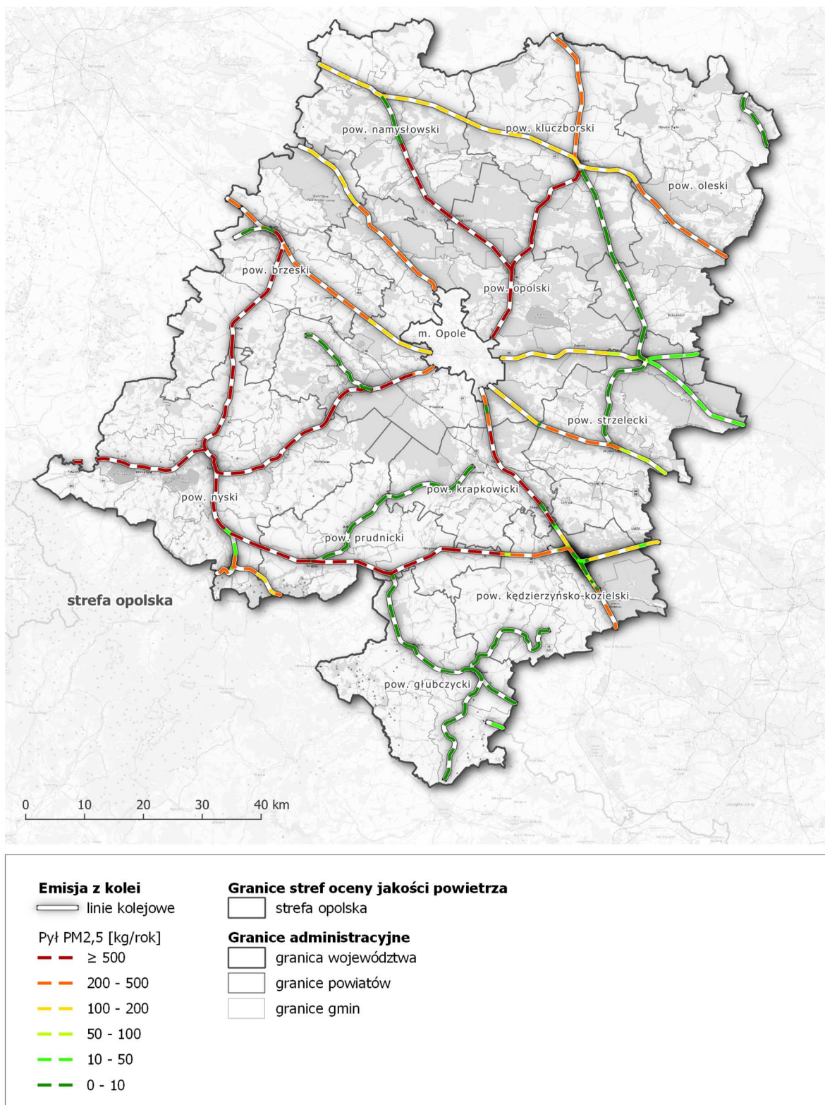
Rysunek 64. Lokalizacja i wielkość emisji pyłu PM 2,5 z kolei w strefie opolskiej w roku bazowym 2018 235
