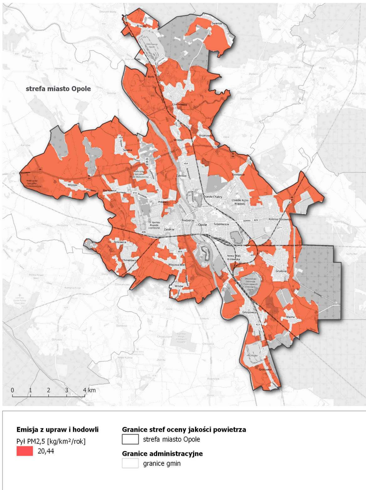
Rysunek 77. Lokalizacja i wielkość emisji pyłu PM 2,5 z upraw i hodowli w strefie miasto Opole w roku bazowym 2018 248
