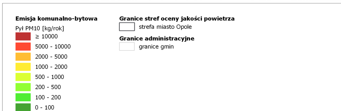
Rysunek 89. Lokalizacja i wielkość emisji pyłu PM10 ze źródeł z sektora komunalno-bytowego w strefie miasto Opole w roku bazowym 2018 260
