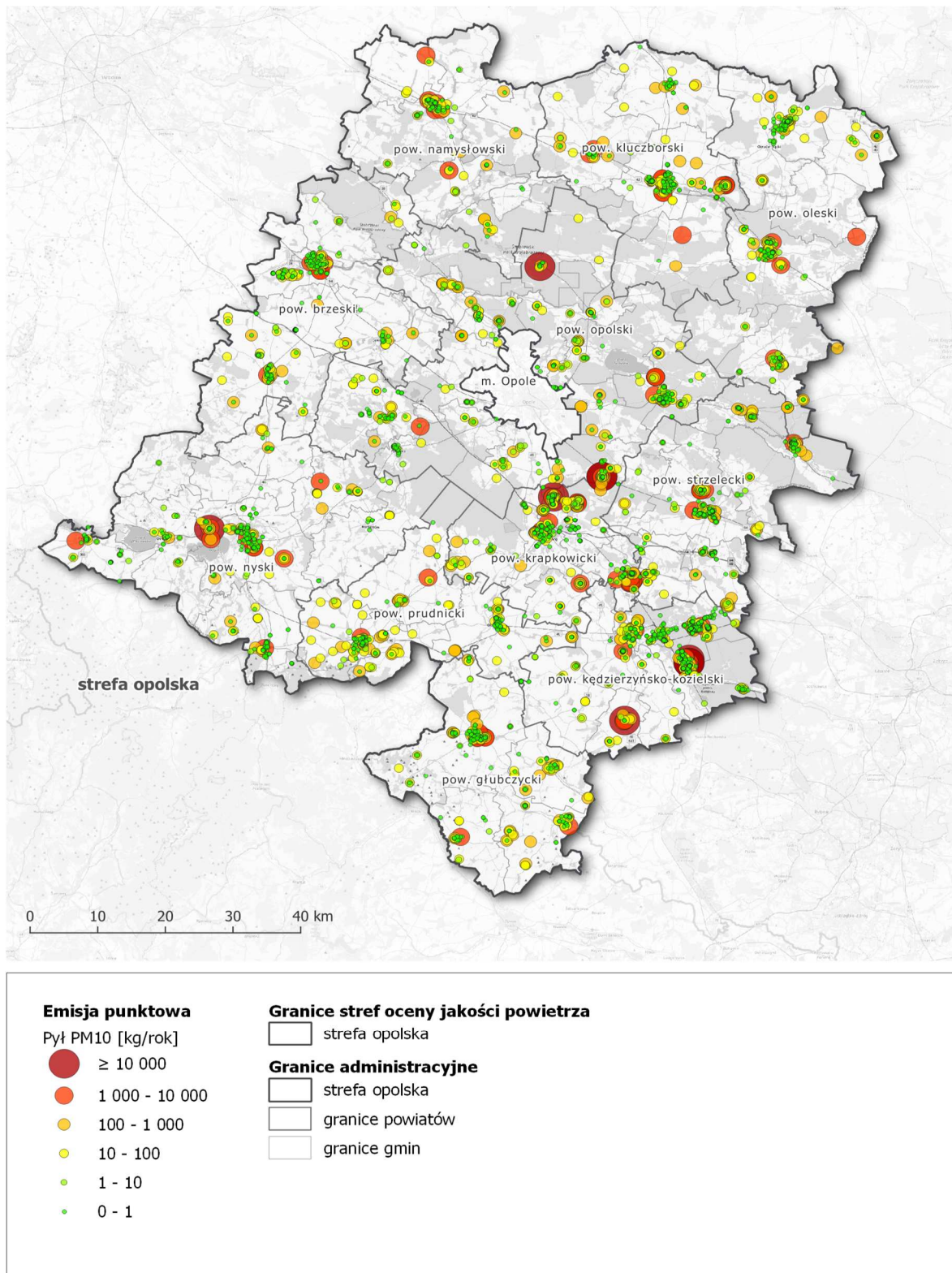
Rysunek 52. Lokalizacja i wielkość emisji pyłu PM10 z przemysłu i energetyki w strefie opolskiej w roku bazowym 2018 223
