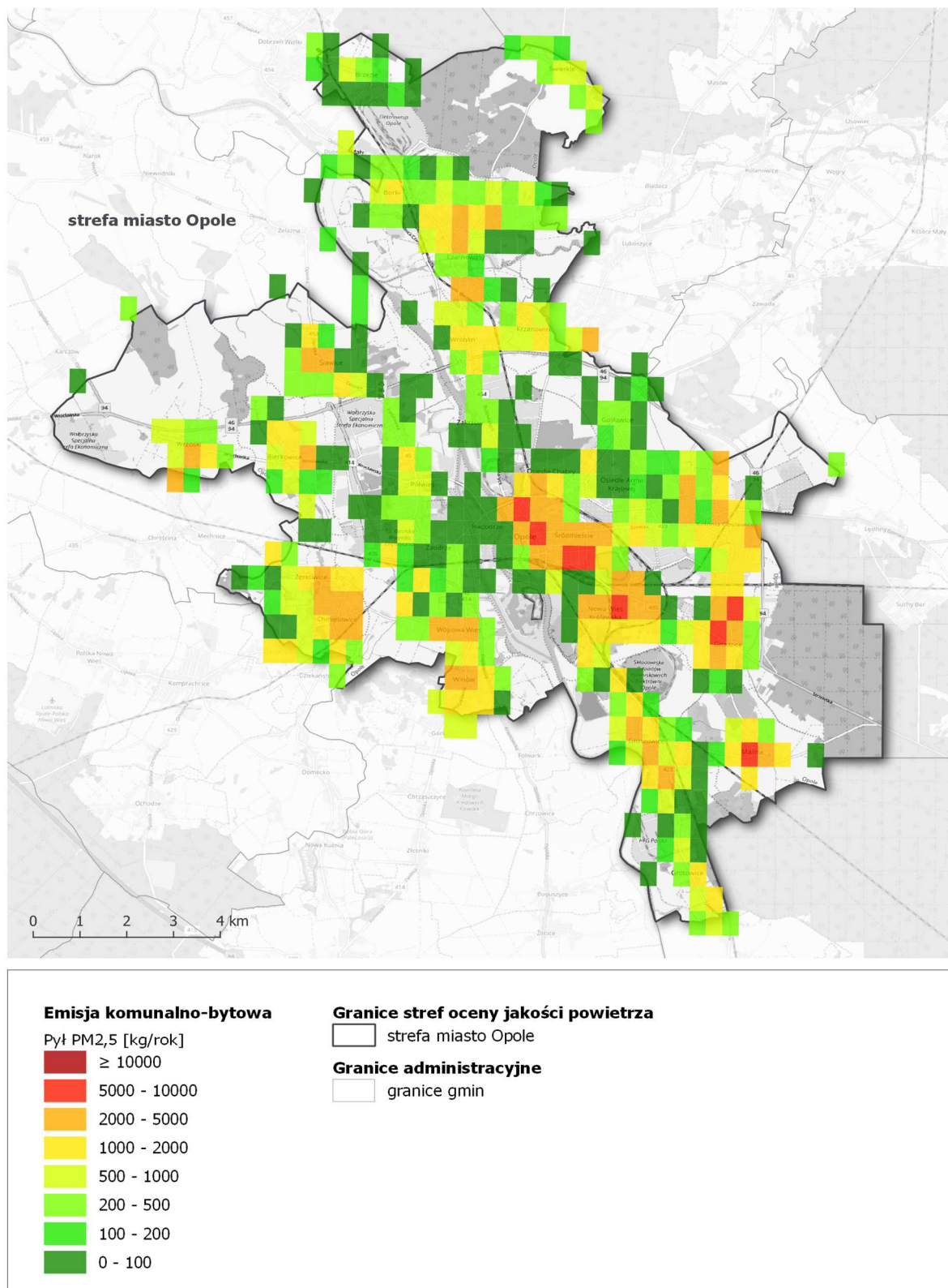
Rysunek 91. Lokalizacja i wielkość emisji pyłu PM 2,5 ze źródeł z sektora komunalno-bytowego w strefie miasto Opole w roku bazowym 2018 262
