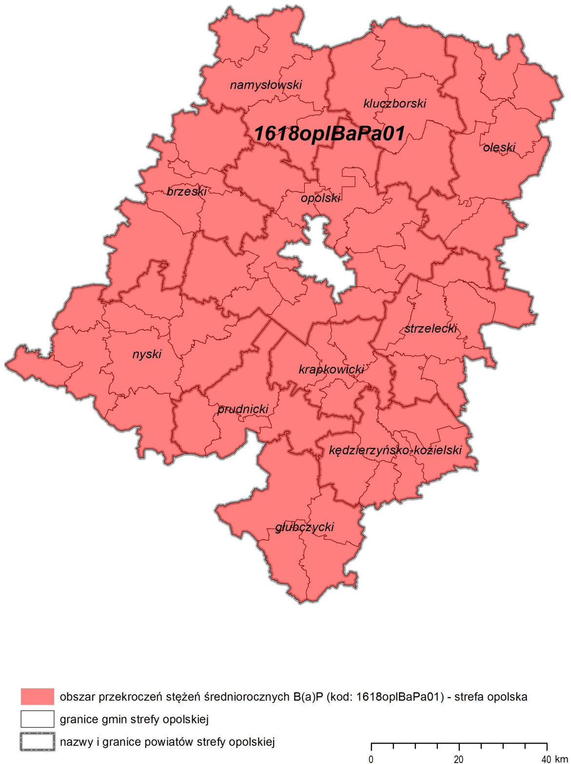
Rysunek 28. Obszar przekroczeń stężeń średniorocznych benzo(a)pirenu na terenie strefy opolskiej 100
