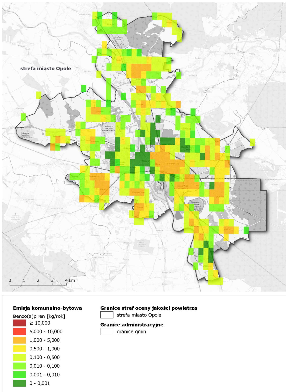
Rysunek 93. Lokalizacja i wielkość emisji benzo(a)pirenu ze źródeł z sektora komunalno-bytowego w strefie miasto Opole w roku bazowym 2018 264
