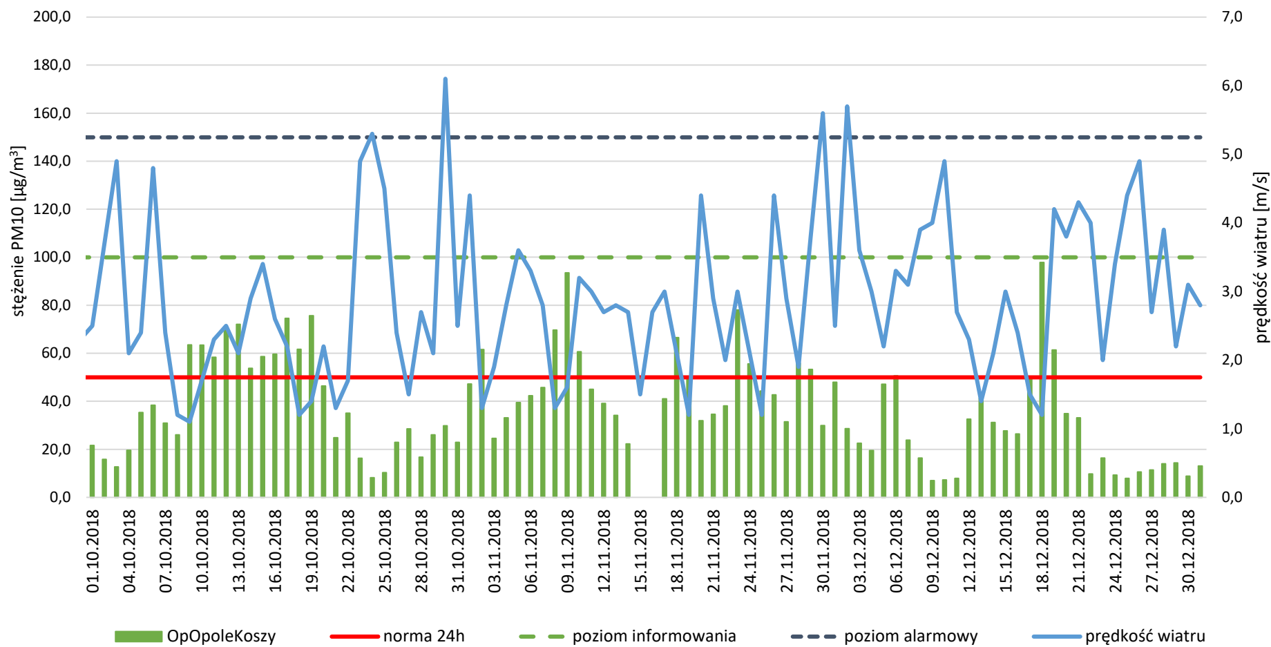
Rysunek 40. Porównanie przebiegu zmienności stężeń 24-godz. pyłu zawieszzonego PM10 w IV kwartale 2018 r. w Opolu z prędkością wiatru.
