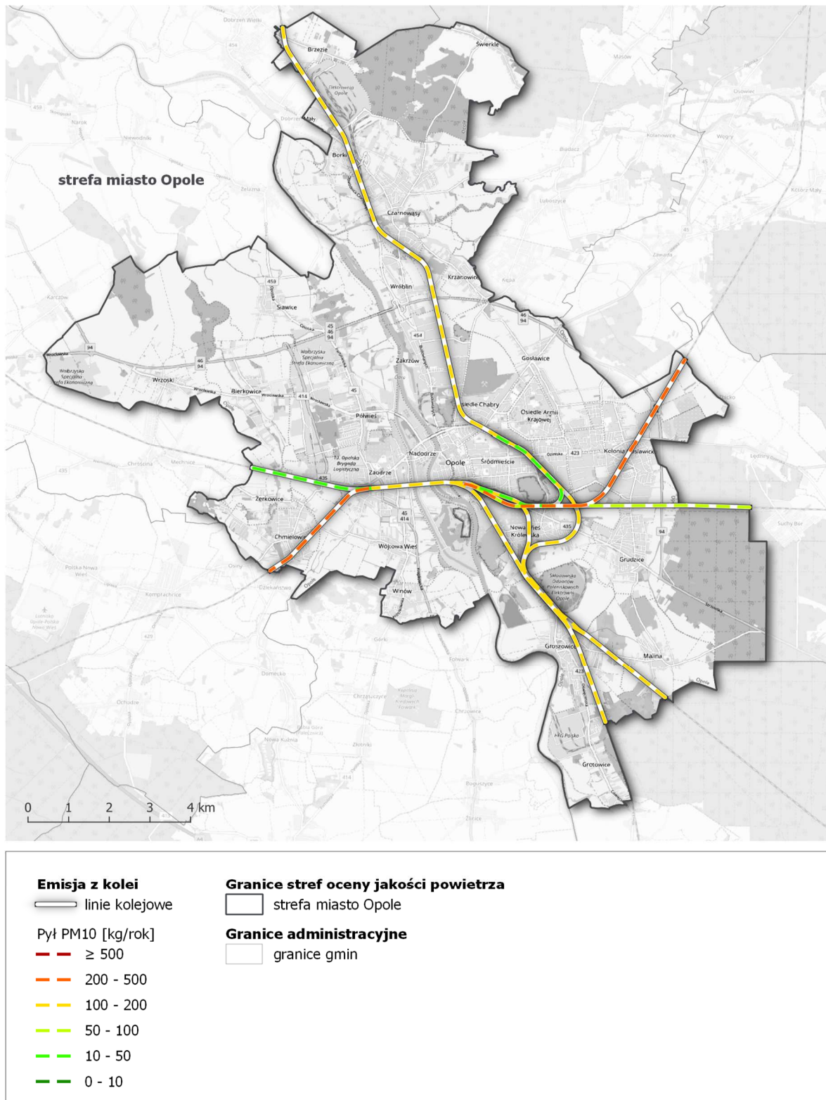
Rysunek 61. Lokalizacja i wielkość emisji pyłu PM10 z kolei w strefie miasto Opole w roku bazowym 2018 232
