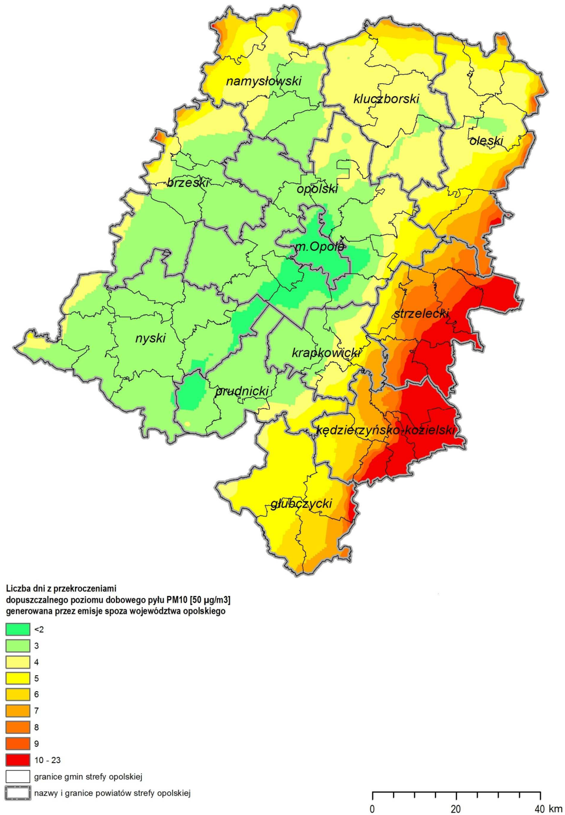
Rysunek 36. Liczba dni z przekroczeniem dopuszczalnego poziomu dobowego pyłu zawieszony PM10 generowana przez emisję spoza województwa opolskiego 120
