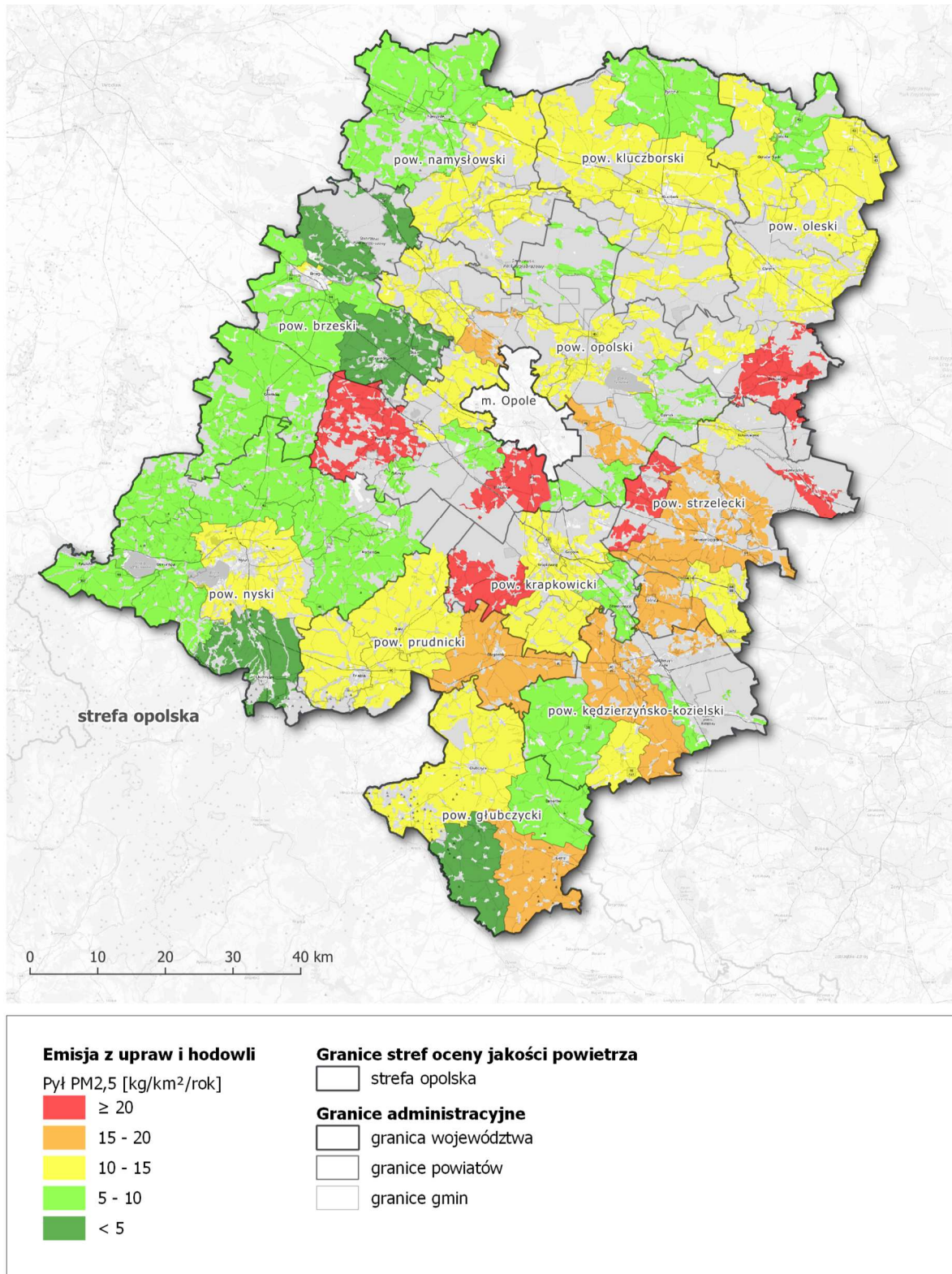
Rysunek 78. Lokalizacja i wielkość emisji pyłu PM 2,5 z upraw i hodowli w strefie opolskiej w roku bazowym 2018 249
