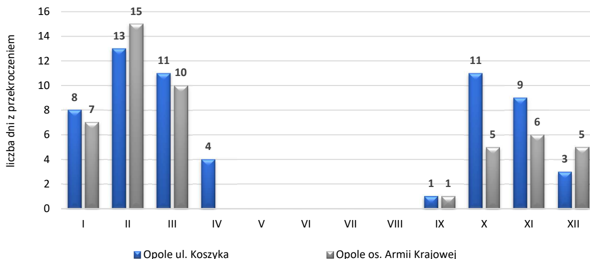
Rysunek 12. Liczba dni w poszczególnych miesiącach z przekroczeniem poziomu dopuszczalnego 24-godzinnego pyłu zawieszonego PM10 w roku 2018 w punktach pomiarowych w strefie miasto Opole 66
