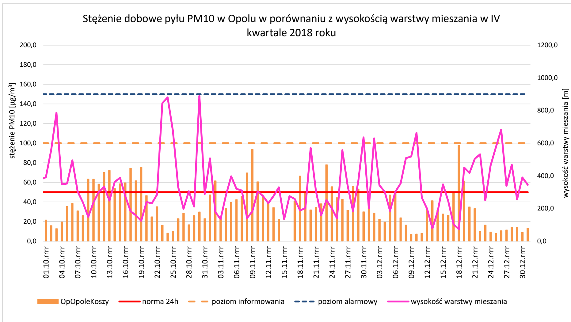
Rysunek 42. Porównanie przebiegu zmienności stężeń 24-godz. pyłu zawieszonego PM10 w IV kwartale 2018 r. w Opolu z wysokością warstwy mieszania.
