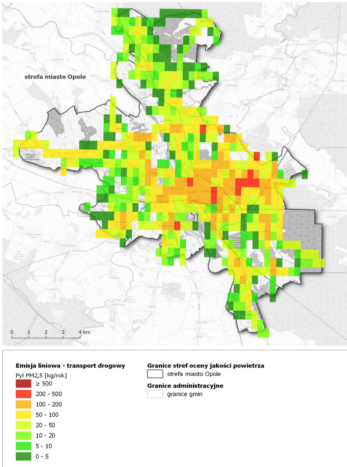
Rysunek 85. Lokalizacja i wielkość emisji pyłu PM 2,5 z sektora transportu drogowego w strefie miasto Opole w roku bazowym 2018 256
