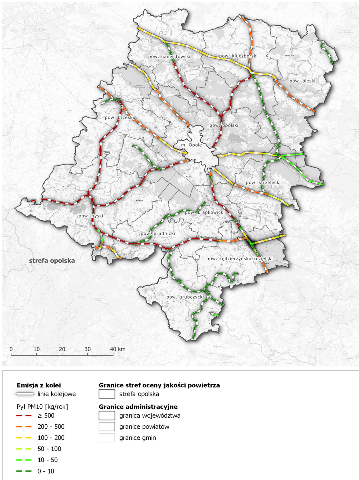
Rysunek 62. Lokalizacja i wielkość emisji pyłu PM10 z kolei w strefie opolskiej w roku bazowym 2018 233
