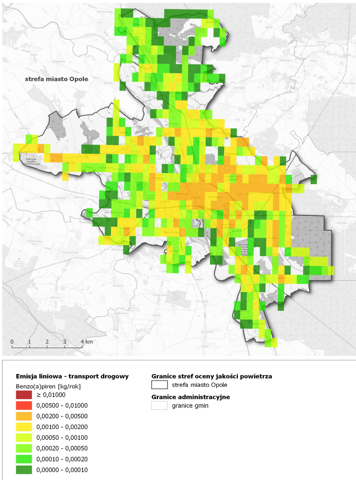
Rysunek 87. Lokalizacja i wielkość emisji benzo(a)pirenu z sektora transportu drogowego w strefie miasto Opole w roku bazowym 2018 258
