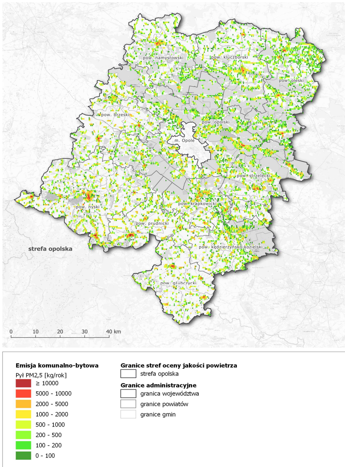
Rysunek 92. Lokalizacja i wielkość emisji pyłu PM 2,5 ze źródeł z sektora komunalno-bytowego w strefie opolskiej w roku bazowym 2018 263
