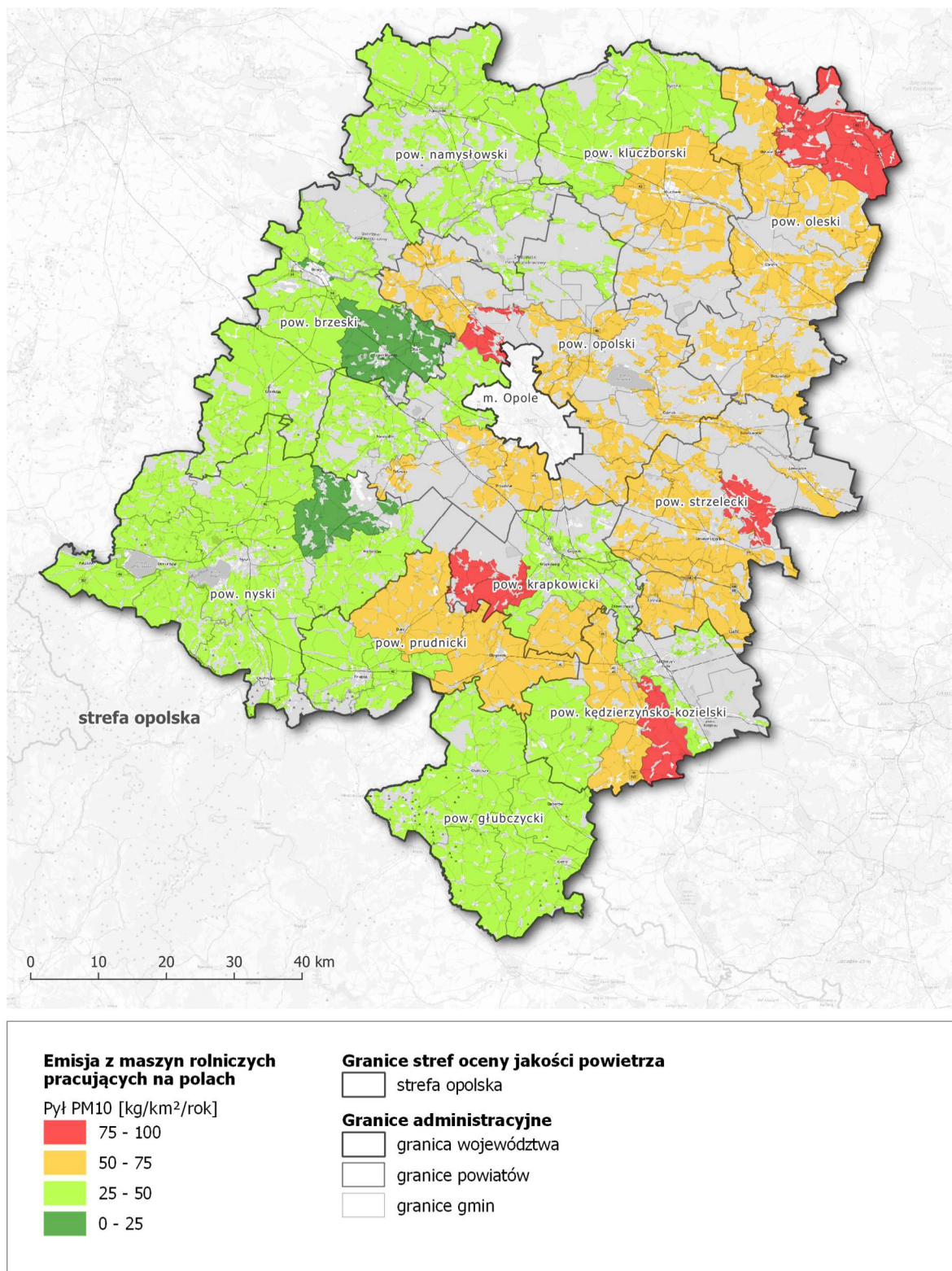
Rysunek 72. Lokalizacja i wielkość emisji pyłu PM10 z maszyn rolniczych w strefie opolskiej w roku bazowym 2018 243
