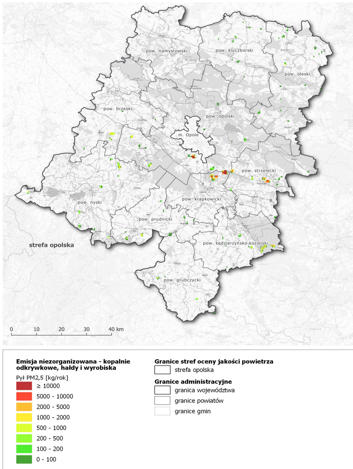
Rysunek 70. Lokalizacja i wielkość emisji pyłu PM 2,5 ze źródeł niezorganizowanych (kopalnie odkrywkowe, hałdy i wyrobiska) w strefie opolskiej w roku bazowym 2018 241
