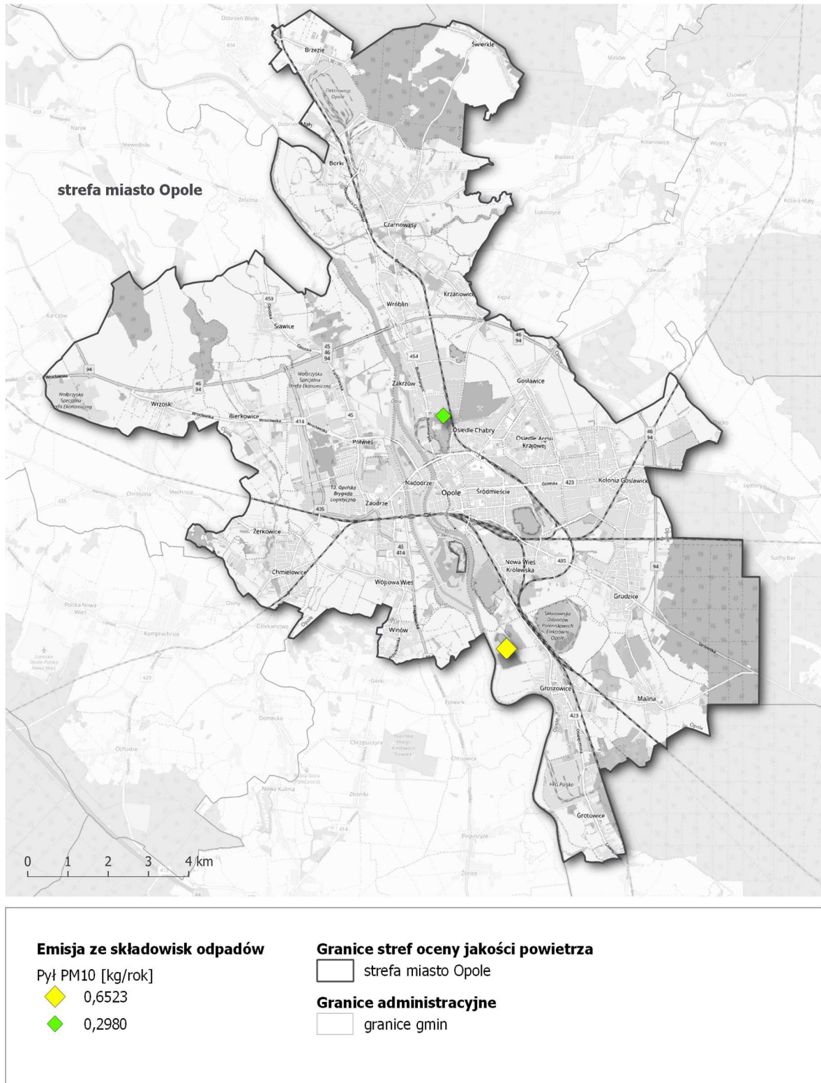
Rysunek 79. Lokalizacja i wielkość emisji pyłu PM10 ze składowisk odpadów w strefie miasto Opole w roku bazowym 2018 250
