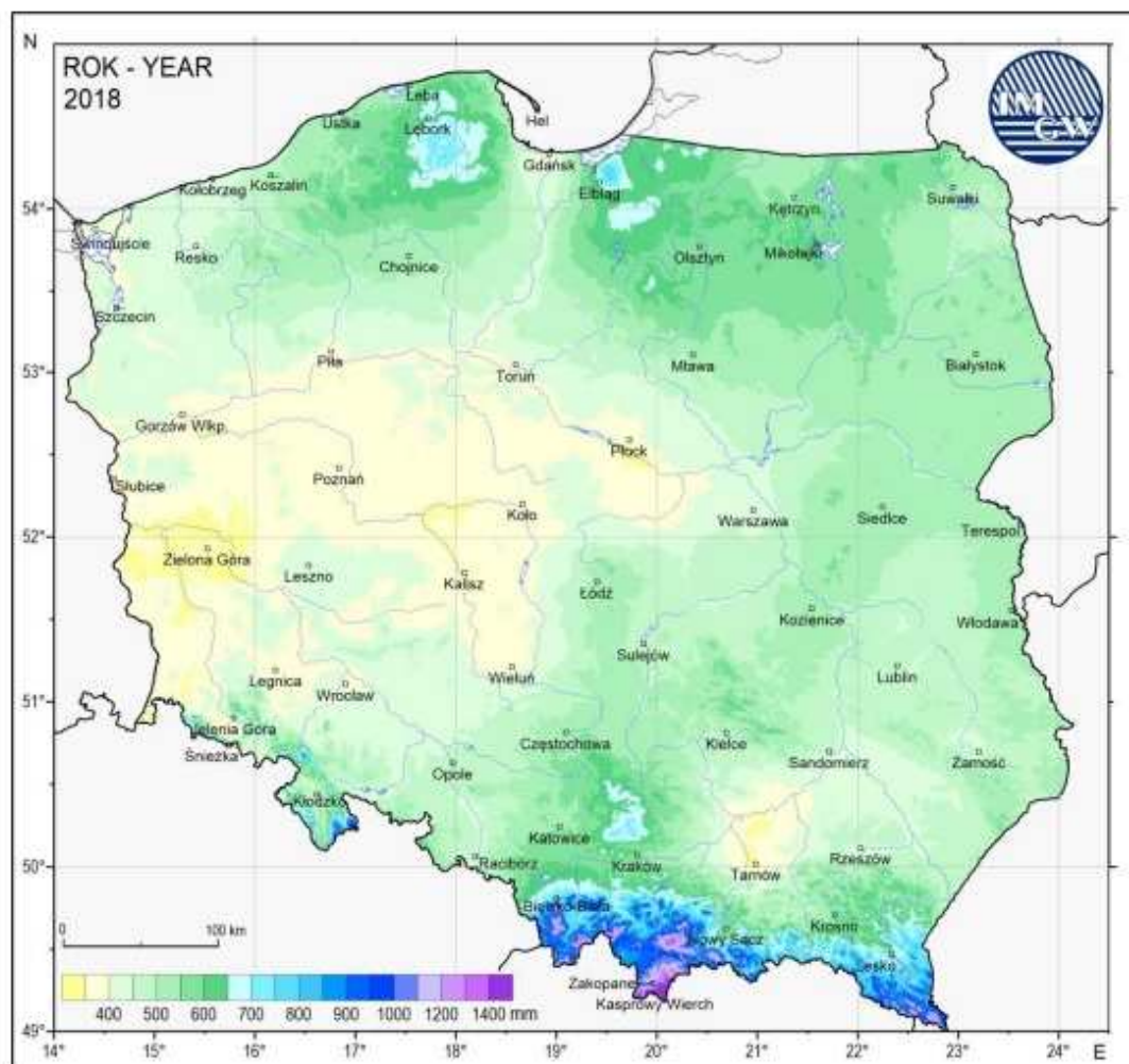
Rysunek 8. Roczne sumy opadów atmosferycznych w roku 2018 58
