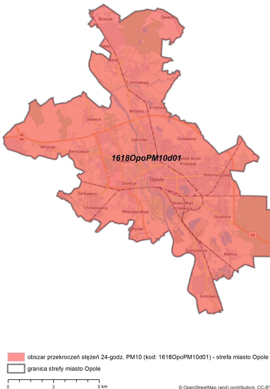
Rysunek 23. Obszar przekroczeń stężeń 24-godzinnych pyłu zawieszzonego PM10 na terenie strefy miasto Opole 90
