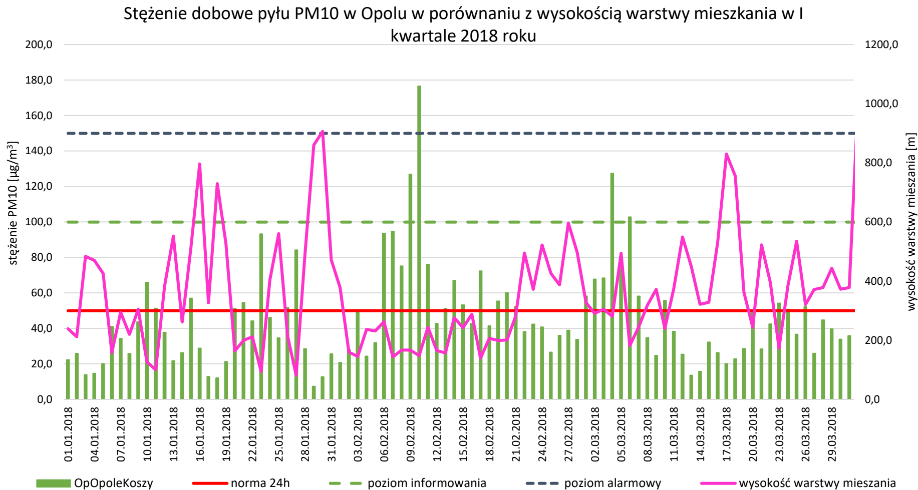
Rysunek 41. Porównanie przebiegu zmienności stężeń 24-godz. pyłu zawieszonego PM10 w I kwartale 2018 r. w Opolu z wysokością warstwy mieszkania.
