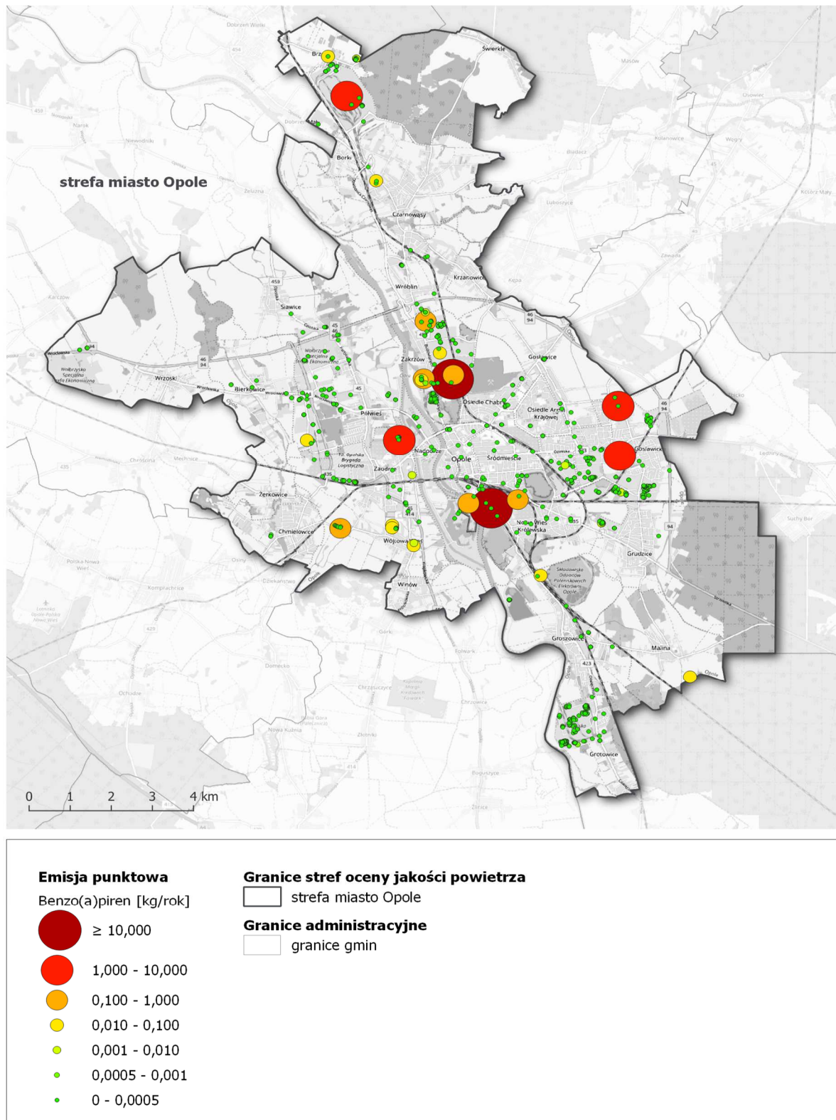
Rysunek 55. Lokalizacja i wielkość emisji benzo(a)pirenu z przemysłu i energetyki w strefie miasto Opole w roku bazowym 2018 226
