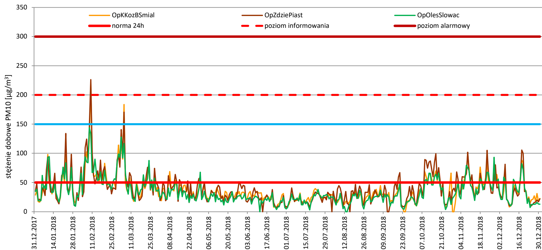
Rysunek 19. Przebieg zmienności stężeń dobowych pyłu zawieszonego PM10 w 2018 roku w strefie opolskiej 83
