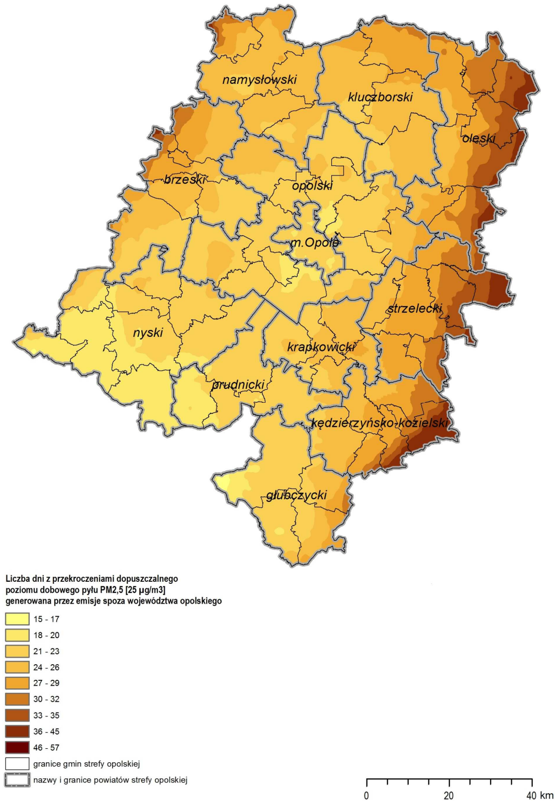
Rysunek 37. Liczba dni z przekroczeniem dopuszczalnego poziomu dobowego pyłu zawieszonego PM 10 generowana przez emisję spoza województwa opolskiego 121
