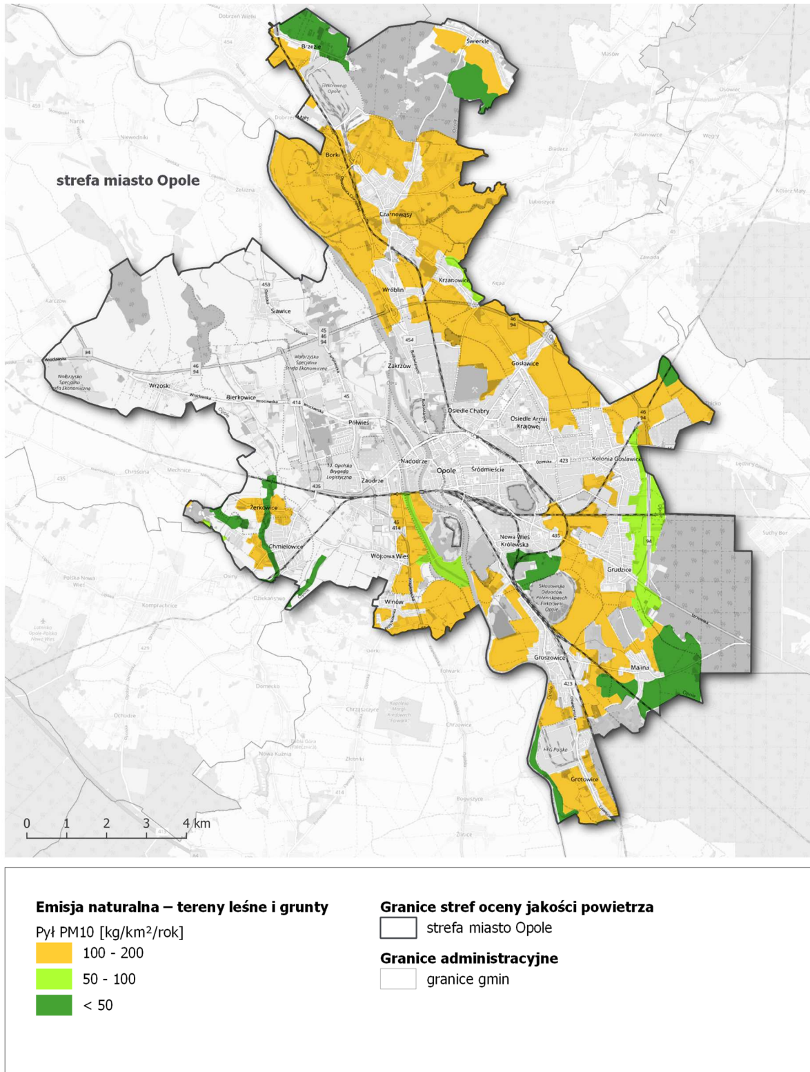
Rysunek 57. Lokalizacja i wielkość emisji pyłu PM10 ze źródeł naturalnych w strefie miasto Opole w roku bazowym 2018 228
