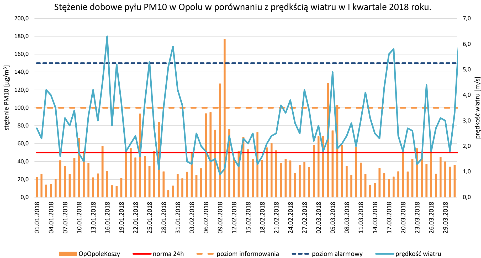
Rysunek 39. Porównanie przebiegu zmienności stężeń 24-godz. pyłu zawieszzonego PM10 w I kwartale 2018 r. w Opolu z prędkością wiatru
