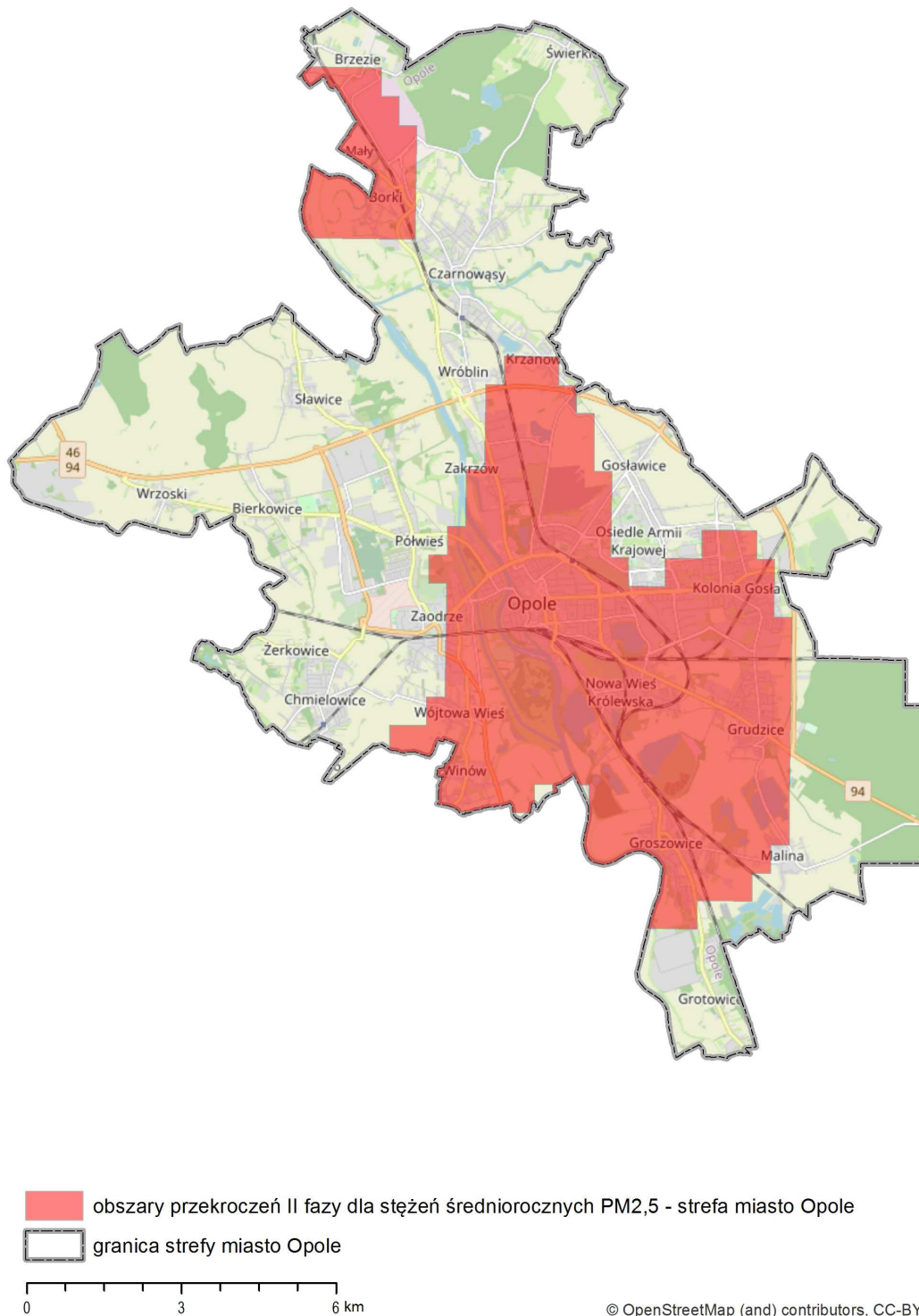
Rysunek 25. Obszary przekroczeń stężeń średniorocznych pyłu zawieszonego PM 2,5 dla tzw. fazy II na terenie strefy miasto Opole w roku 2018 96
