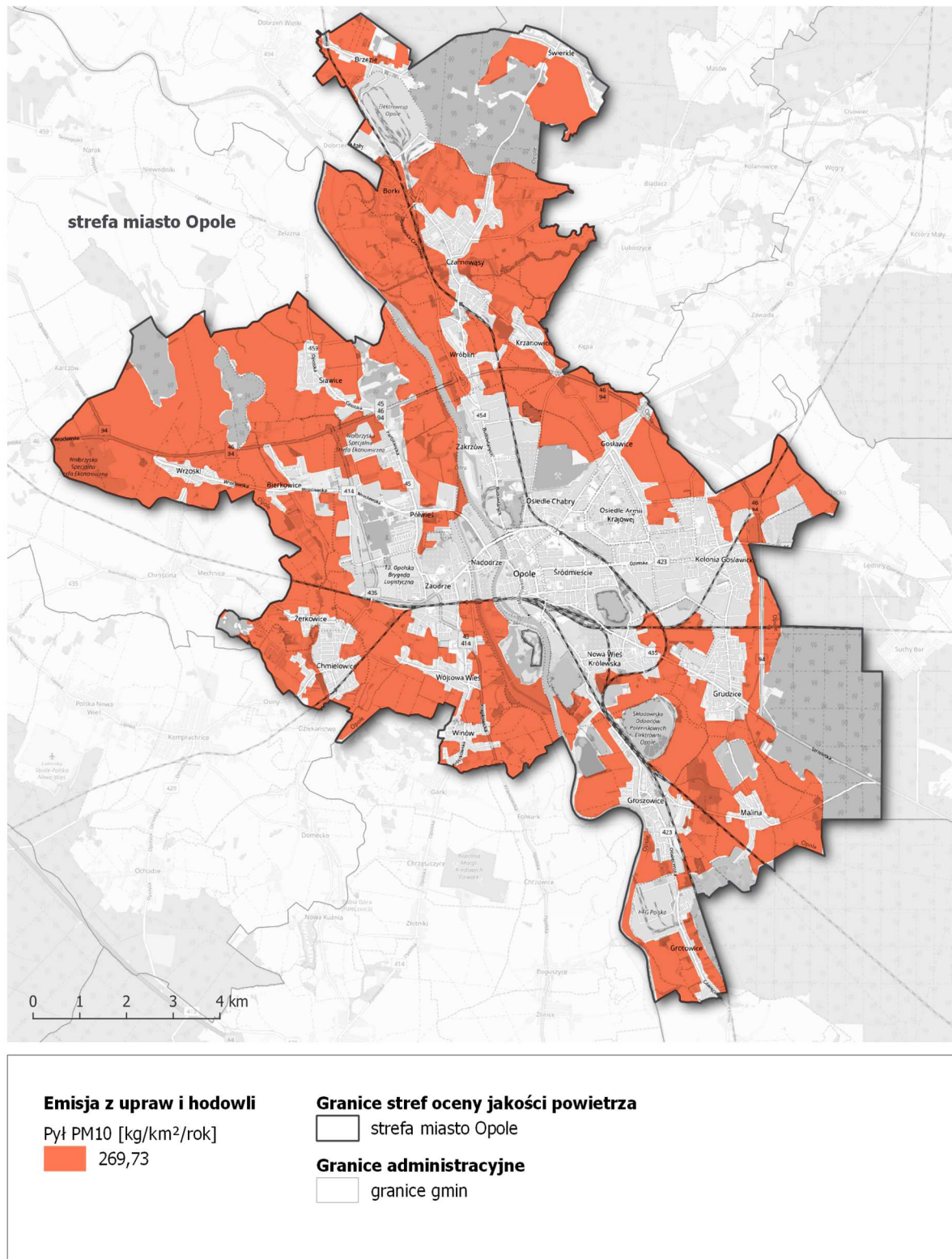
Rysunek 75. Lokalizacja i wielkość emisji pyłu PM10 z upraw i hodowli w strefie miasto Opole w roku bazowym 2018 246
