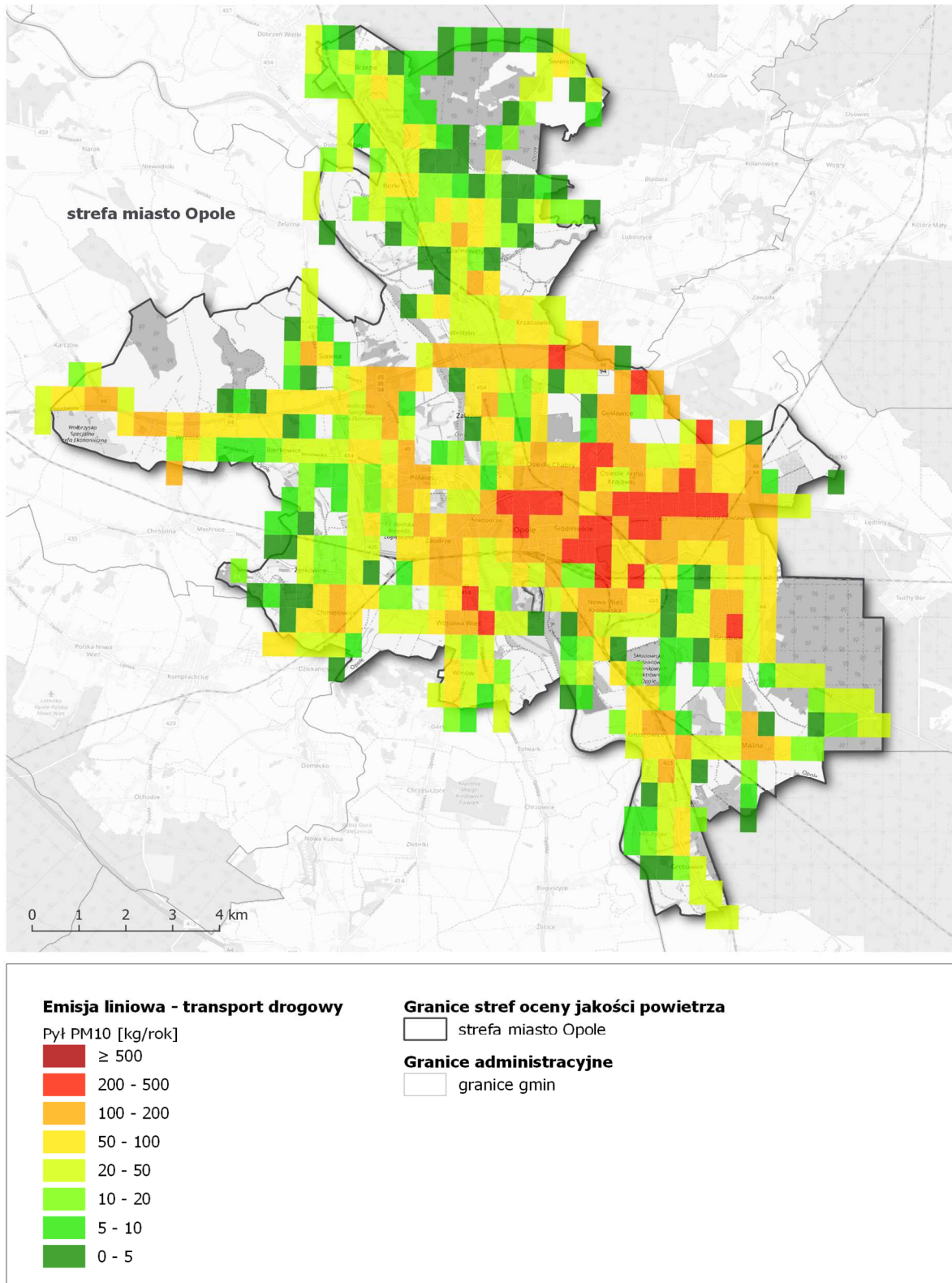
Rysunek 83. Lokalizacja i wielkość emisji pyłu PM10 z sektora transportu drogowego w strefie miasto Opole w roku bazowym 2018 254
