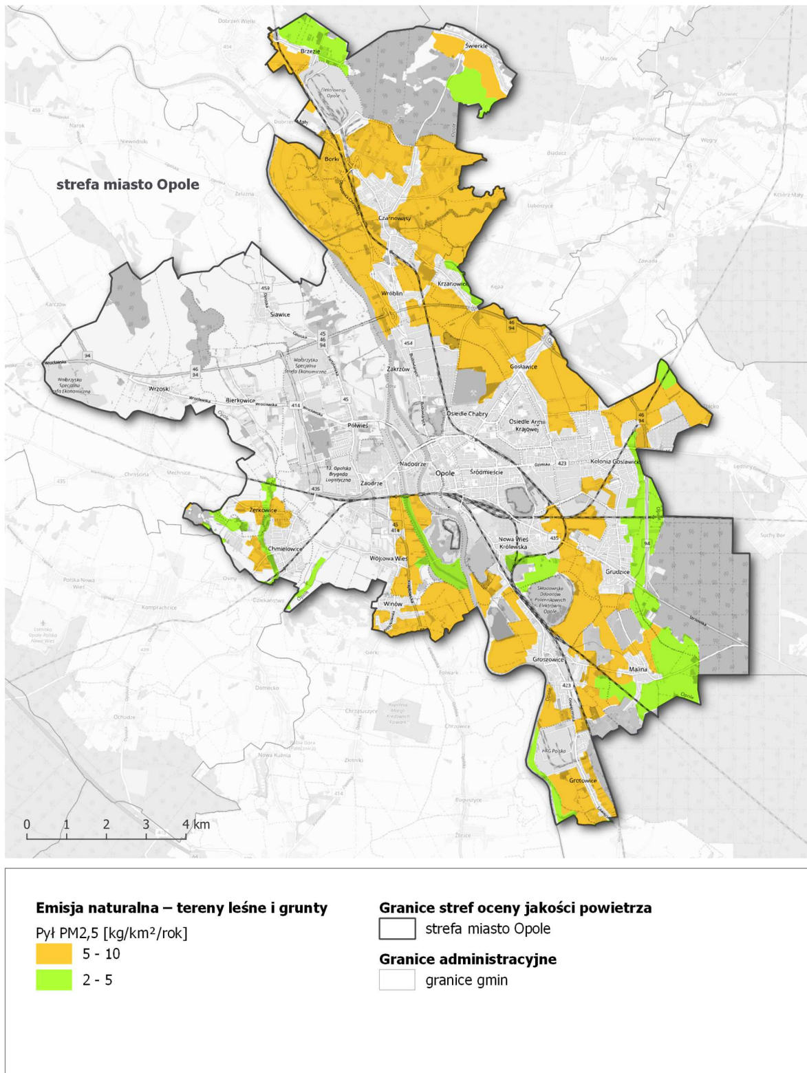
Rysunek 59. Lokalizacja i wielkość emisji pyłu PM 2,5 ze źródeł naturalnych w strefie miasto Opole w roku bazowym 2018 230
