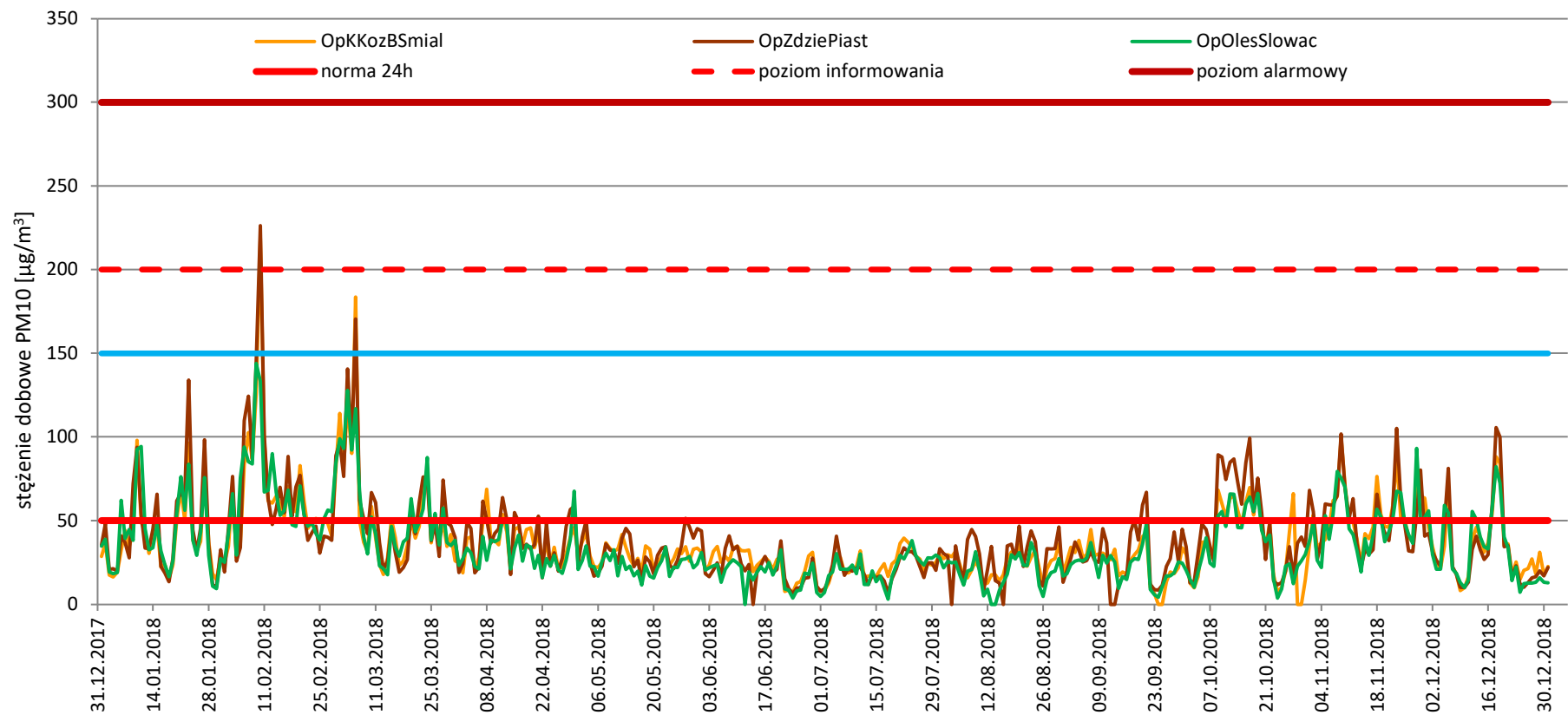
Rysunek 19. Przebieg zmienności stężeń dobowych pyłu zawieszonego PM10 w 2018 roku w strefie opolskiej 83
