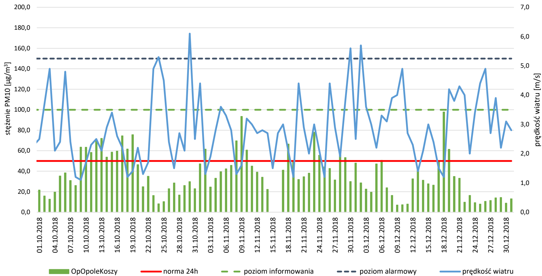
Rysunek 40. Porównanie przebiegu zmienności stężeń 24-godz. pyłu zawieszzonego PM10 w IV kwartale 2018 r. w Opolu z prędkością wiatru.
