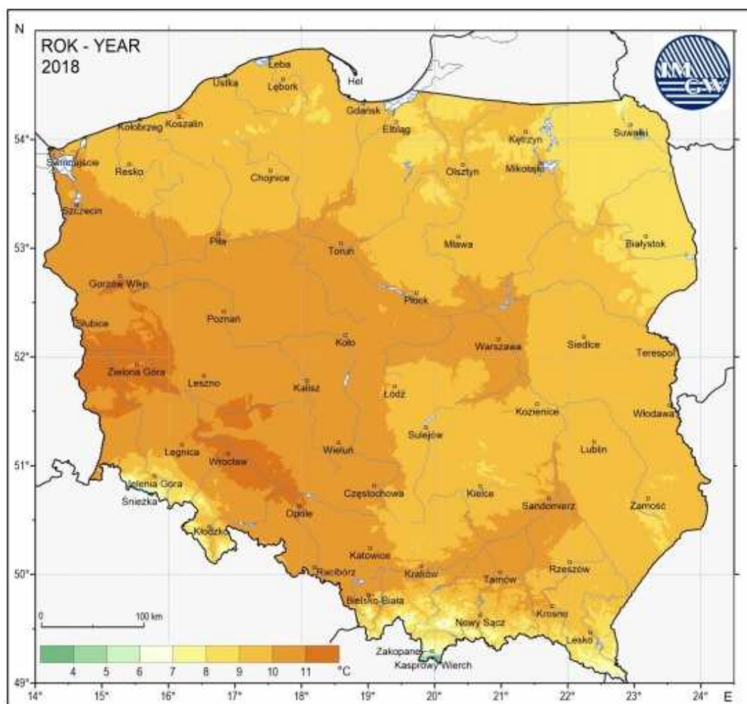
Rysunek 7. Średnia roczna temperatura powietrza w roku 2018 57
