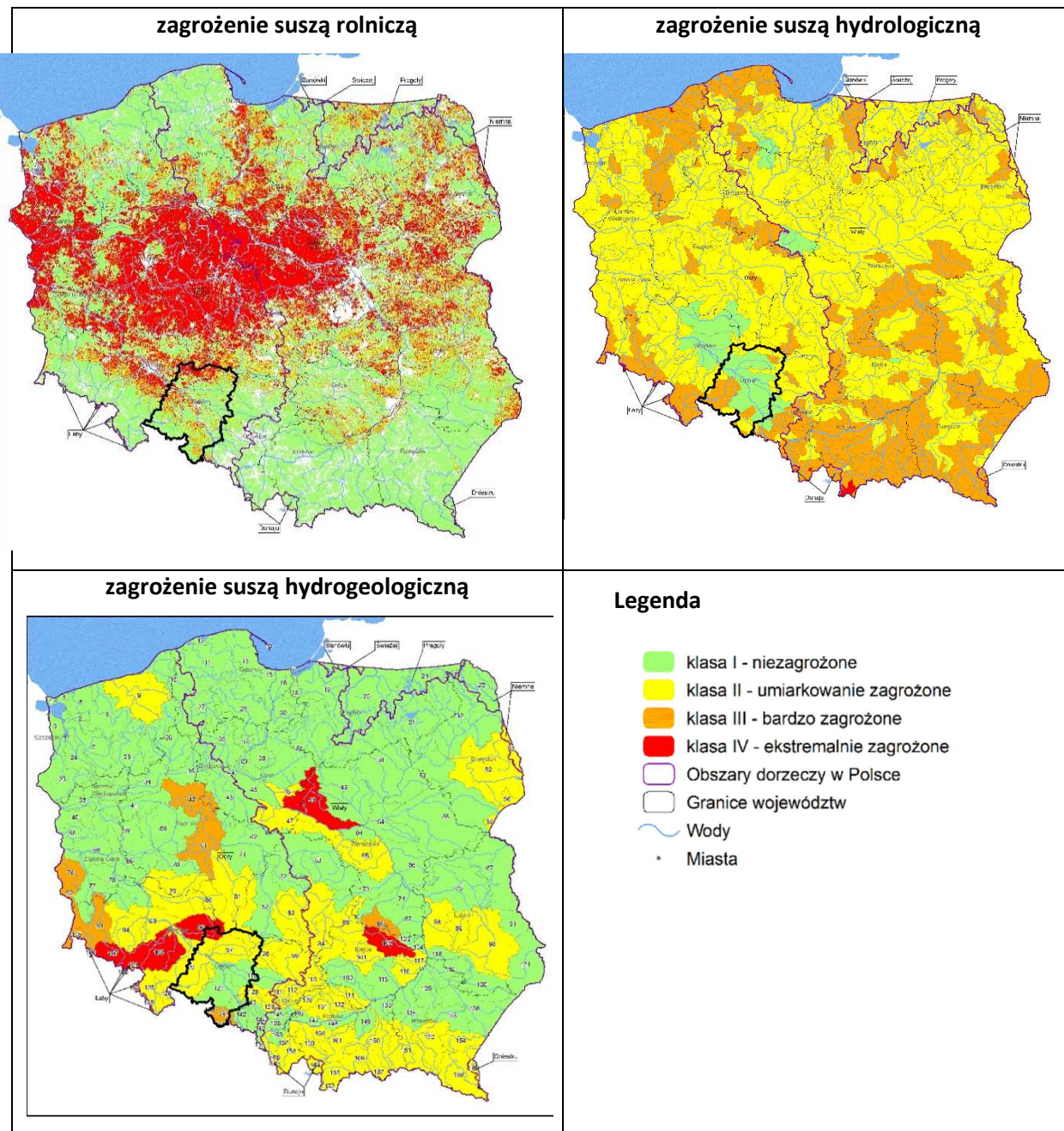
Ryc. 11. Zagrożenie zjawiskiem suszy poszczególnych rodzajów
