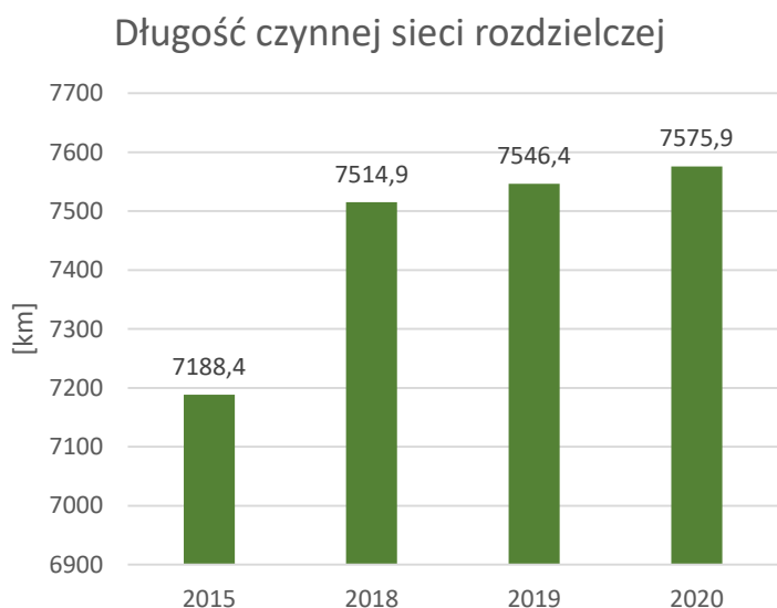
Ryc. 2. Długość czynnej sieci rozdzielczej wodociągowej w latach 2015, 2018 i 2019, 2020 w województwie opolskim
