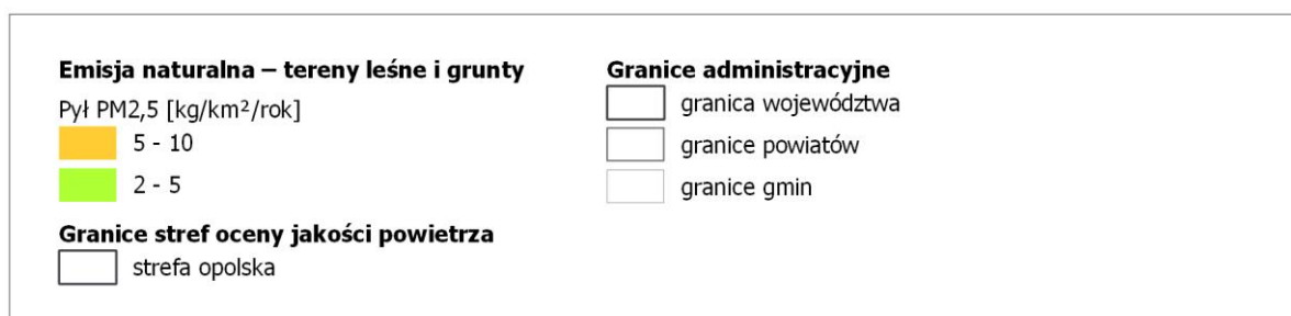
Rysunek 56. Lokalizacja i wielkość emisji pyłu PM 2,5 ze źródeł naturalnych w strefie opolskiej w roku bazowym 2018 228
