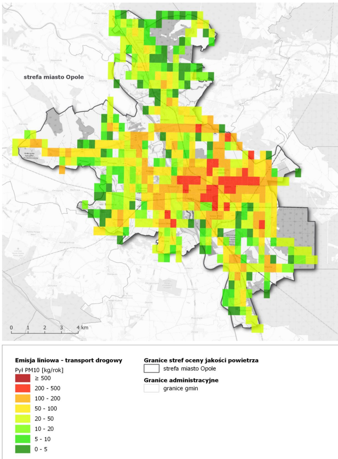
Rysunek 79. Lokalizacja i wielkość emisji pyłu PM10 z sektora transportu drogowego w strefie miasto Opole w roku bazowym 2018 251
