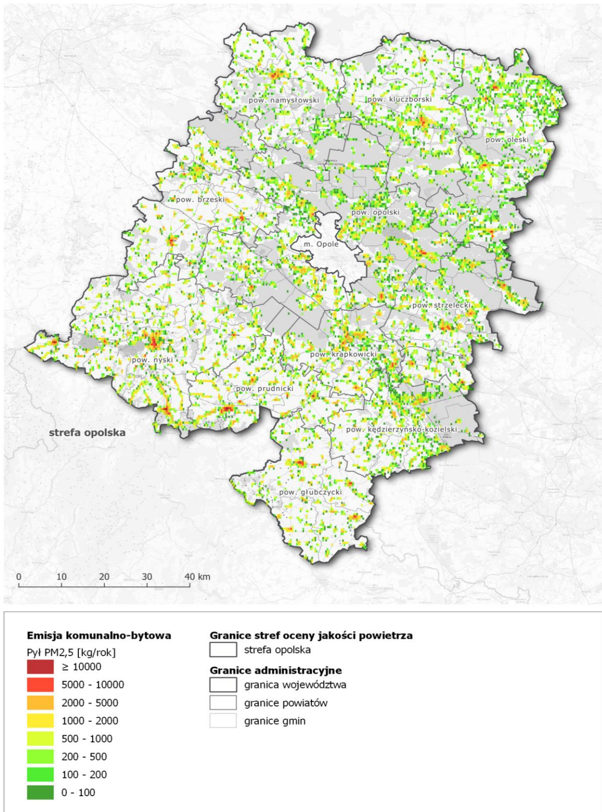
Rysunek 88. Lokalizacja i wielkość emisji pyłu PM 2,5 ze źródeł z sektora komunalno-bytowego w strefie opolskiej w roku bazowym 2018 260
