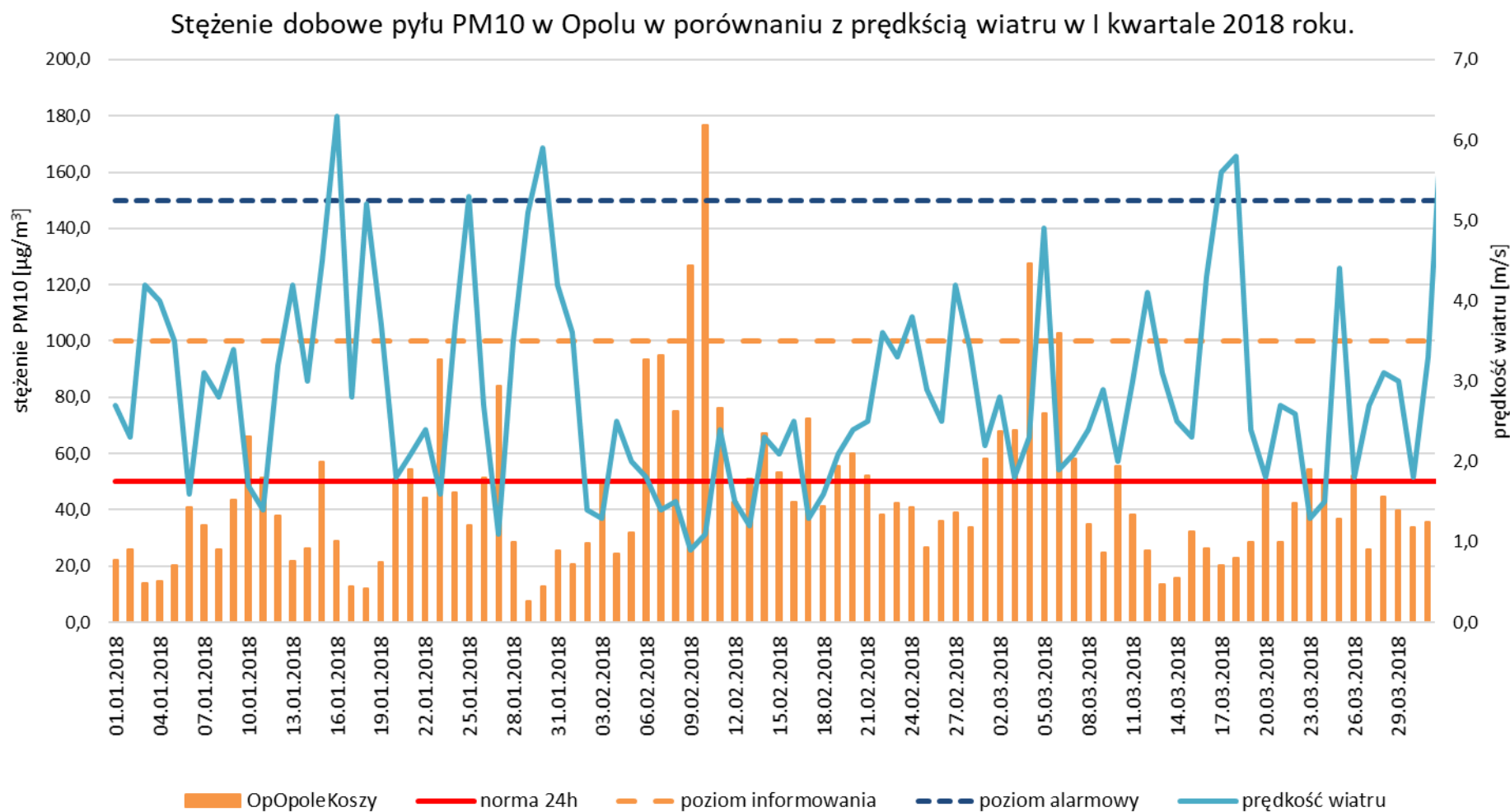
Rysunek 35. Porównanie przebiegu zmienności stężeń 24-godz. pyłu zawieszzonego PM10 w I kwartale 2018 r. w Opolu z prędkością wiatru
