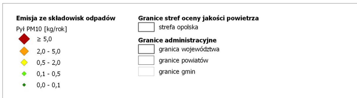
Rysunek 76. Lokalizacja i wielkość emisji pyłu PM10 ze składowisk odpadów w strefie opolskiej w roku bazowym 2018 248
