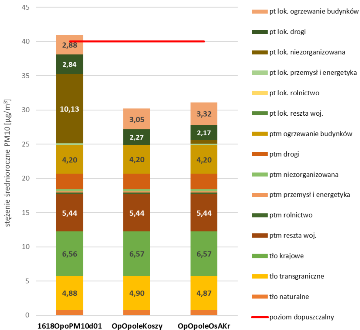
Rysunek 25. Prezentacja poziomów tła regionalnego oraz przyrostu tła miejskiego i lokalnego przyrostu stężeń dla pyłu zawieszonoego PM10 w obszarze przekroczeń i w punktach pomiarowych w Opolu w 2018 roku 108
