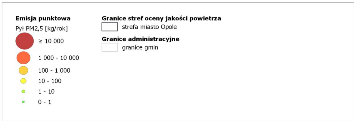
Rysunek 49. Lokalizacja i wielkość emisji pyłu PM 2,5 z przemysłu i energetyki w strefie miasto Opole w roku bazowym 2018 221
