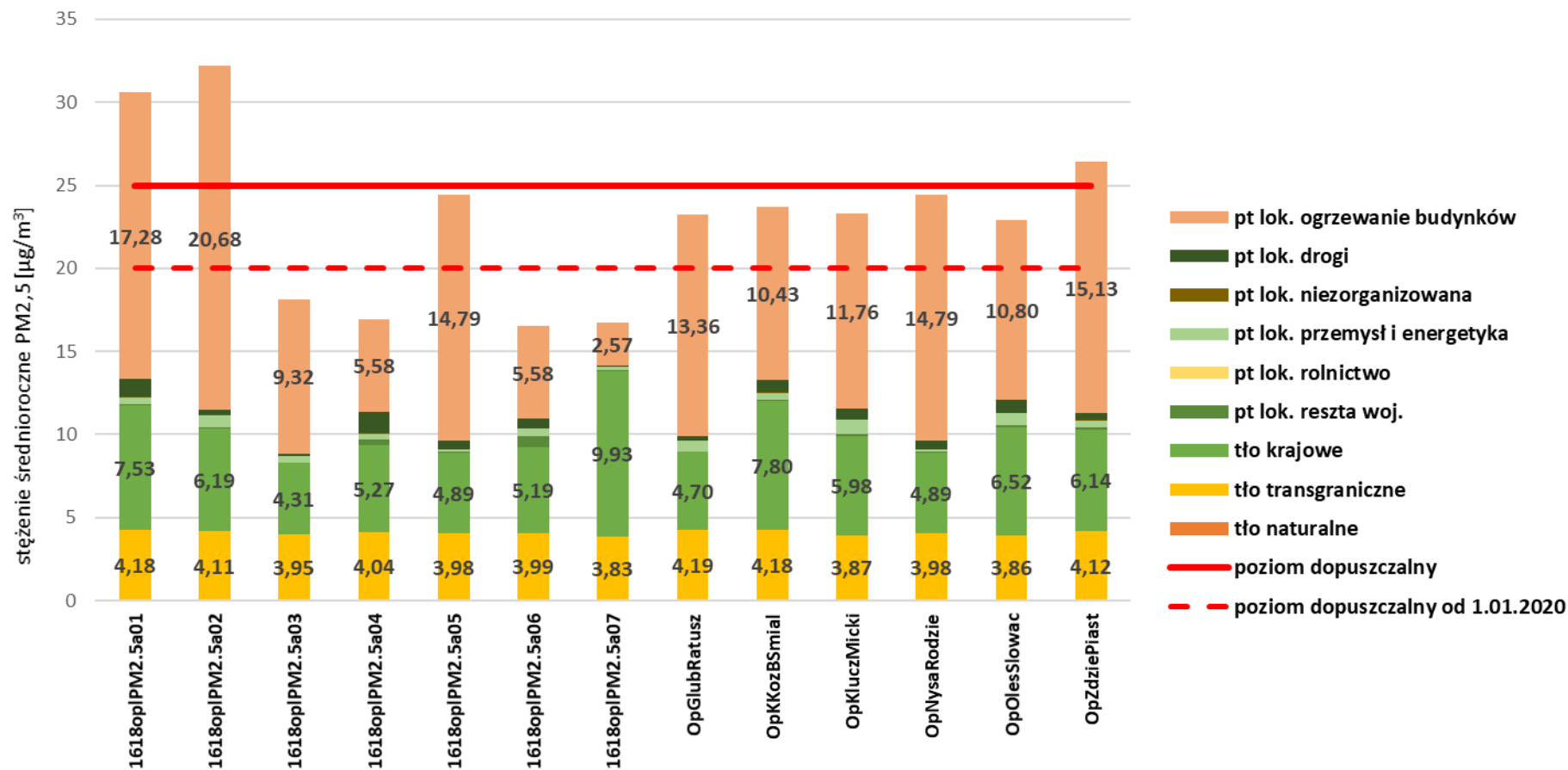
Rysunek 30. Prezentacja poziomów tła regionalnego oraz lokalnego przyrostu stężeń dla pyłu zawieszono PM 2,5 w obszarach przekroczeń i w punktach pomiarowych w strefie opolskiej w 2018 roku 113
