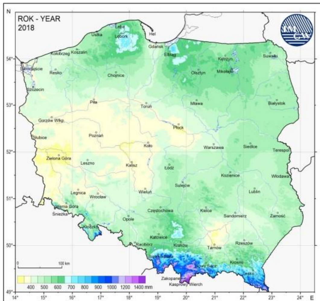
Rysunek 4. Roczne sumy opadów atmosferycznych w roku 2018 56
