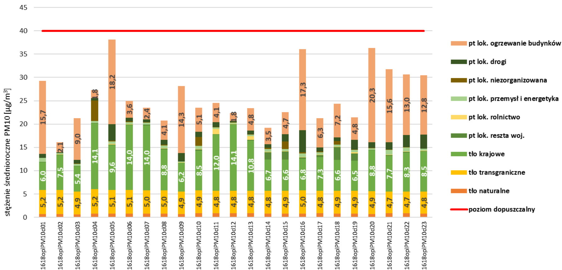
Rysunek 28. Prezentacja poziomów tła regionalnego oraz lokalnego przyrostu stężeń dla pyłu zawieszzonego PM10 w obszarach przekroczeń w strefie opolskiej w 2018 roku 111
