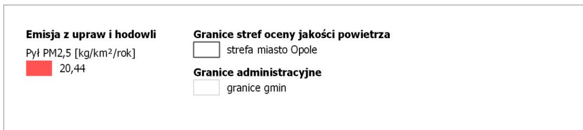
Rysunek 73. Lokalizacja i wielkość emisji pyłu PM2,5 z upraw i hodowli w strefie miasto Opole w roku bazowym 2018 245
