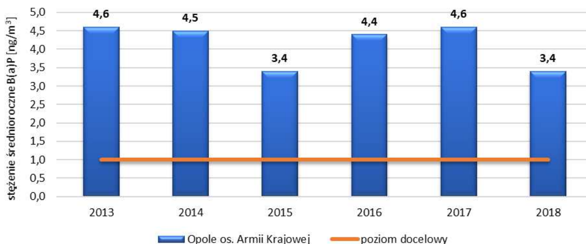
Rysunek 11. Wyniki pomiarów stężeń średniorocznych benzo(a)pirenu w latach 2013-2018 w strefie miasto Opole 72
