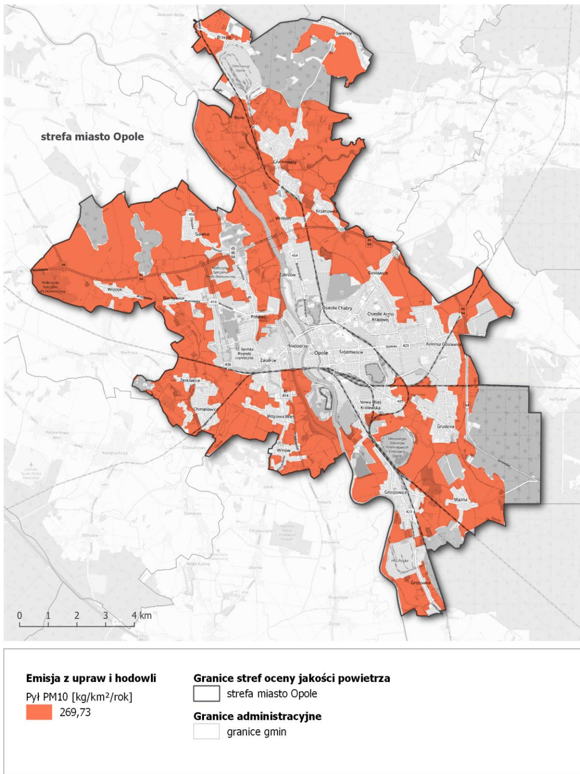
Rysunek 71. Lokalizacja i wielkość emisji pyłu PM10 z upraw i hodowli w strefie miasto Opole w roku bazowym 2018 243
