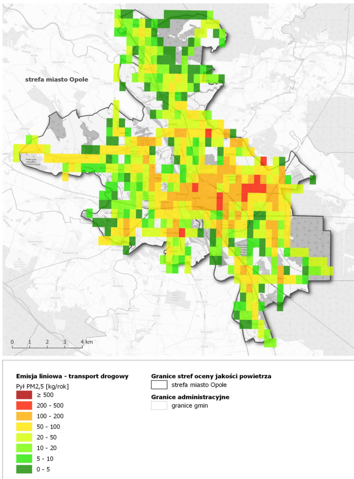
Rysunek 81. Lokalizacja i wielkość emisji pyłu PM 2,5 z sektora transportu drogowego w strefie miasto Opole w roku bazowym 2018 253
