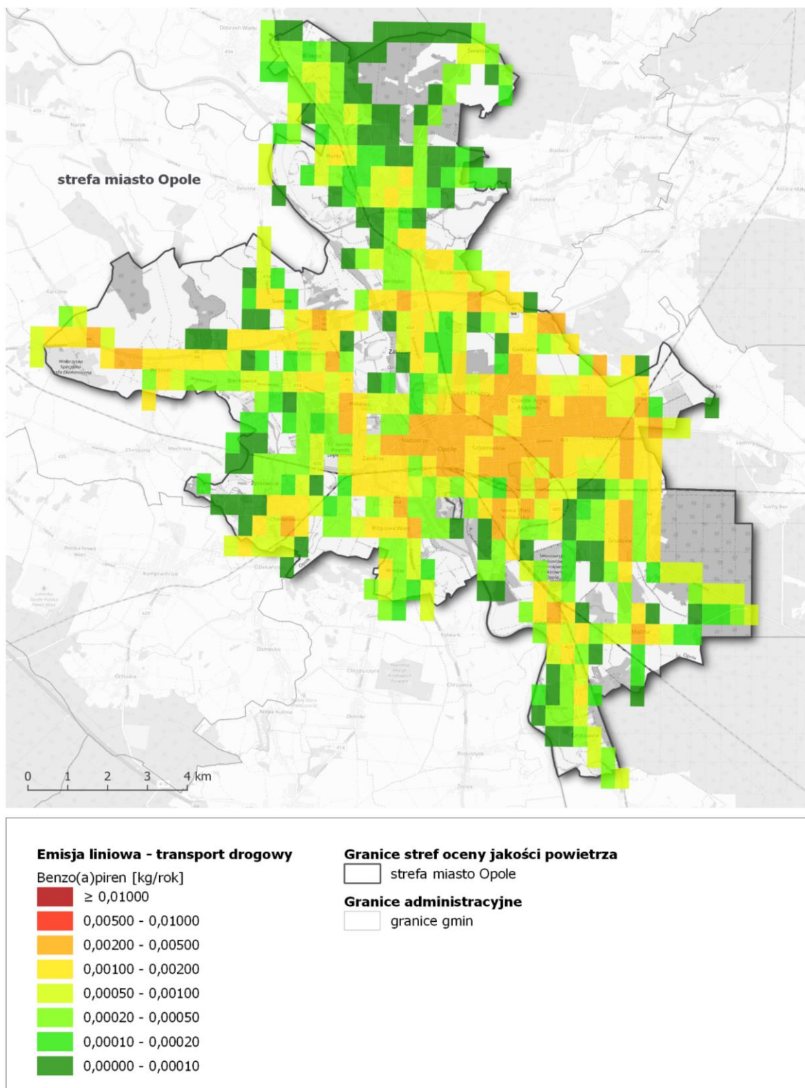
Rysunek 83. Lokalizacja i wielkość emisji benzo(a)pirenu z sektora transportu drogowego w strefie miasto Opole w roku bazowym 2018 255
