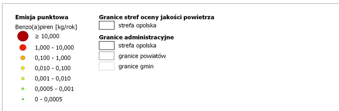
Rysunek 52. Lokalizacja i wielkość emisji benzo(a)pirenu z przemysłu i energetyki w strefie opolskiej w roku bazowym 2018 224
