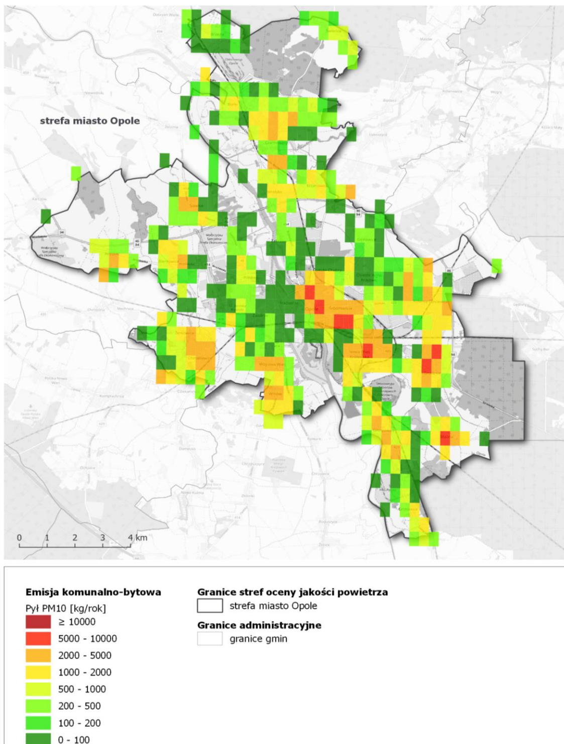
Rysunek 85. Lokalizacja i wielkość emisji pyłu PM10 ze źródeł z sektora komunalno-bytowego w strefie miasto Opole w roku bazowym 2018 257
