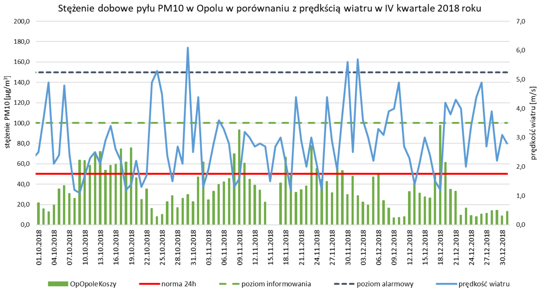
Rysunek 36. Porównanie przebiegu zmienności stężeń 24-godz. pyłu zawieszzonego PM10 w IV kwartale 2018 r. w Opolu z prędkością wiatru.
