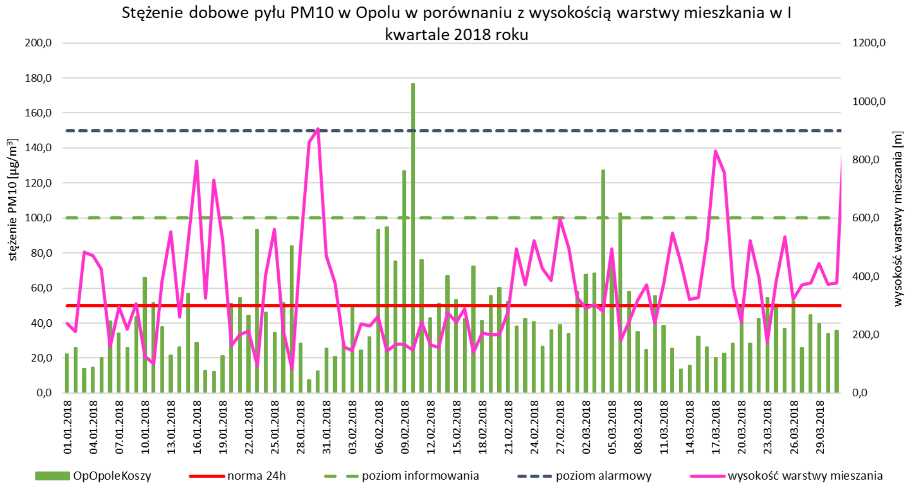
Rysunek 37. Porównanie przebiegu zmienności stężeń 24-godz. pyłu zawieszzonego PM10 w I kwartale 2018 r. w Opolu z wysokością warstwy mieszkania.
