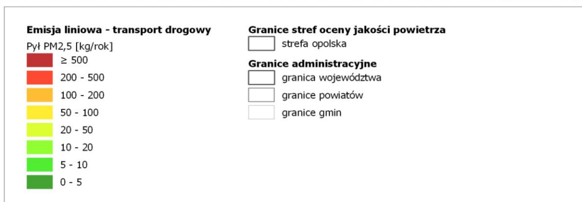
Rysunek 82. Lokalizacja i wielkość emisji pyłu PM 2,5 z sektora transportu drogowego w strefie opolskiej w roku bazowym 2018 254
