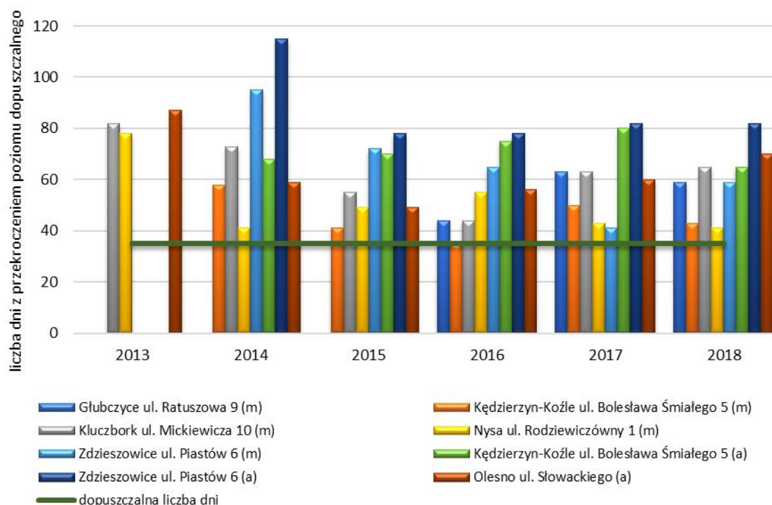
Rysunek 14. Liczba dni z przekroczeniem poziomu dopuszczalnego 24-godzinnej pyłu zawieszonego PM10 w latach 2013-2018 w punktach pomiarowych w strefie opolskiej 78
