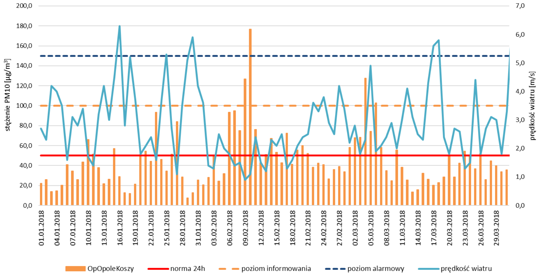
Stężenie dobowe pyłu PM10 w Opolu w porównaniu z prędkością wiatru w I kwartale 2018 roku.
