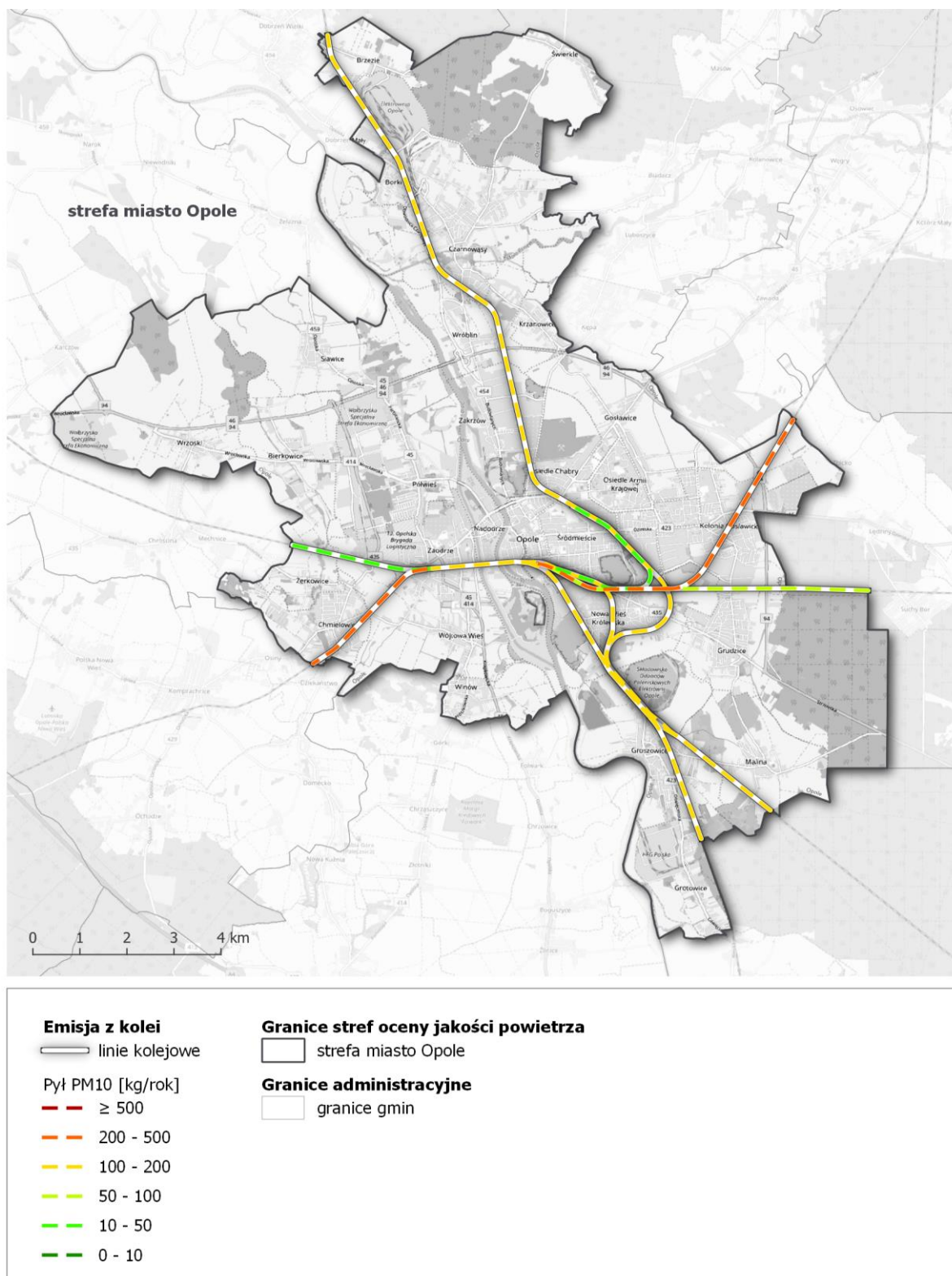
Rysunek 57. Lokalizacja i wielkość emisji pyłu PM10 z kolei w strefie miasto Opole w roku bazowym 2018 229
