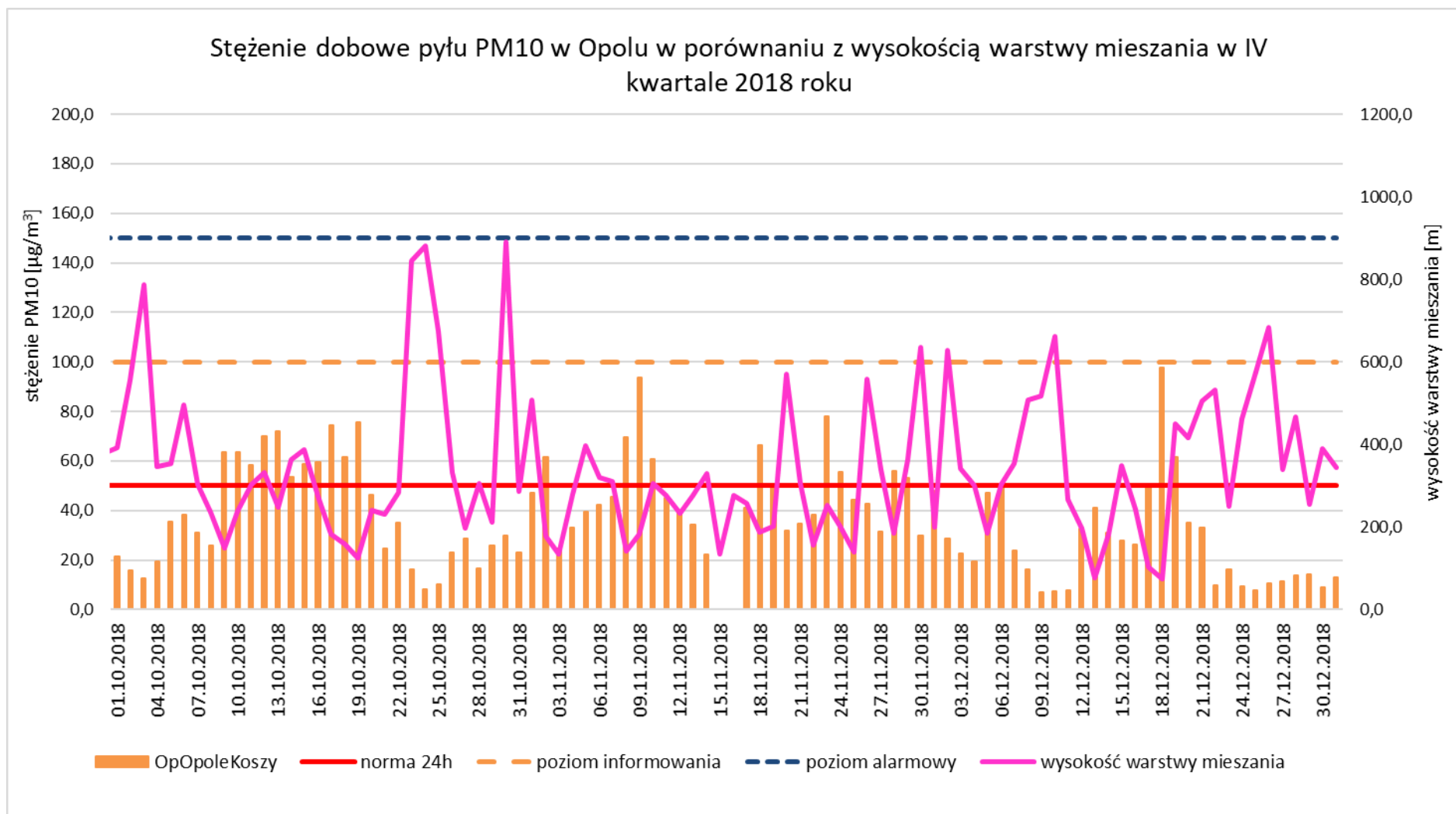
Rysunek 38. Porównanie przebiegu zmienności stężeń 24-godz. pyłu zawieszonoego PM10 w IV kwartale 2018 r. w Opolu z wysokością warstwy mieszania.
