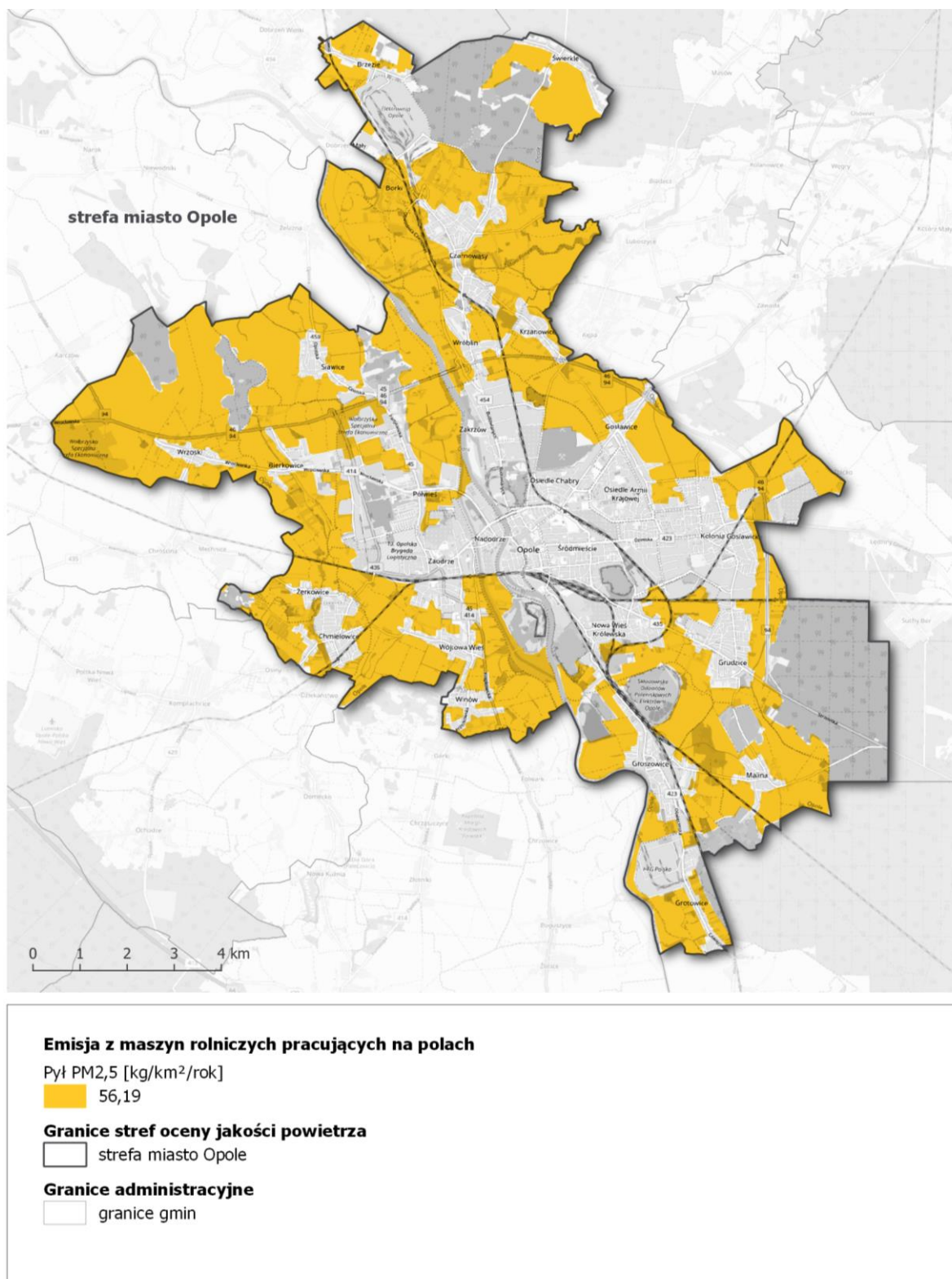
Rysunek 69. Lokalizacja i wielkość emisji pyłu PM 2,5 z maszyn rolniczych w strefie miasto Opole w roku bazowym 2018 241
