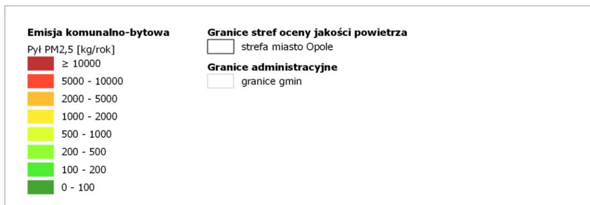
Rysunek 87. Lokalizacja i wielkość emisji pyłu PM 2,5 ze źródeł z sektora komunalno-bytowego w strefie miasto Opole w roku bazowym 2018 259
