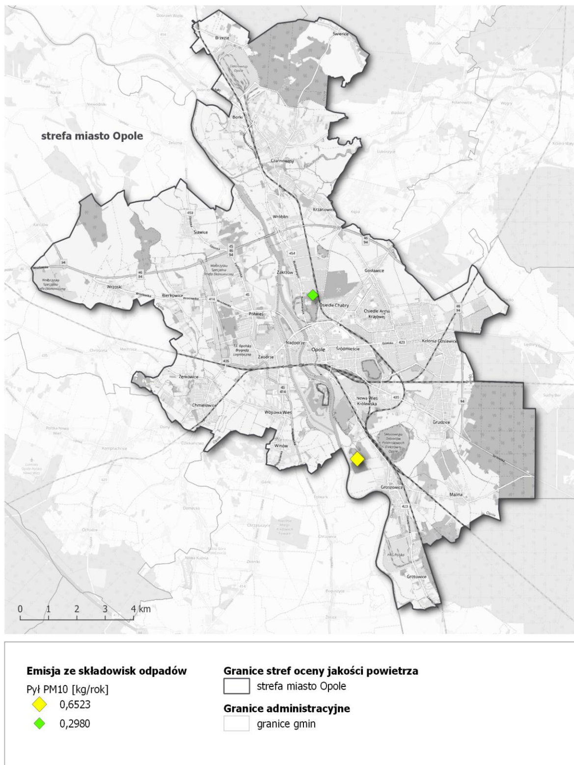
Rysunek 75. Lokalizacja i wielkość emisji pyłu PM10 ze składowisk odpadów w strefie miasto Opole w roku bazowym 2018 247
