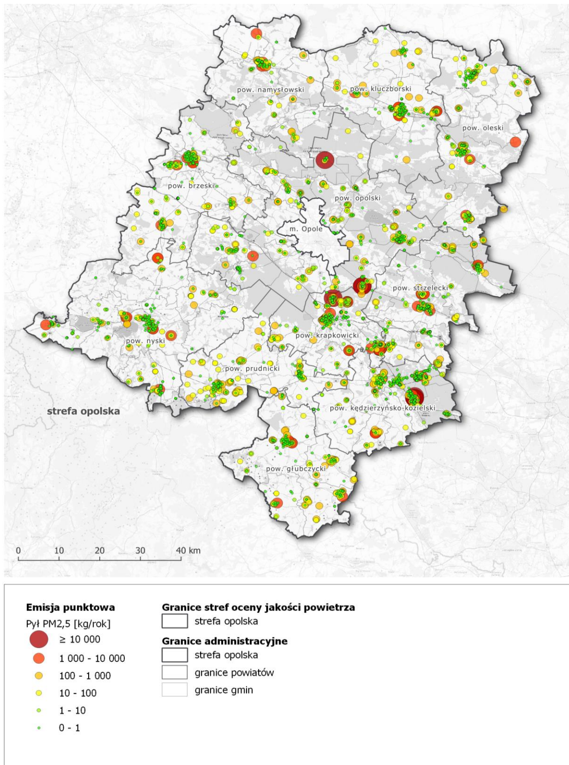
Rysunek 50. Lokalizacja i wielkość emisji pyłu PM 2,5 z przemysłu i energetyki w strefie opolskiej w roku bazowym 2018 222
