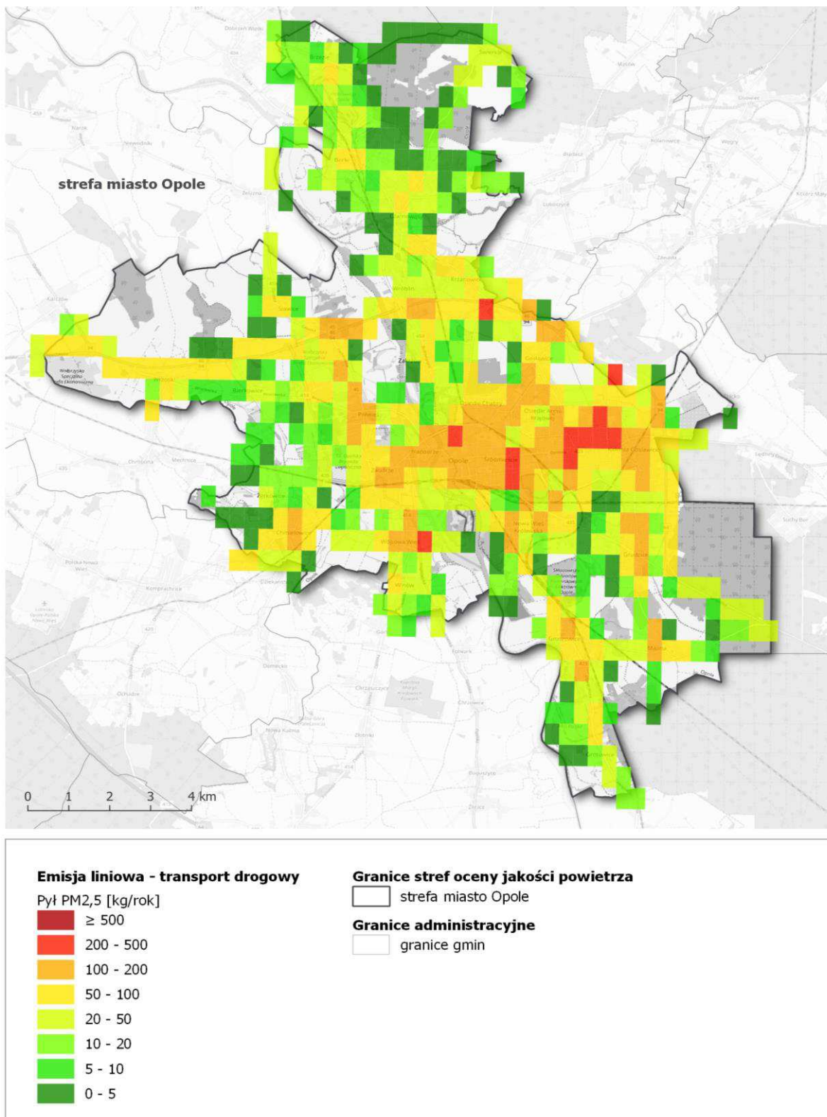
Rysunek 78. Lokalizacja i wielkość emisji pyłu PM 2,5 z sektora transportu drogowego w strefie miasto Opole w roku bazowym 2018 232
