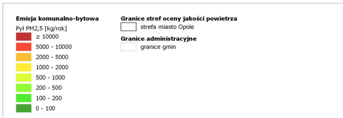
Rysunek 84. Lokalizacja i wielkość emisji pyłu PM 2,5 ze źródeł z sektora komunalno-bytowego w strefie miasto Opole w roku bazowym 2018 238
