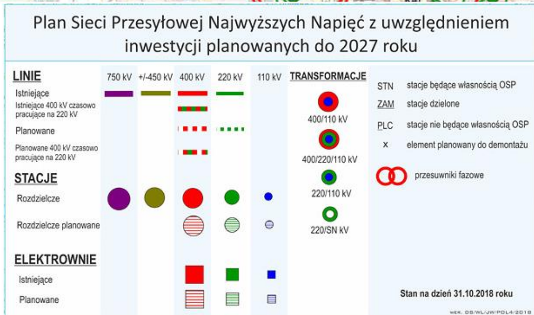
Rysunek 4. Fragment krajowego systemu przesyłowego energii elektrycznej w rejonie Gminy Gorzów Śląski
