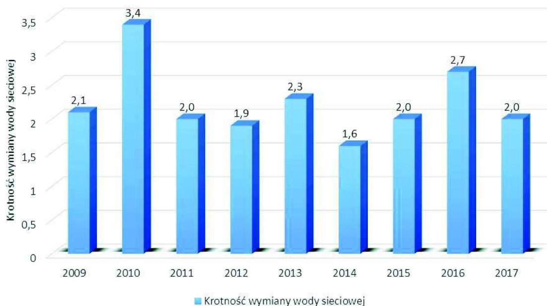
Wykres 21 Krotność wymiany wody sieciowej
