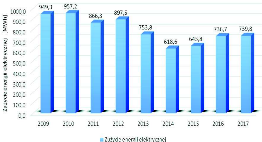
Wykres 13 Przystawienie zużycia energii elektrycznej w latach 2009 - 2017
