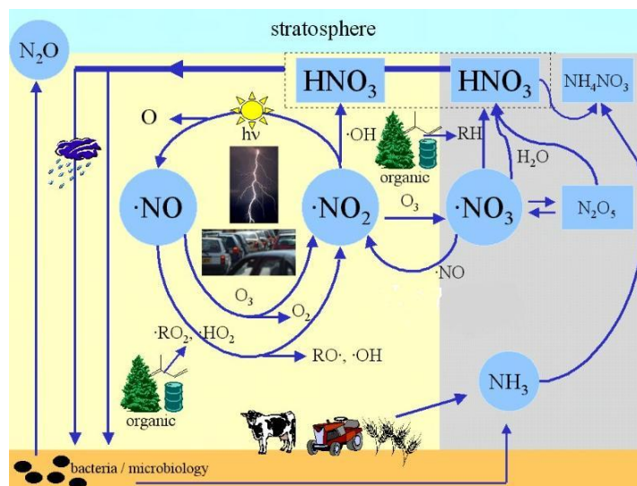
Rysunek 8. Procesy i wybrane reakcje chemiczne tlenków azotu w atmosferze 43
