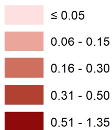
Rysunek 73. Rozkład emisji liniowej pyłu zawieszonego PM10 z dróg powiatowych i gminnych w roku 2016 na terenie strefy opolskiej (źródło: opracowanie własne).
