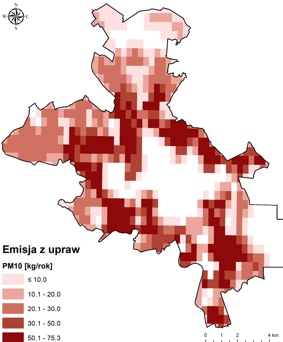
Rysunek 77. Rozkład emisji z upraw, nawożenia i maszyn rolniczych pyłu zawieszzonego PM10 w roku 2016 na terenie strefy miasto Opole (źródło: opracowanie własne).
