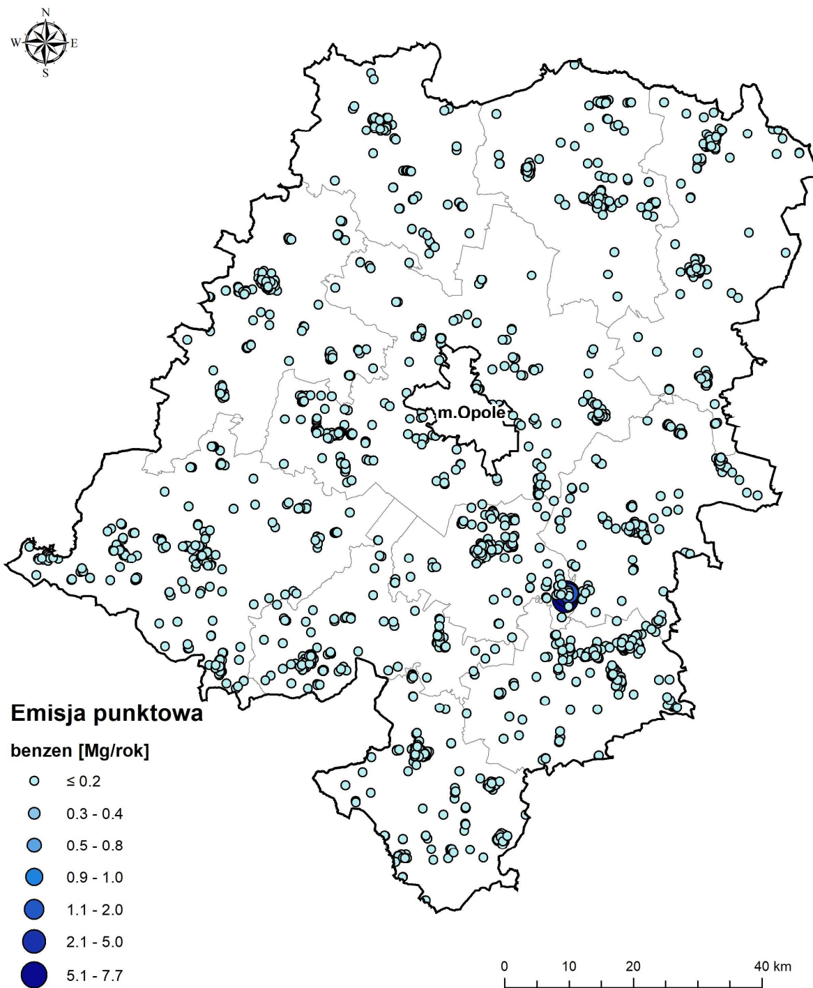
Rysunek 56. Rozkład emisji punktowej benzenu w roku 2016 na terenie strefy opolskiej (źródło: opracowanie własne).
