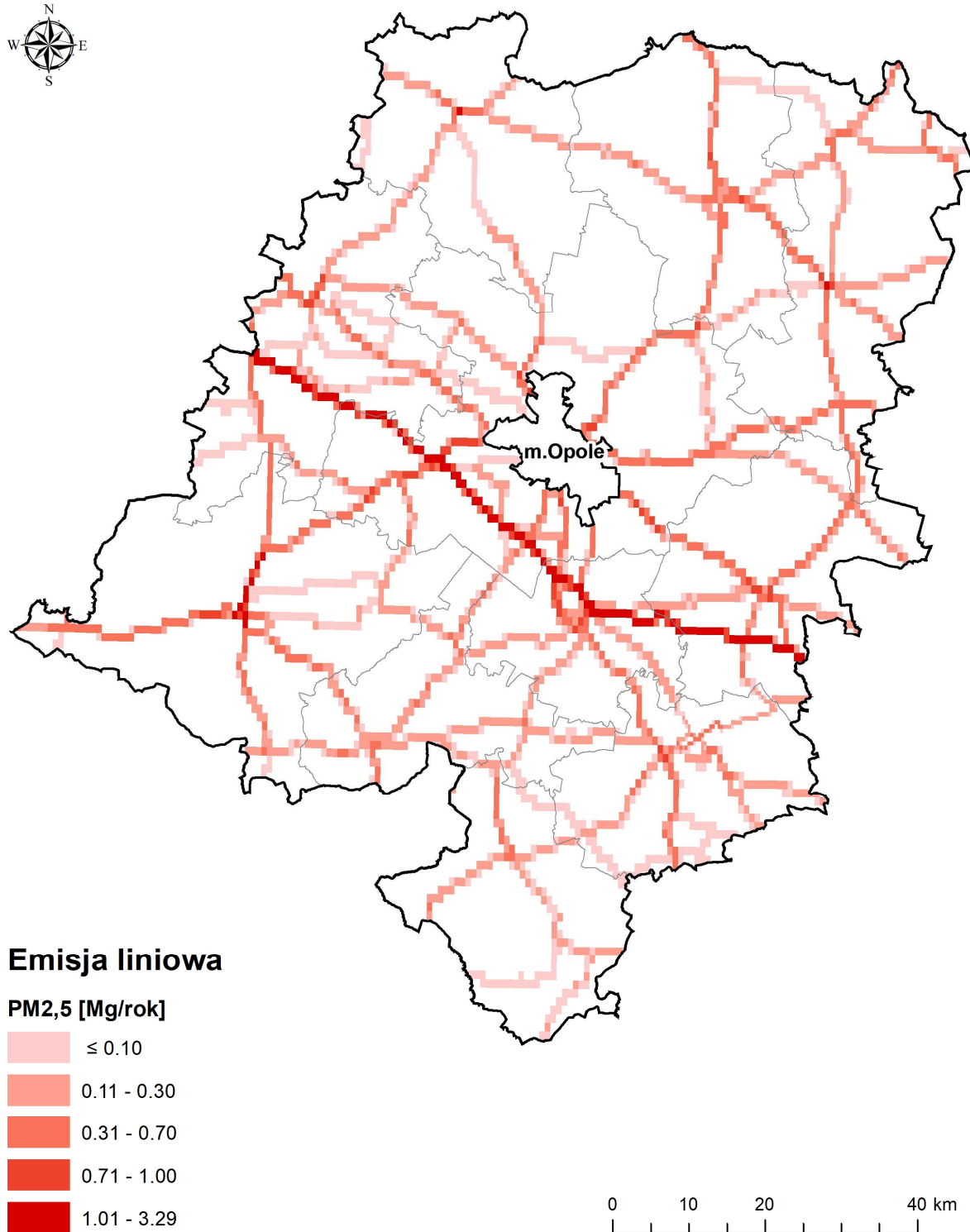
Rysunek 70. Rozkład emisji liniowej pyłu zawieszonoego PM2,5 z dróg krajowych i wojewódzkich w roku 2016 na terenie strefy opolskiej (źródło: opracowanie własne).
