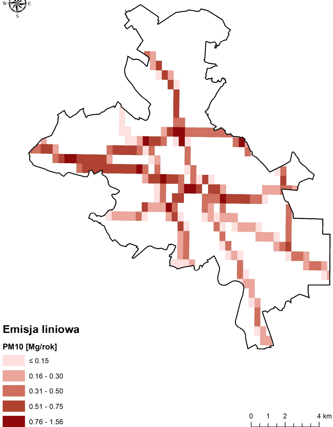
Rysunek 65. Rozkład emisji liniowej pyłu zawieszonego PM10 z dróg krajowych i wojewódzkich w roku 2016 na terenie miasta Opola (źródło: opracowanie własne).
