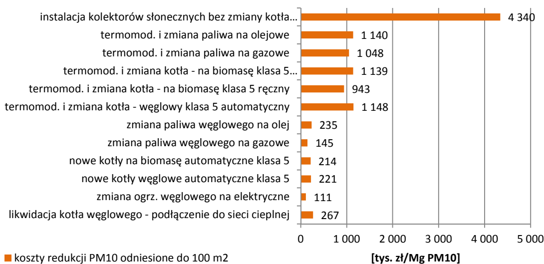
Rysunek 87. Porównanie wskaźników kosztowych redukcji pyłu zawieszonego PM10 z indywidualnych systemów grzewczych (źródło: opracowanie własne na podstawie aktualnych cen w 2016 roku).
