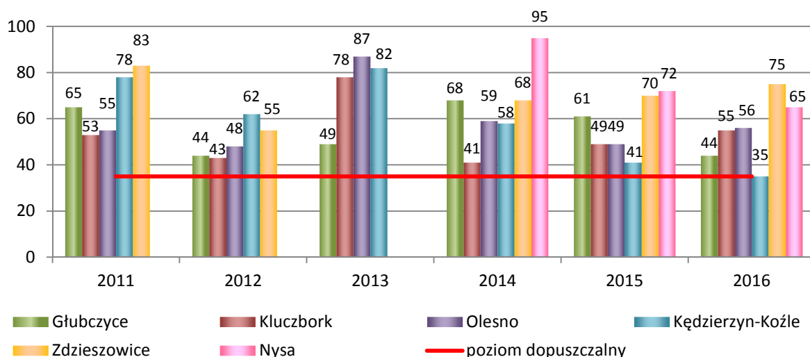
Rysunek 22. Ilość dni z przekroczeniem dopuszczalnego poziomu 24-godzinnej średniej zawieszonych pyłu PM10 w strefie opolskiej w latach 2011-2016 (źródło: opracowanie własne na podstawie danych WIOŚ).
