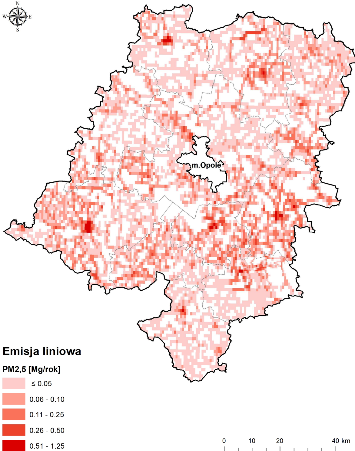
Rysunek 74. Rozkład emisji liniowej pyłu zawieszanego PM 2,5 z dróg powiatowych i gminnych w roku 2016 na terenie strefy opolskiej (źródło: opracowanie własne).
