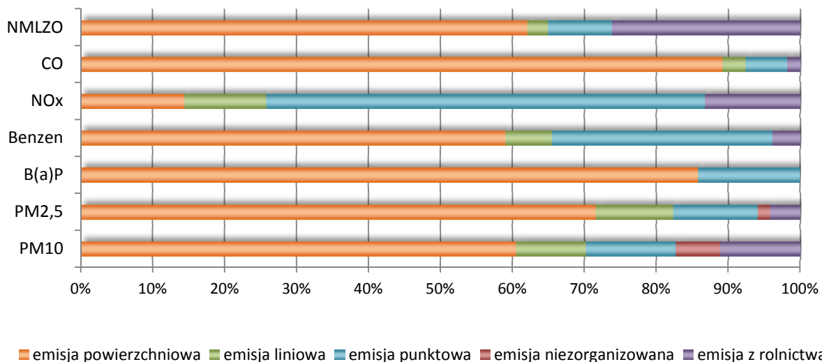
Rysunek 35. Udziół poszczególnych rodzajów źródeł w emisji analizowanych zanieczyszczeń na terenie strefy opolskiej w roku bazowym 2016 (źródło: opracowanie własne na podstawie bilansu emisji substancji dla roku 2016).
