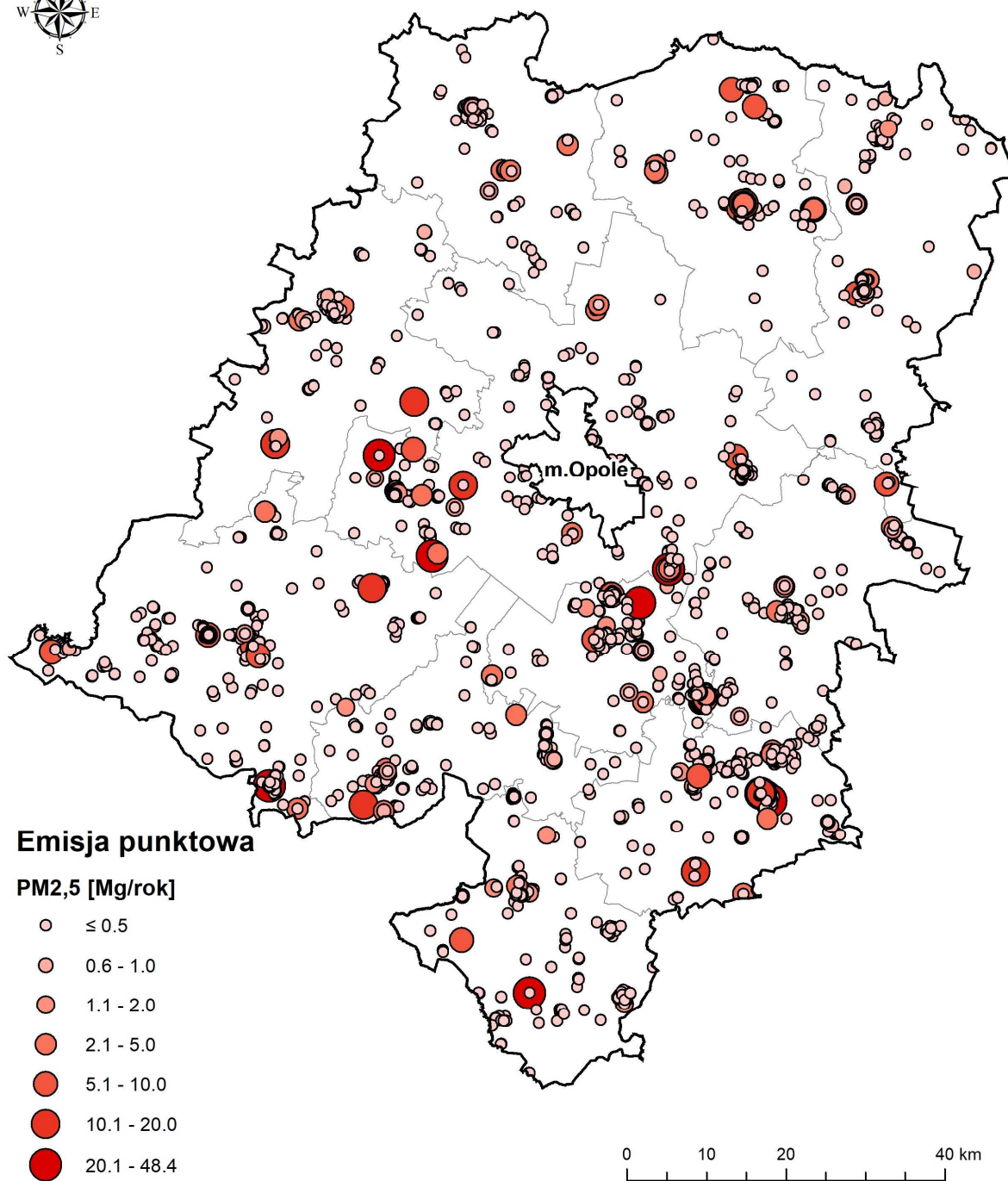
Rysunek 54. Rozkład emisji punktowej pyłu zawieszonego PM2,5 w roku 2016 na terenie strefy opolskiej (źródło: opracowanie własne).
