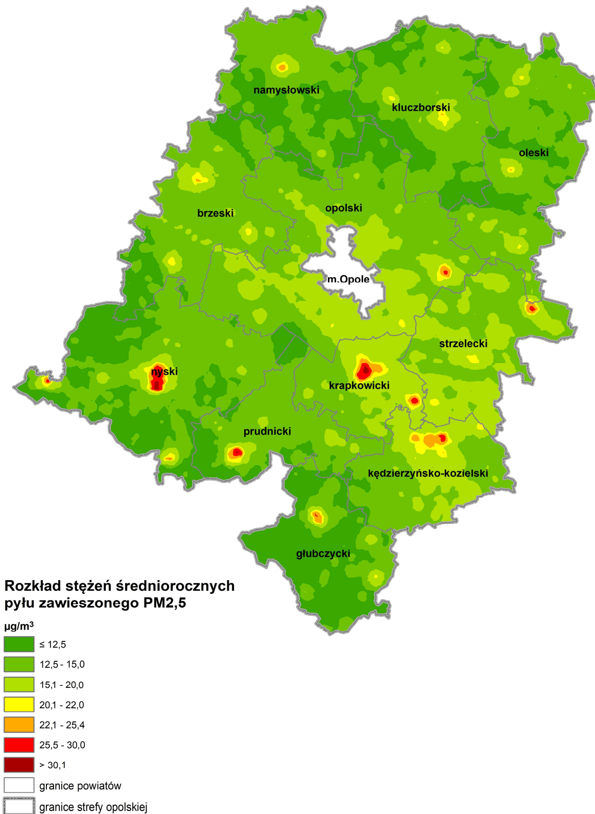
Rysunek 12. Rozkład stężeń średniorocznych pyłu zawieszonego PM 2,5 w strefie opolskiej w roku bazowym 2016 (źródło: opracowanie własne na podstawie wyników modelowania modelem CALPUFF dla 2016 r.).
