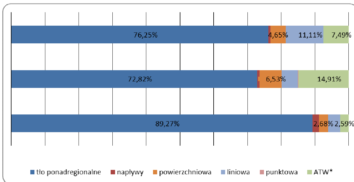
Rysunek 9. Średnie stężenia roczne benzenu według procentowego udziału źródeł na terenie strefy opolskiej i w powiatach kędzierzyńsko-kozielskim oraz krapkowskim w 2012 roku 4445
