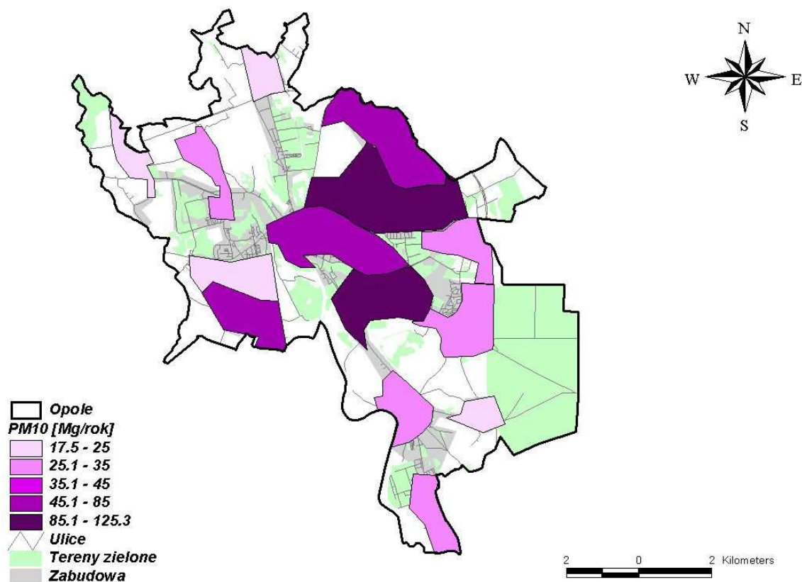
Rysunek 43 Emisja powierzchniowa pyłu zawieszonego PM_{10} w Opolu w 2005 r.
