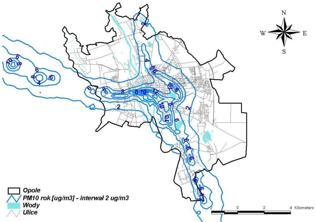
Rysunek 90 Rozkład stężeń pyłu zawieszonego \text{PM}_{10} o okresie uśredniania wyników pomiarów rok kalendarzowy pochodzących od emisji z transportu kolejowego na terenie Opola w 2005 r.
