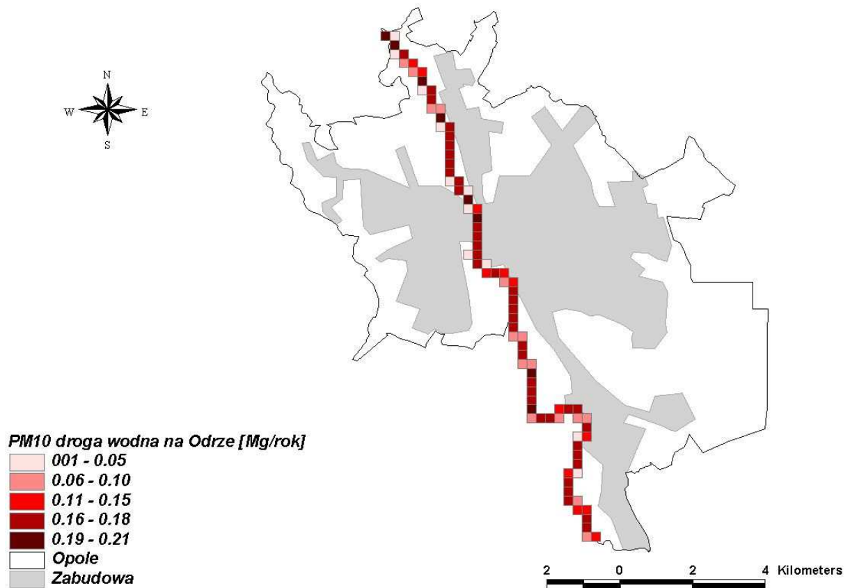
Rysunek 51 Emisja liniowa pyłu zawieszonego PM 10 , z transportu Odrą w Opolu w 2005 r.
