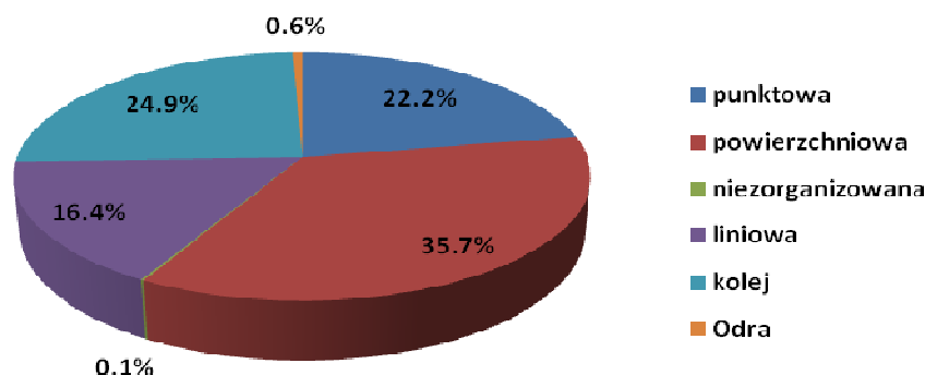
Emisja pyłu PM_{10} z terenu Opola
