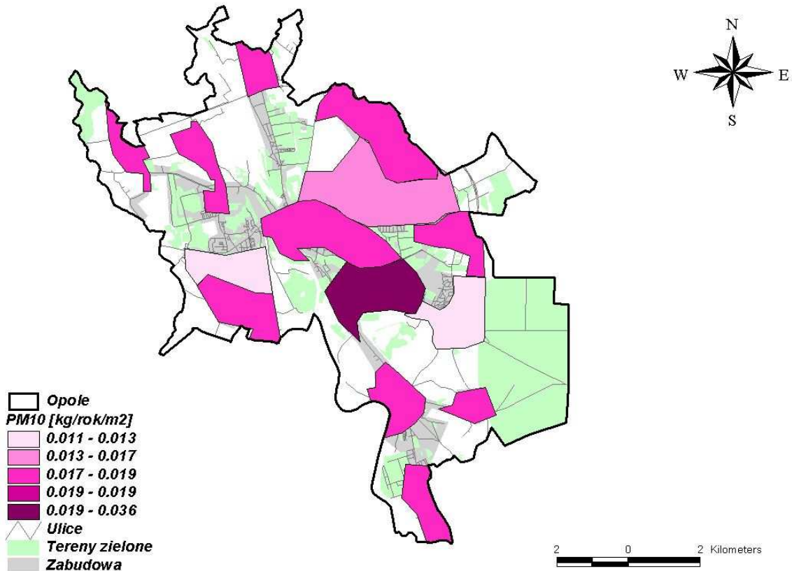
Rysunek 44 Gęstość emisji powierzchniowej pyłu zawieszonoego PM 10 na terenie Opola w 2005 roku
