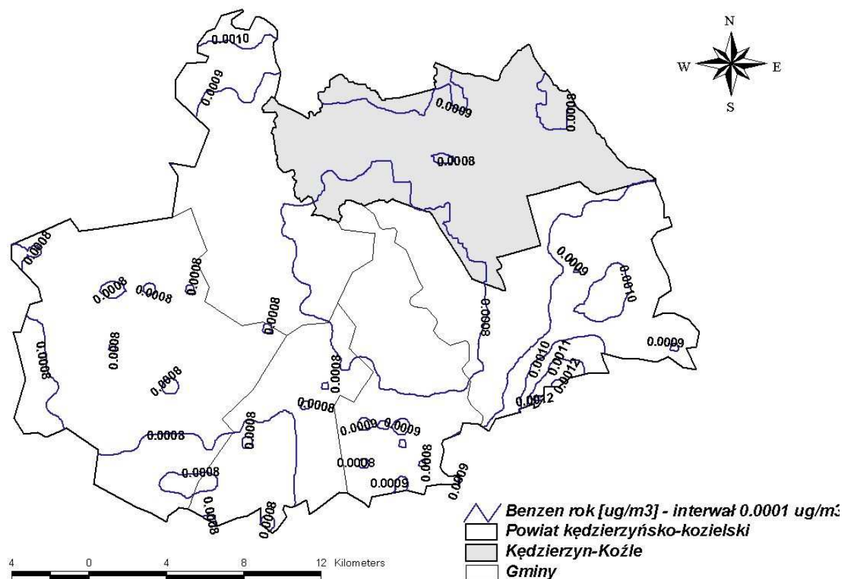
Rysunek 135 Stężenia benzenu o okresie uśredniania wyników pomiarów rok kalendarzowy w powiecie kędzierzyńsko-kozielskim pochodzące od emisji punktowej z pasa 30 km wokół powiatu w 2005 r.
