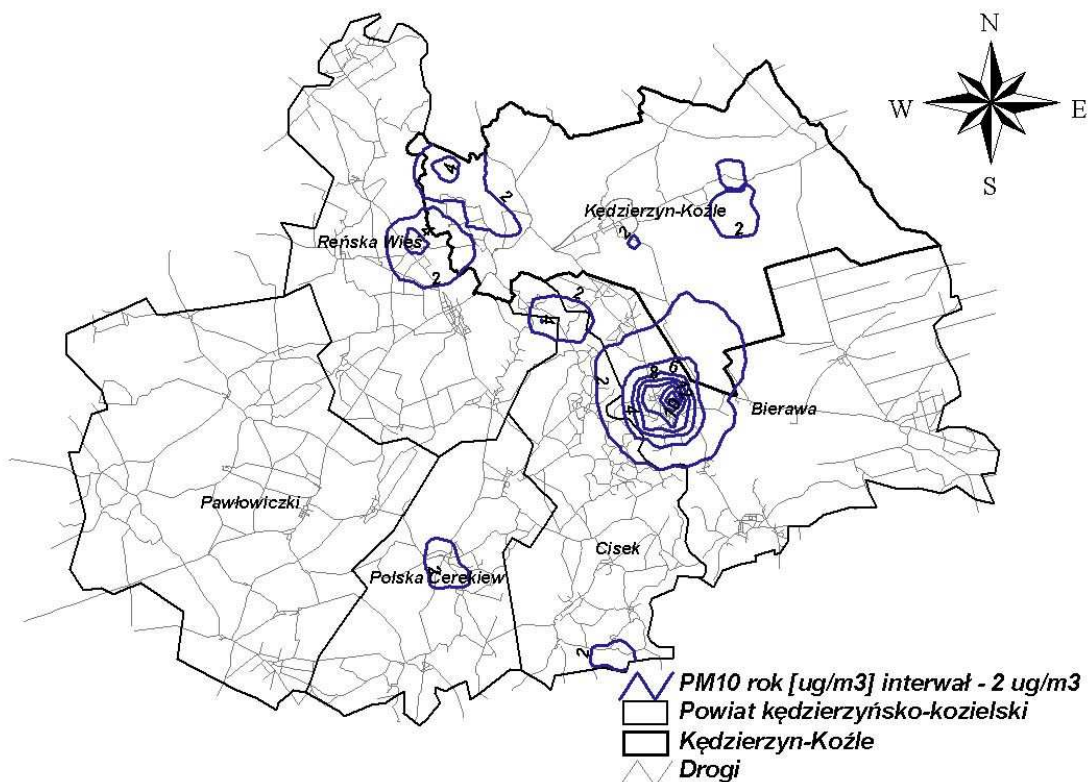
Rysunek 69 Rozkład stężeń pyłu zawieszonego \text{PM}_{10} o okresie uśredniania wyników pomiarów rok kalendarzowy pochodzących od emisji punktowej, na terenie powiatu kędzierzyńsko-kozielskiego w 2005 r.
