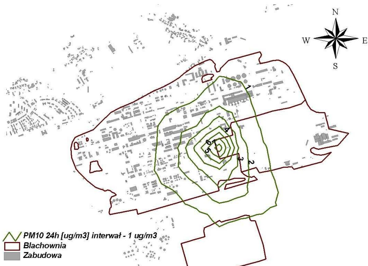
Rysunek 74 Stężenia pyłu zawieszonego PM_{10} o okresie uśredniania wyników pomiarów 24 godziny pochodzące z zakładu Famet S.A.
