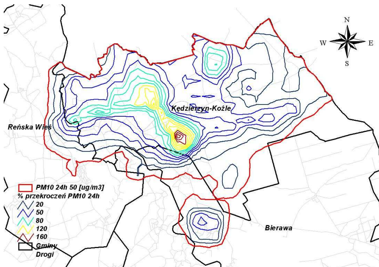
Rysunek 106 Wartość procentowa przekroczeń stężeń pyłu zawieszonego PM 10 o okresie uśredniania wyników pomiarów 24 godziny w Kędzierzynie-Koźlu, gminie Bierawa oraz gminie Reńska Wieś
