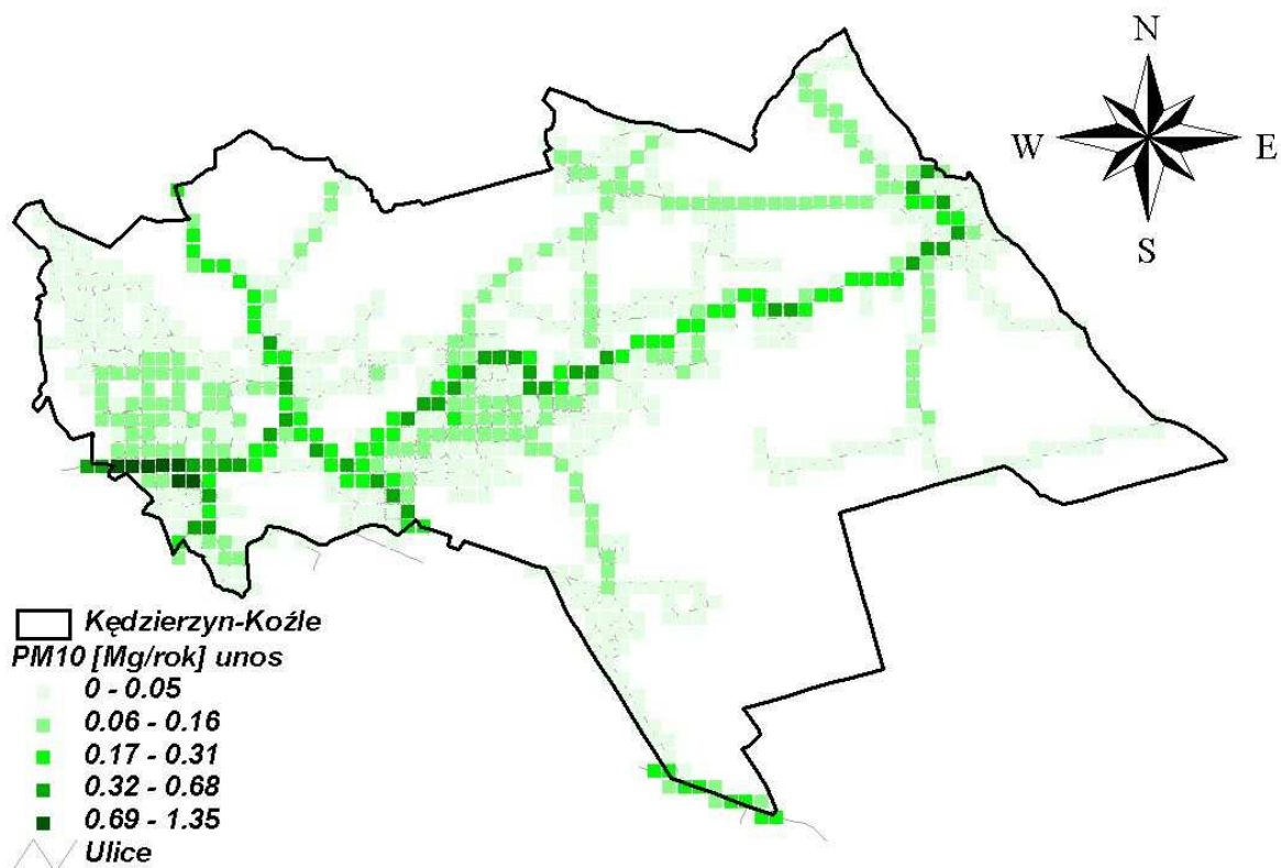
Rysunek 43 Emisja pyłu zawieszonego PM 10 z unosu, ze źródeł komunikacyjnych w Kędzierzynie-Koźlu w 2005 r.
