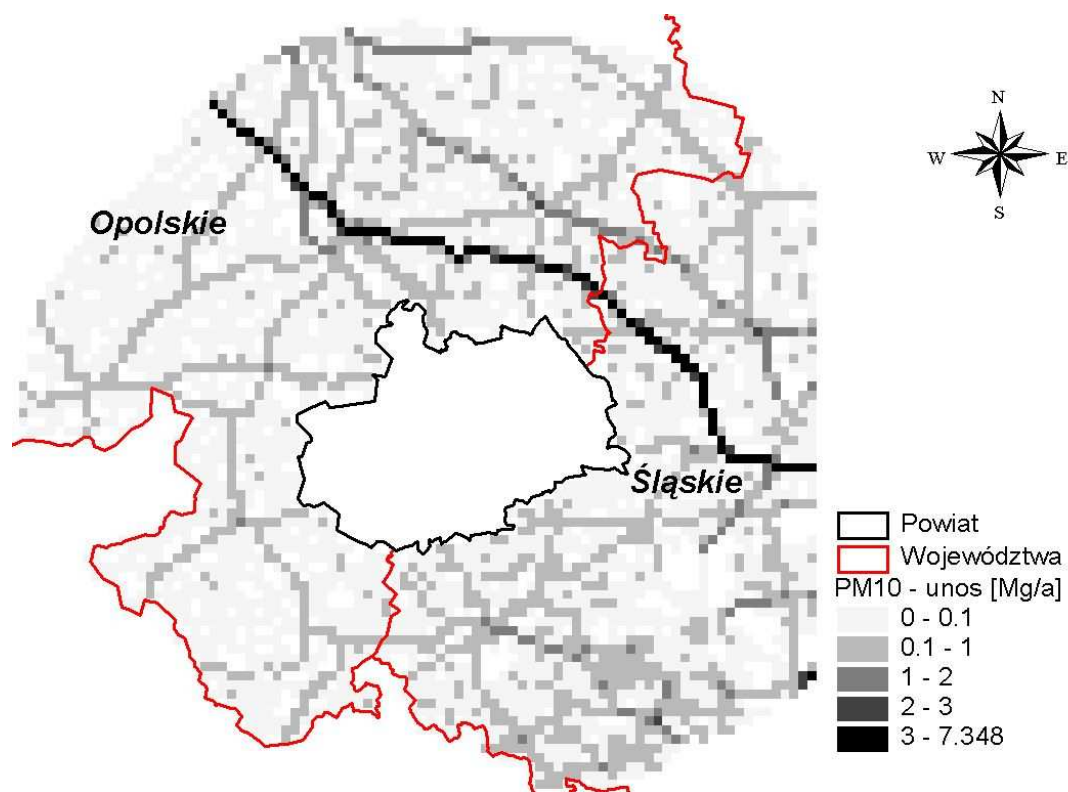
Rysunek 29 Emisja pyłu zawieszonoego PM 10 z unosu, ze źródeł liniowych zlokalizowanych w pasie 30 km wokół powiatu kędzierzyńsko-kozielskiego w 2005 r.
