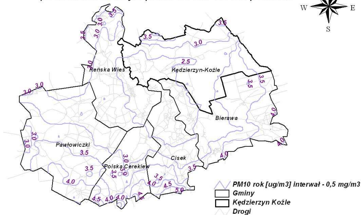
Rysunek 53 Stężenia pyłu zawieszonego PM 10 o okresie uśredniania wyników rok kalendarzowy, w powiecie kędzierzyńsko-kozielskim, pochodzące od emitorów powierzchniowych zlokalizowanych w pasie 30 km wokół powiatu w 2005 r.
