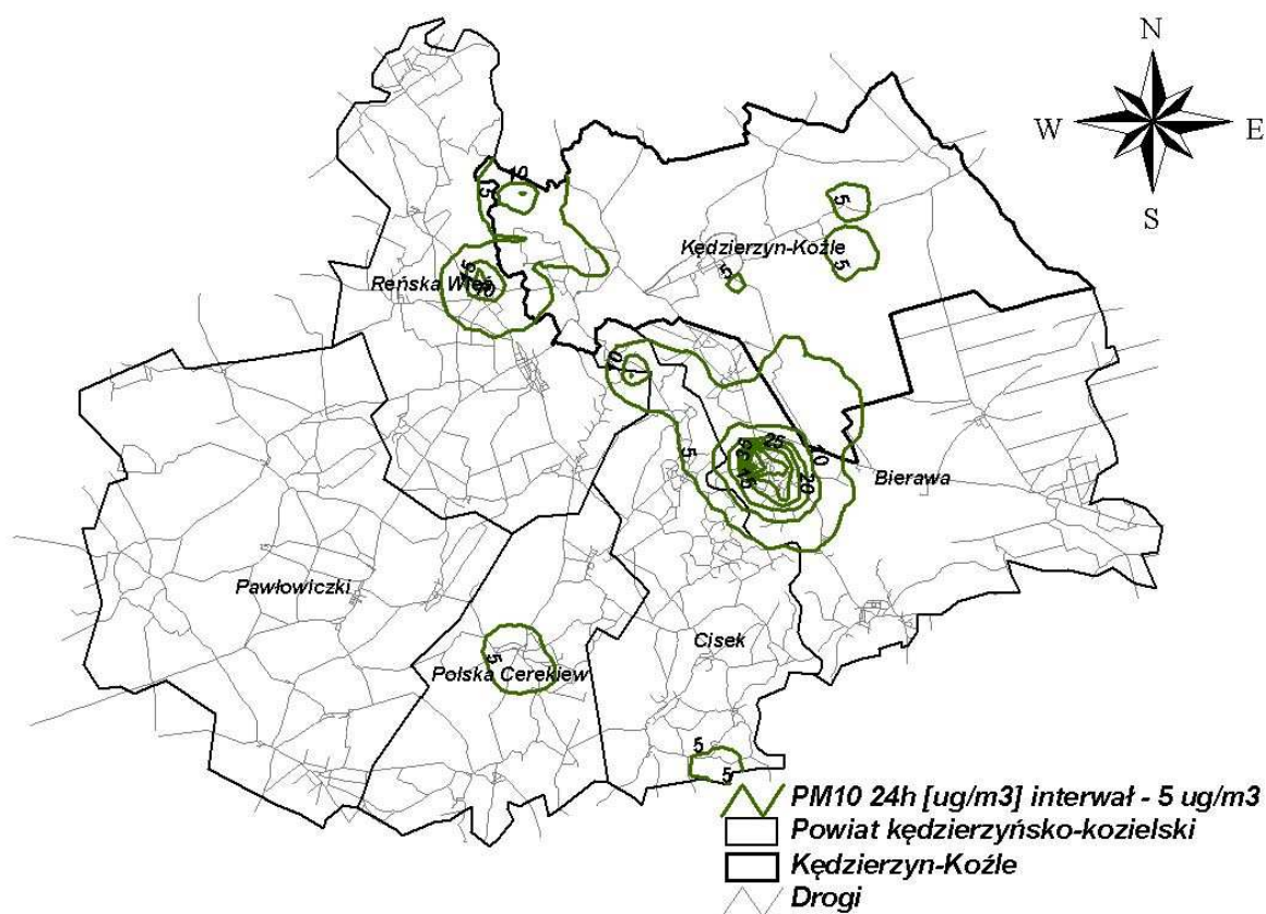
Rysunek 67 Rozkład stężeń pyłu zawieszonego PM_{10} o okresie uśredniania wyników pomiarów 24 godziny (36 max) pochodzących od emisji punktowej na terenie powiatu kędzierzyńsko-kozielskiego w 2005 r.
