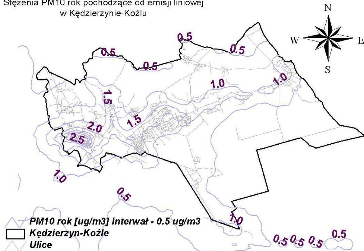
Rysunek 88 Rozkład stężeń pyłu zawieszonego PM 10 o okresie uśredniania wyników pomiarów - rok kalendarzowy pochodzących od emisji komunikacyjnej w Kędzierzynie-Koźlu w 2005 r.
