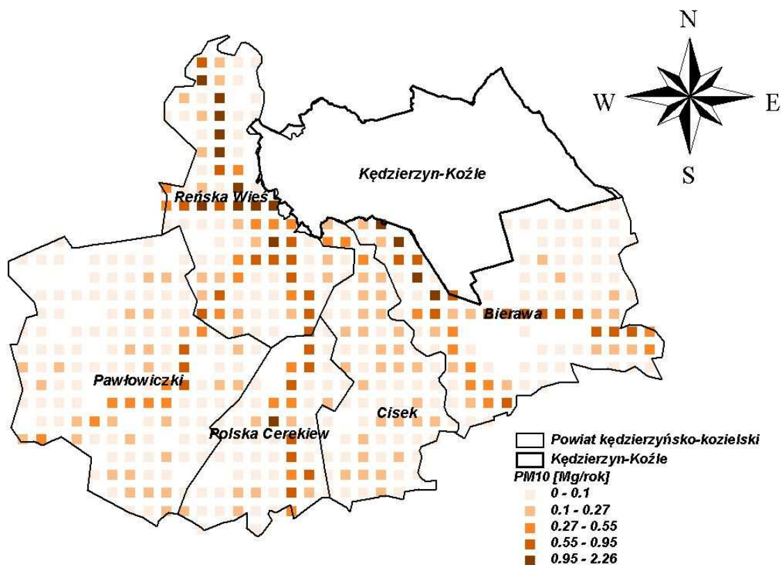
Rysunek 36 Emisja komunikacyjna pyłu zawieszonego PM 10 na drogach powiatu kędzierzyńsko-kozielskiego w 2005 r.
