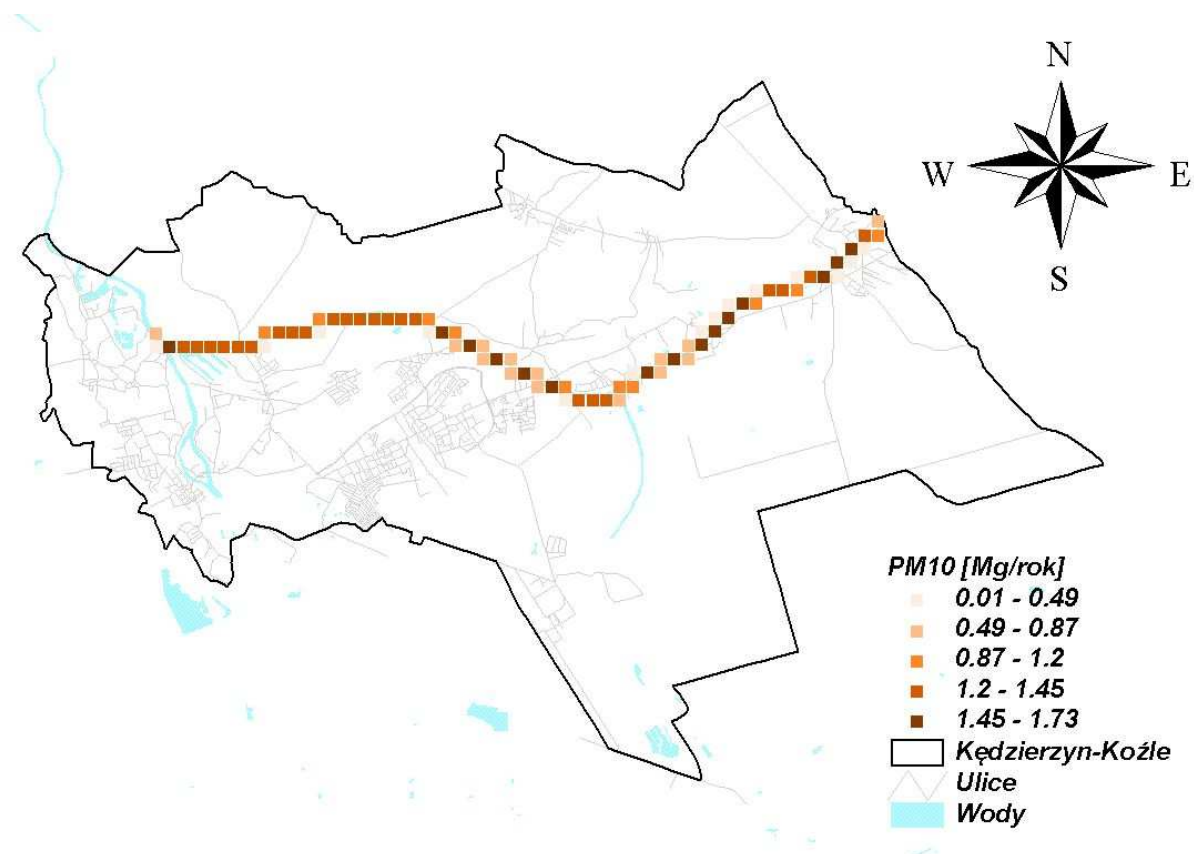
Rysunek 47 Emisja liniowa pyłu zawieszonego PM 10 z transportu Kanalem Gliwickim w Kędzierzynie-Koźlu w 2005 r.
