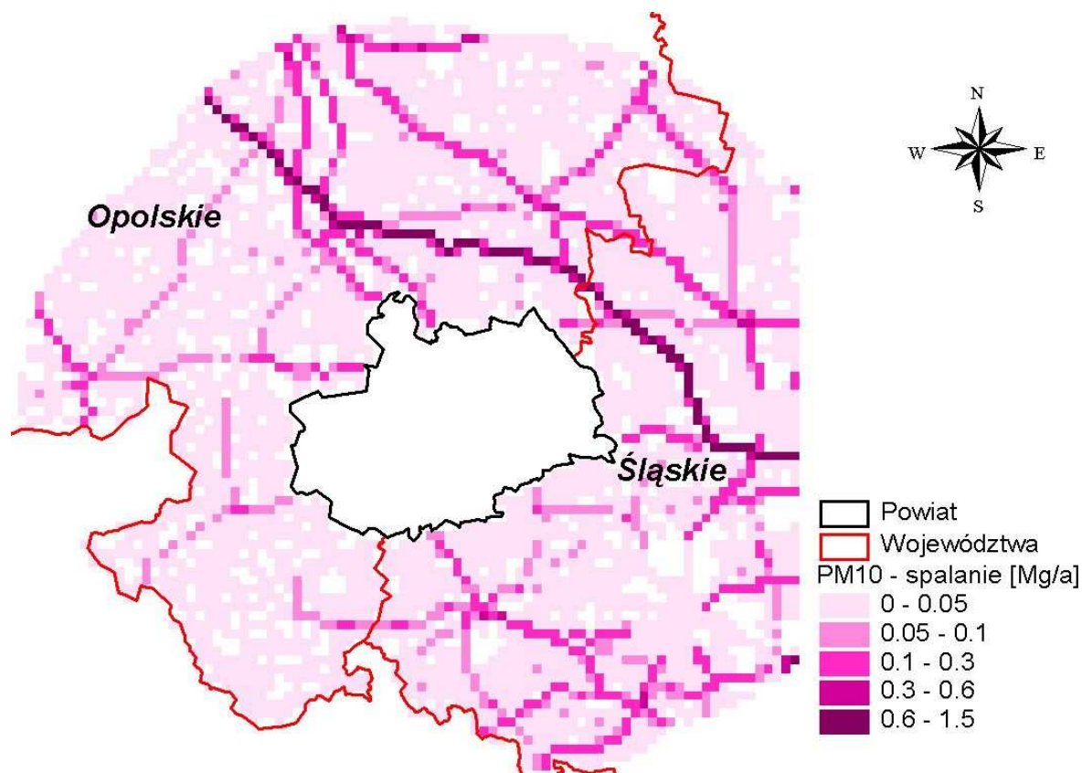
Rysunek 30 Emisja pyłu zawieszonoego PM 10 ze spalania, ze źródeł liniowych zlokalizowanych w pasie 30 km wokół powiatu kędzierzyńsko-kozielskiego w 2005 r.
