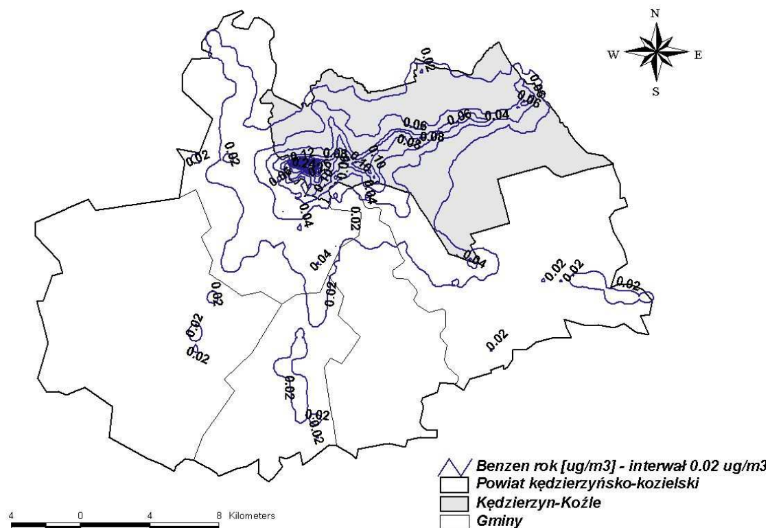
Rysunek 143 Stężenia benzenu o okresie uśredniania wyników pomiarów rok kalendarzowy w strefie kędzierzyńsko-kozielskiej pochodzące od emisji liniowej – komunikacyjnej w 2005 r.
