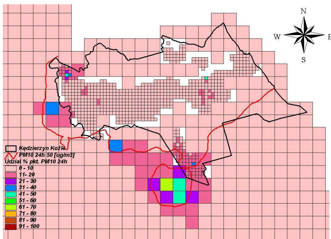
Rysunek 111 Udział procentowy emisji punktowej w imisji całkowitej pyłu zawieszonego PM 10 o okresie uśredniania wyników pomiarów 24 godziny w Kędzierzynie-Koźlu, gminie Bierawa oraz gminie Reńska
