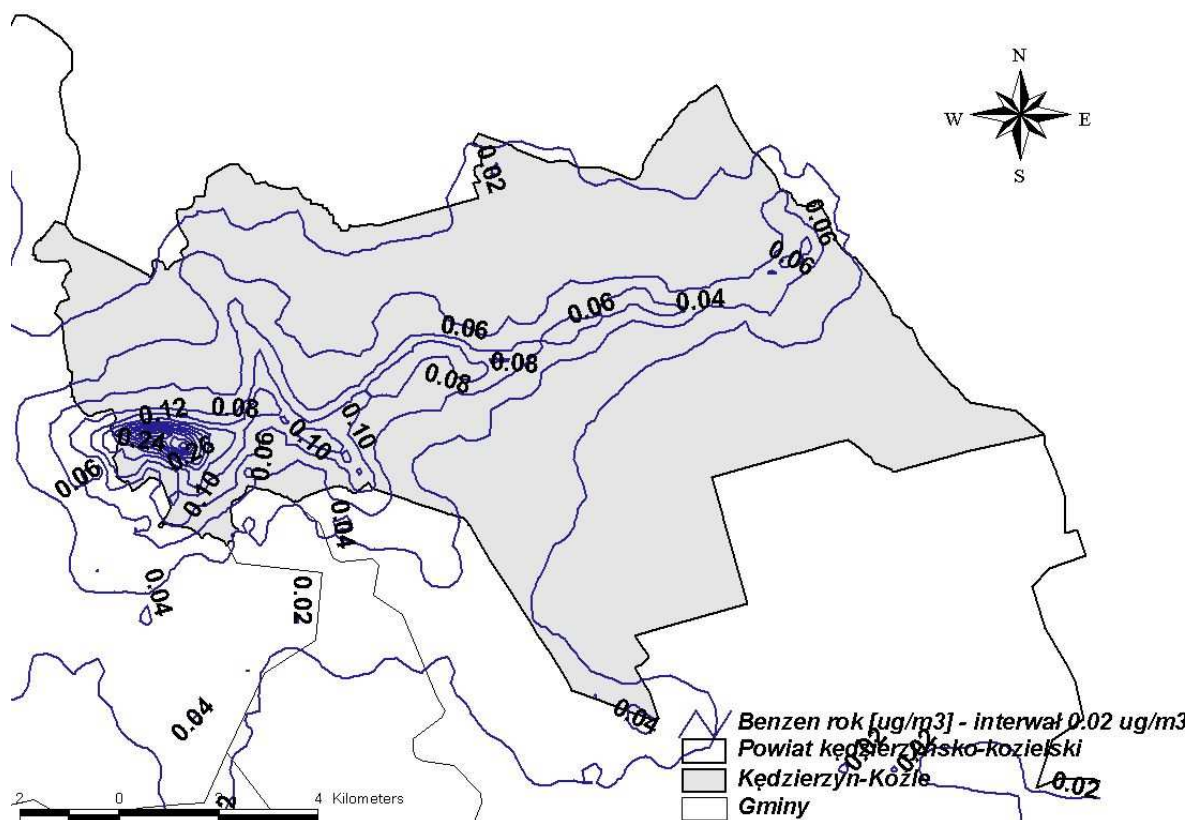
Rysunek 144 Stężenia benzenu o okresie uśredniania wyników pomiarów rok kalendarzowy w Kędzierzynie-Koźlu pochodzące od emisji liniowej – komunikacyjnej w 2005 r.
