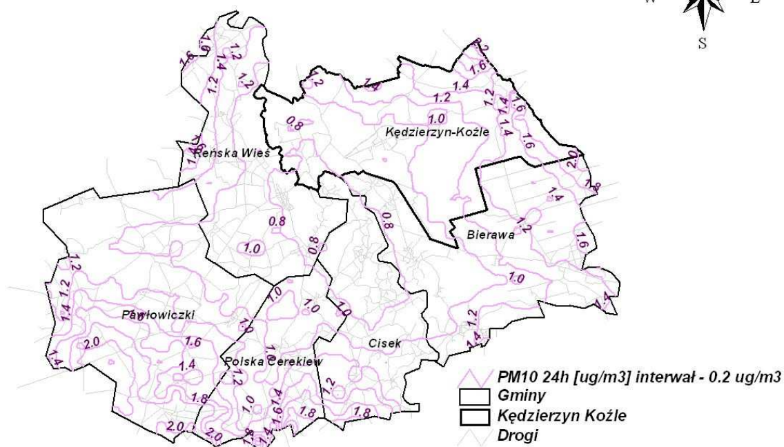
Rysunek 54 Stężenia pyłu zawieszonego PM 10 o okresie uśredniania wyników pomiarów 24 godziny w powiecie kędzierzyńsko-kozielskim pochodzące od emitorów liniowych zlokalizowanych w pasie 30 km od powiatu w 2005 r.
