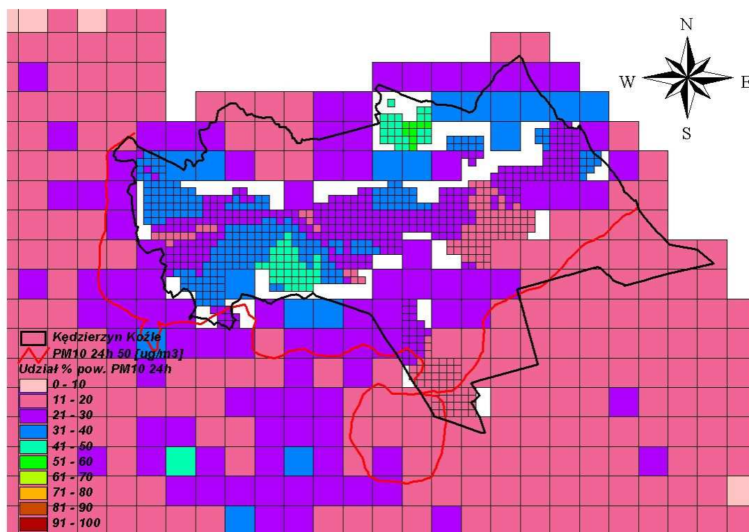
Rysunek 112 Udział procentowy emisji powierzchniowej w imisji całkowitej pyłu zawieszonego PM 10 o okresie uśredniania wyników pomiarów 24 godziny w Kędzierzynie-Koźlu, gminie Bierawa oraz gminie Reńska
