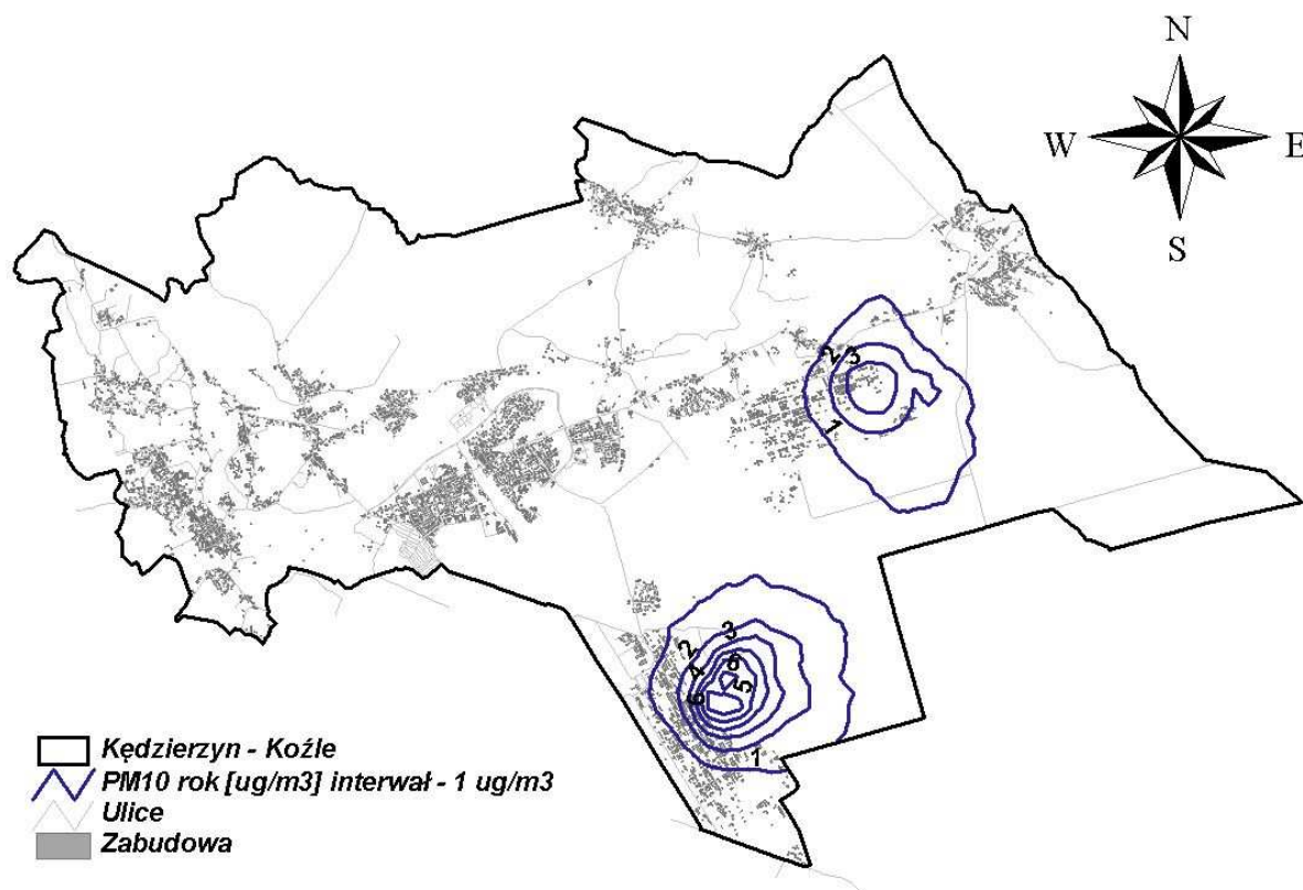
Rysunek 82 Stężenia pyłu zawieszonego PM 10 o okresie uśredniania wyników pomiarów rok kalendarzowy z emisji niezorganizowanej w Kędzierzynie-Koźlu w 2005 r.
