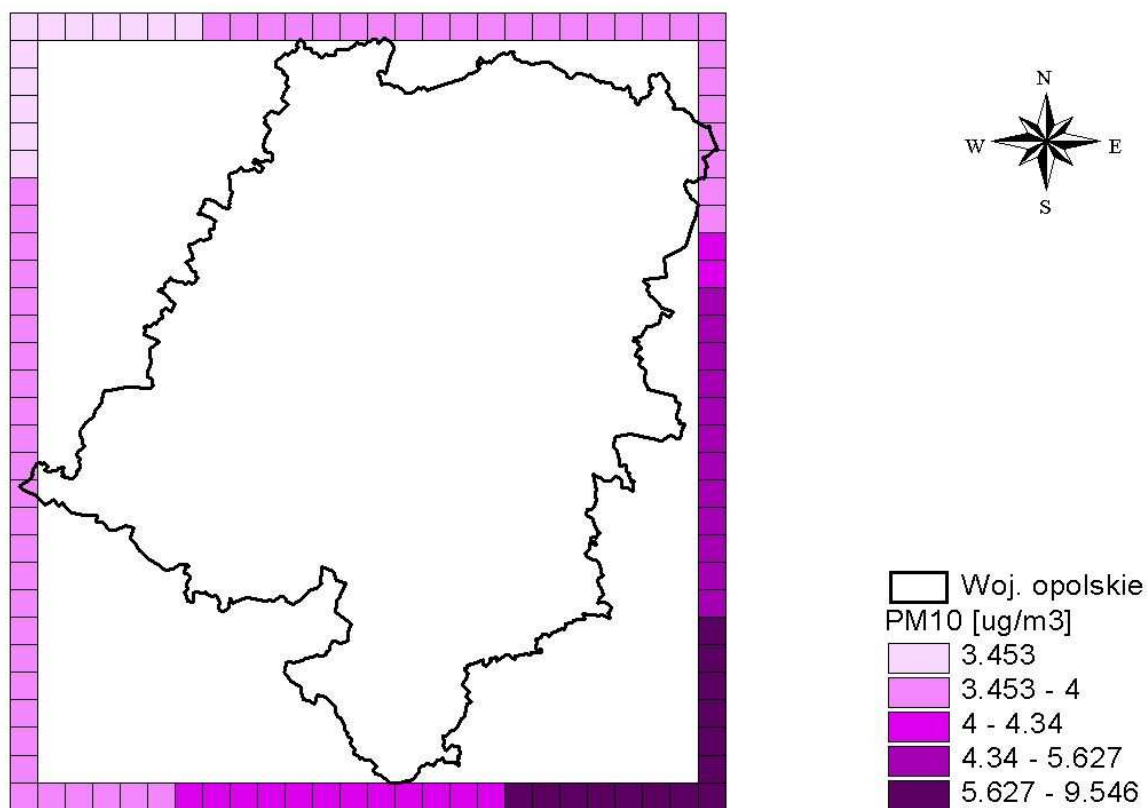
Rysunek 16 Warunki brzegowe dla \text{PM}_{10} pierwotnego dla obszaru województwa opolskiego
