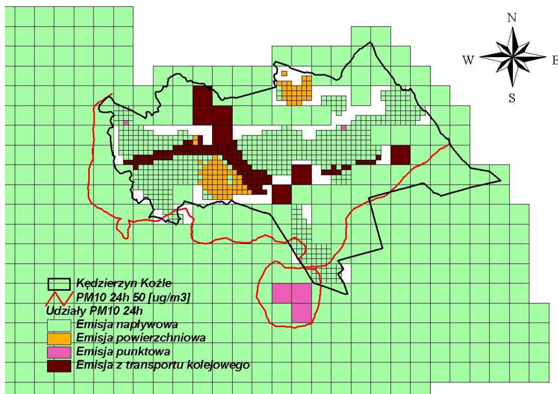
Rysunek 108 Większościowy udział poszczególnych typów emisji w imisji pyłu zawieszonego PM 10 o okresie uśredniania wyników pomiarów 24 godziny w Kędzierzynie-Koźlu, gminie Bierawa oraz gminie Reńska
