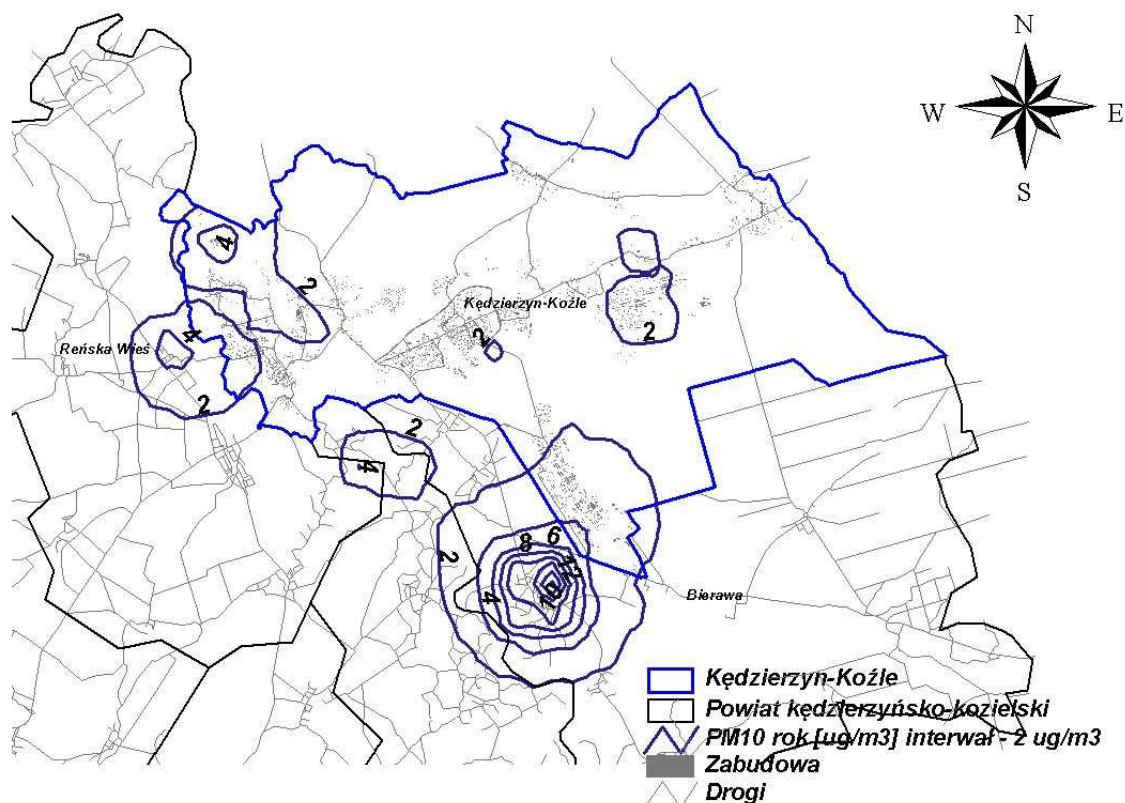
Rysunek 70 Rozkład stężeń pyłu zawieszonego \text{PM}_{10} o okresie uśredniania wyników pomiarów rok kalendarzowy pochodzących od emisji w Kędzierzynie-Koźlu w 2005 r.
