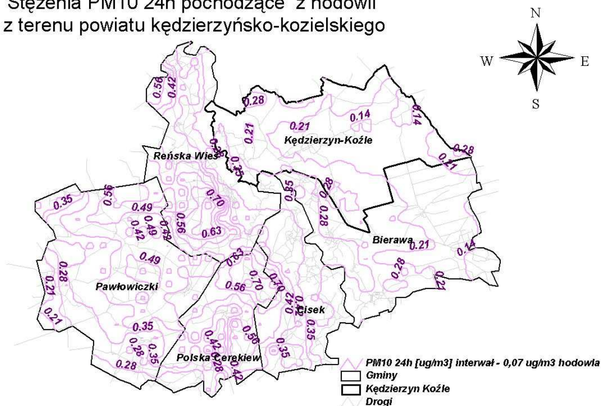
Rysunek 91 Rozkład stężeń pyłu zawieszonego PM 10 o okresie uśredniania wyników pomiarów 24 godziny pochodzących z hodowli na terenie powiatu kędzierzyńsko-kozielskiego w 2005 r.
