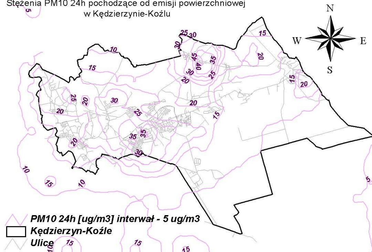
Rysunek 78 Rozkład stężeń pyłu zawieszonego PM 10 o okresie uśredniania wyników pomiarów 24 godziny (36max) pochodzących od emisji powierzchniowej w Kędzierzynie-Koźlu w 2005 r.
