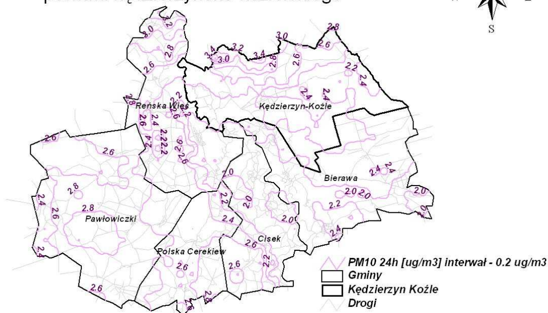
Rysunek 50 Stężenia pyłu zawieszonego PM 10 o okresie uśredniania wyników 24 godziny, w powiecie kędzierzyńsko-kozielskim pochodzące od emitorów punktowych zlokalizowanych w pasie 30 km wokół powiatu, w 2005 r.
