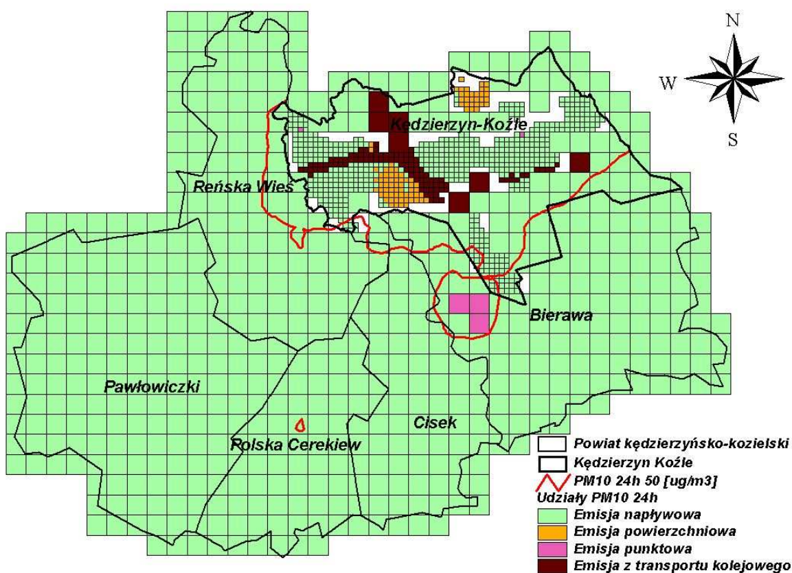
Rysunek 95 Udziały poszczególnych typów emisji w stężeniach pyłu zawieszonego PM_{10} o okresie uśredniania wyników pomiarów 24 godziny na terenie powiatu kędzierzyńsko-kozielskiego w 2005 r.
