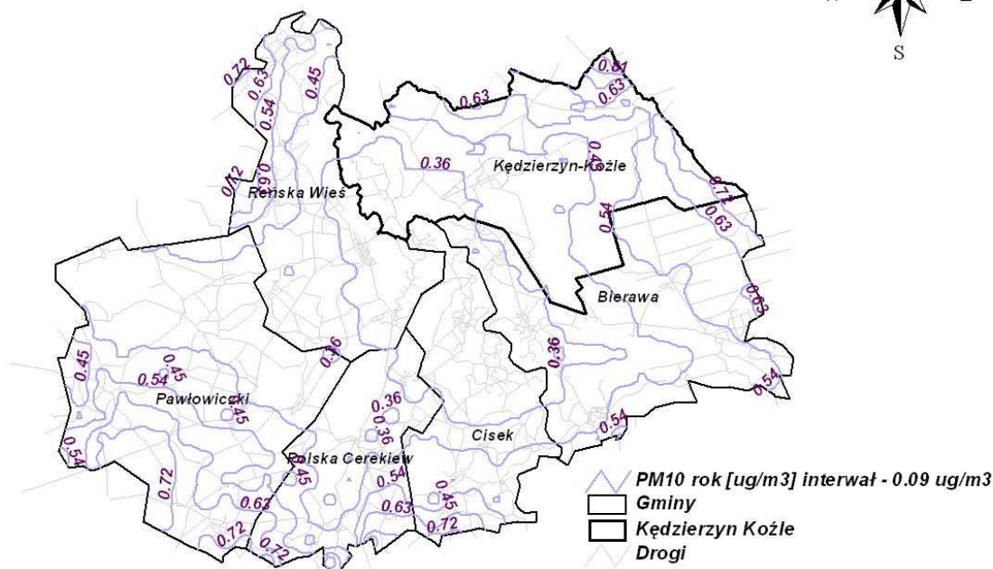
Rysunek 55 Stężenia pyłu zawieszonego PM 10 o okresie uśredniania wyników pomiarów rok kalendarzowy w powiecie kędzierzyńsko-kozielskim, pochodzące od emitorów liniowych zlokalizowanych w pasie 30 km wokół powiatu, w 2005 r.
