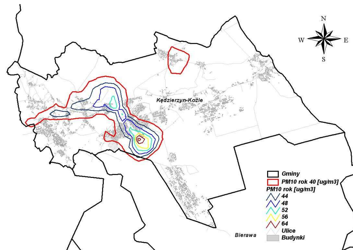
Rysunek 105 Obszary przekroczeń poziomu dopuszczalnego stężenia pyłu zawieszonego PM 10 o okresie uśredniania wyników pomiarów rok kalendarzowy w Kędzierzynie-Koźle
