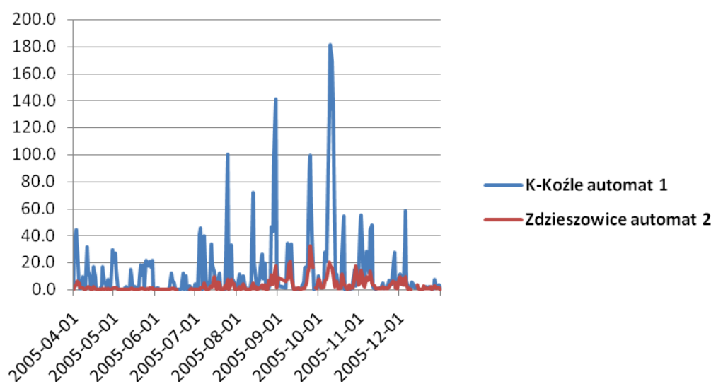
Rysunek 119 Stężenia benzenu na stacjach pomiarów automatycznych Kędzierzynie-Koźlu i w Zdieszowicach w 2005 r.
