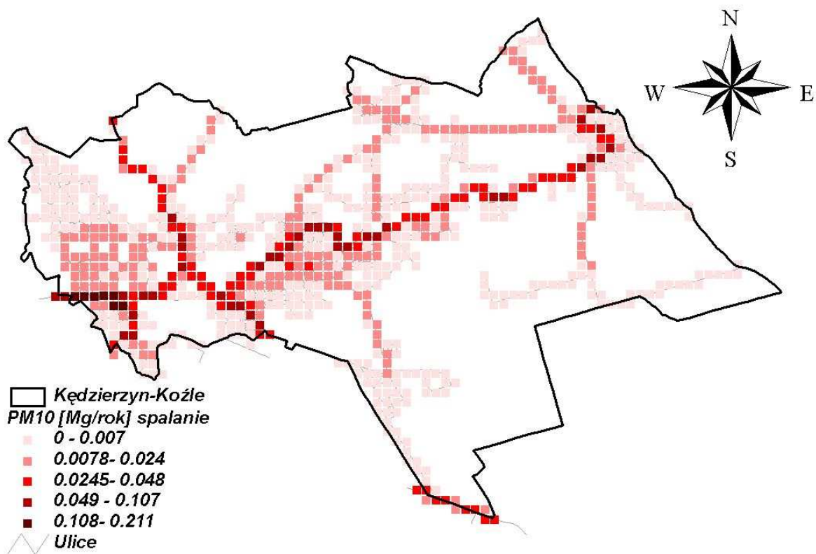
Rysunek 44 Emisja pyłu zawieszonego PM 10 ze spalania paliw, ze źródeł komunikacyjnych w Kędzierzynie-Koźlu w 2005 r.
