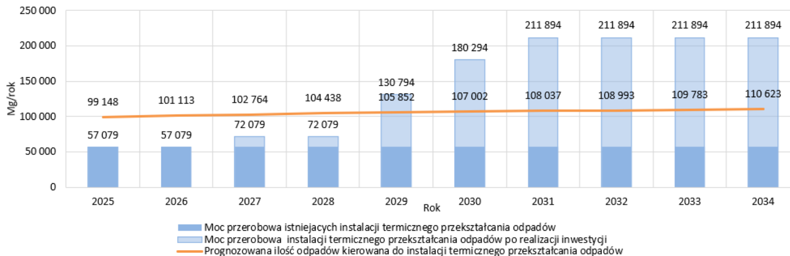
Rysunek 51. Bilans przepustowości instalacji do termicznego przekształcania odpadów komunalnych na terenie województwa opolskiego przed i po realizacji inwestycji
