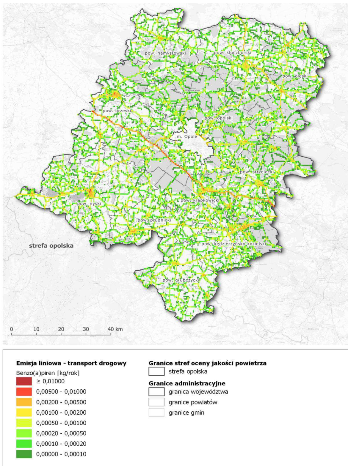
Rysunek 84. Lokalizacja i wielkość emisji benzo(a)pirenu z sektora transportu drogowego w strefie opolskiej w roku bazowym 2018 256
