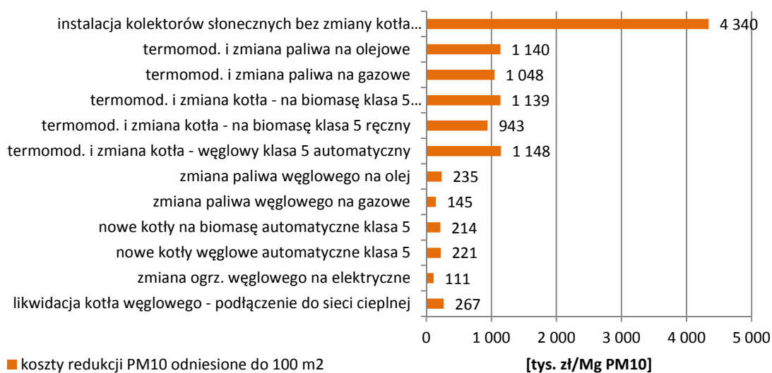
Rysunek 87. Porównanie wskaźników kosztowych redukcji pyłu zawieszonego PM10 z indywidualnych systemów grzewczych (źródło: opracowanie własne na podstawie aktualnych cen w 2016 roku).
