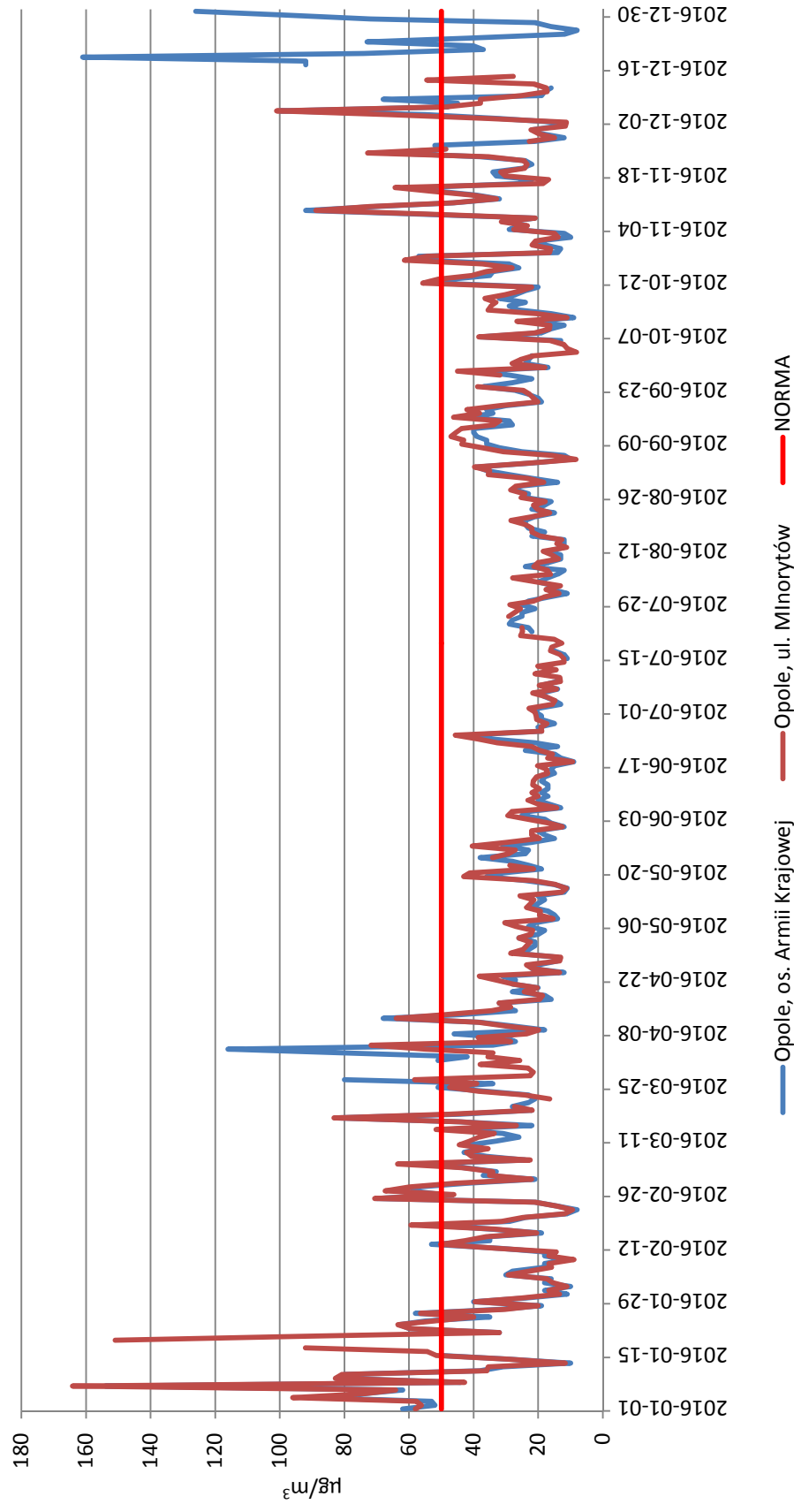
Rysunek 18. Przebieg zmienności stężeń 24-godzinnych pyłu zawieszonego PM10 w strefie miasto Opole w 2016 r. (źródło: dane WIOŚ).
