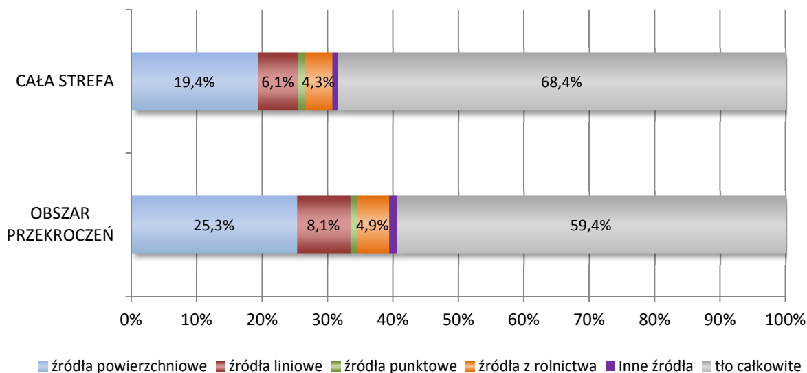
Rysunek 28. Średnie udziały źródeł emisji w stężeniach rocznych obliczone na obszarze całej strefy miasto Opole oraz na obszarze przekroczeń stężeń 24-godzinnych pyłu zawieszonego PM10 w roku bazowym 2016 (źródło: obliczenia własne na podstawie wyników modelowania modelem CALPUFF dla roku 2016).
