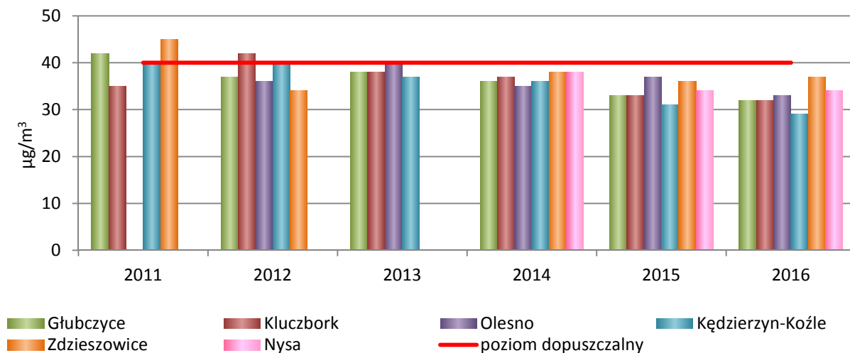
Rysunek 21. Wyniki pomiarów średniorocznych pyłu zawieszonego PM10 w latach 2011-2016 na terenie strefy opolskiej (źródło: opracowanie własne na podstawie danych WIOŚ).
