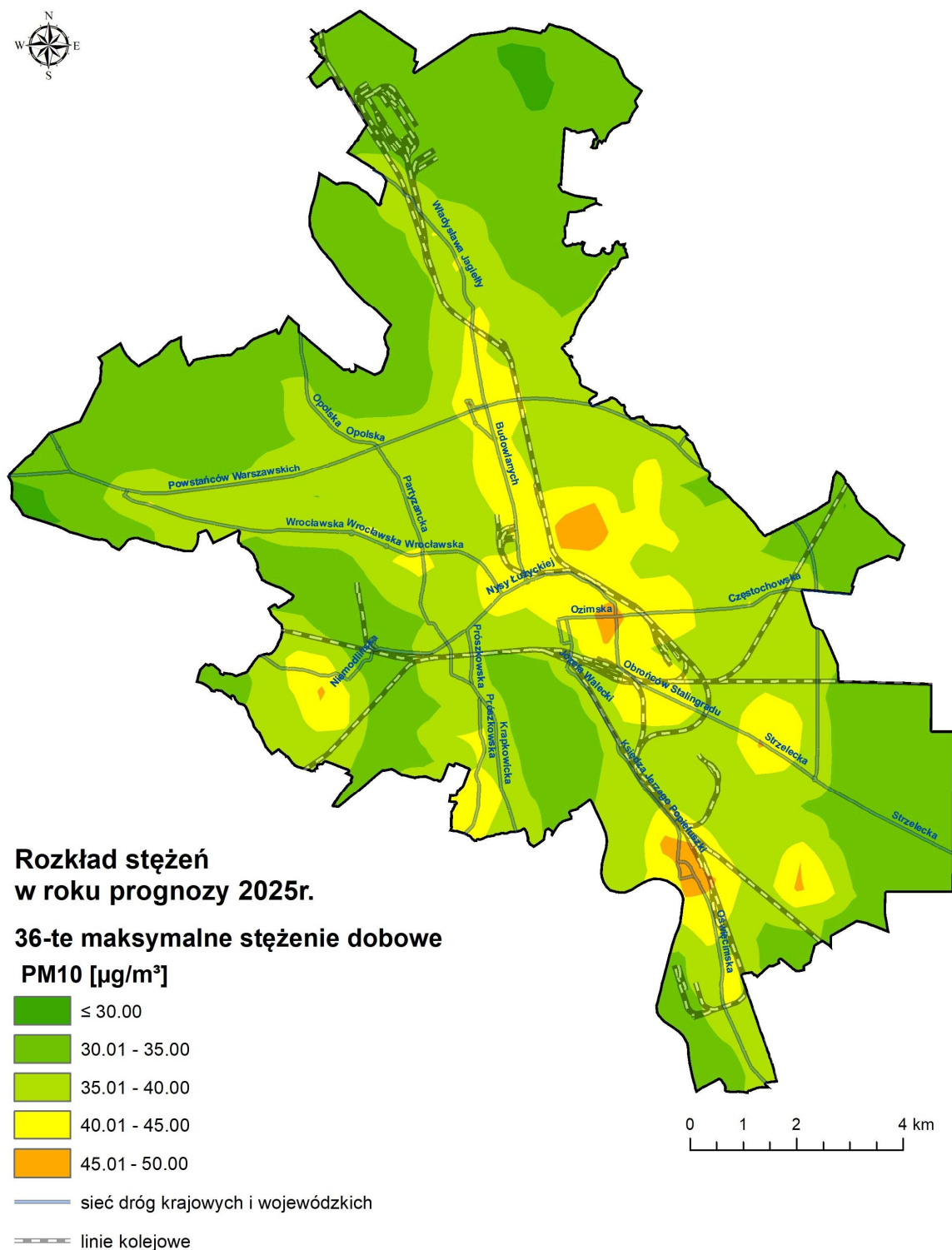
Rysunek 37. Rozkład stężeń 24-godzinnych wyznaczonych jako 36-te maksymalne stężenie pyłu zawieszonego PM10 w strefie miasto Opole w roku prognozy 2025 (źródło: opracowanie własne na podstawie wyników modelowania modelem CALPUFF dla 2016 r.).
