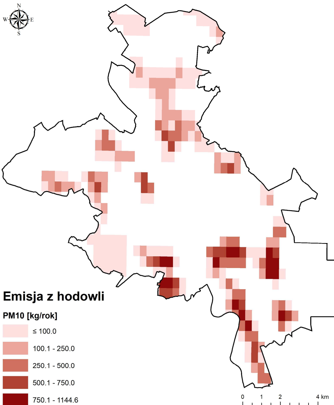
Rysunek 78. Rozkład emisji z hodowli pyłu zawieszonego PM10 w roku 2016 na terenie strefy miasto Opole (źródło: opracowanie własne).
