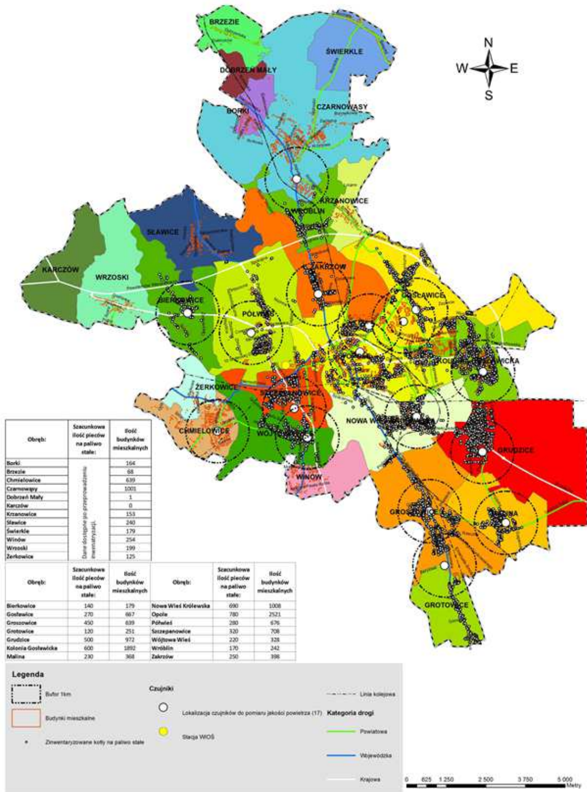
Rysunek 58. Lokalizacja instalacji na paliwo stałe na terenie strefy miasto Opole (źródło: http://www.niskaemisjaopole.pl/monitoring-wspomagajacy-ocene-jakosci-powietrza-w-miescie-opolu-juz-dziala/r6e )
