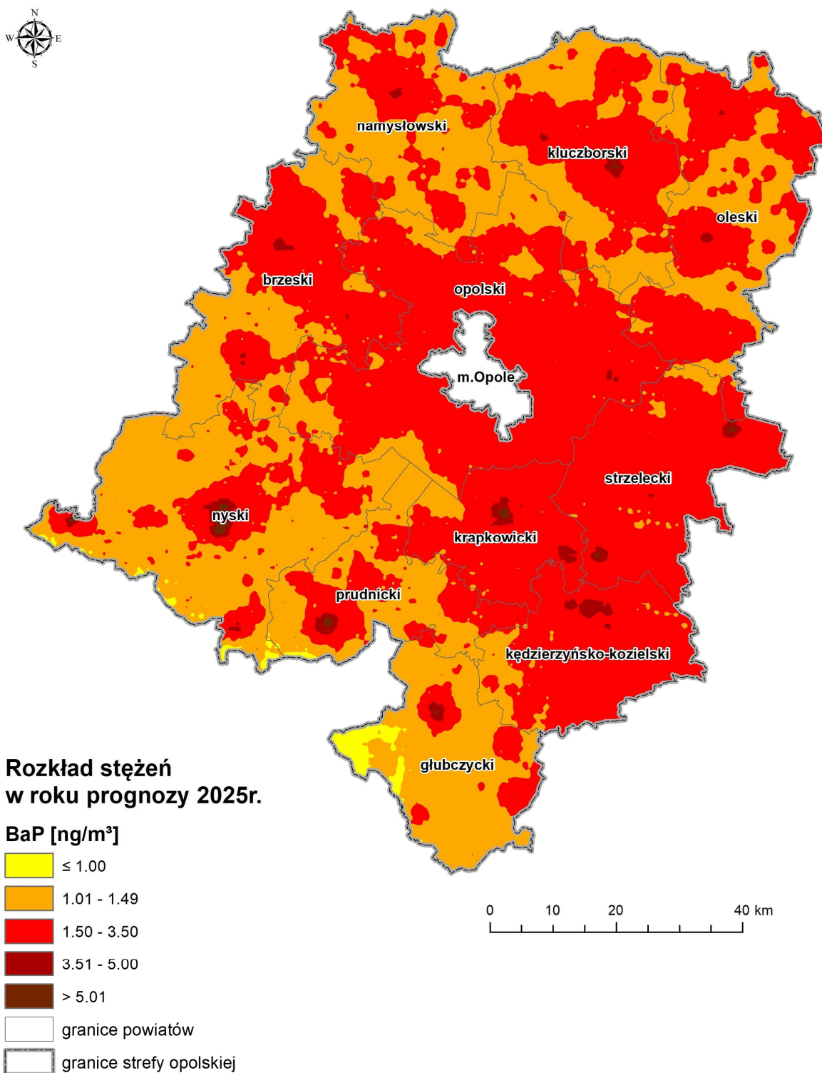
Rysunek 44. Rozkład stężeń średniorocznych benzo(a)pirenu w strefie opolskiej w roku prognozy 2025 (źródło: opracowanie własne na podstawie wyników modelowania modelem CALPUFF dla 2016 r.).
