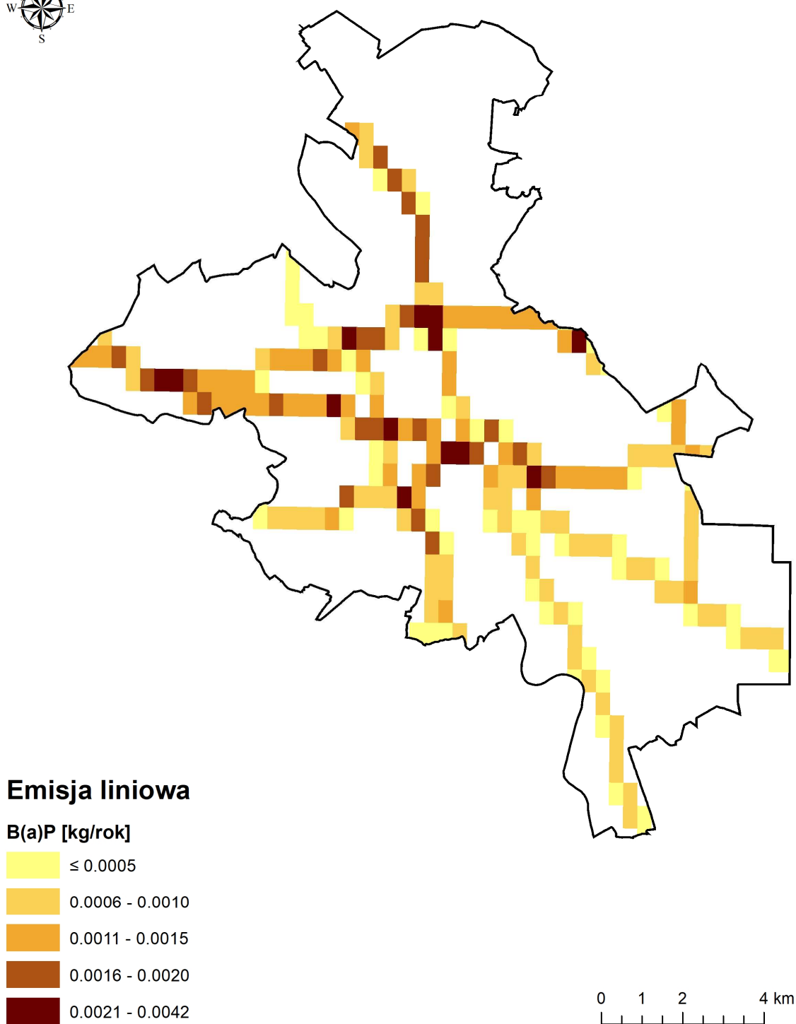
Rysunek 66. Rozkład emisji liniowej benzo(a)pirenu z dróg krajowych i wojewódzkich w roku 2016 na terenie strefy miasto Opole (źródło: opracowanie własne).
