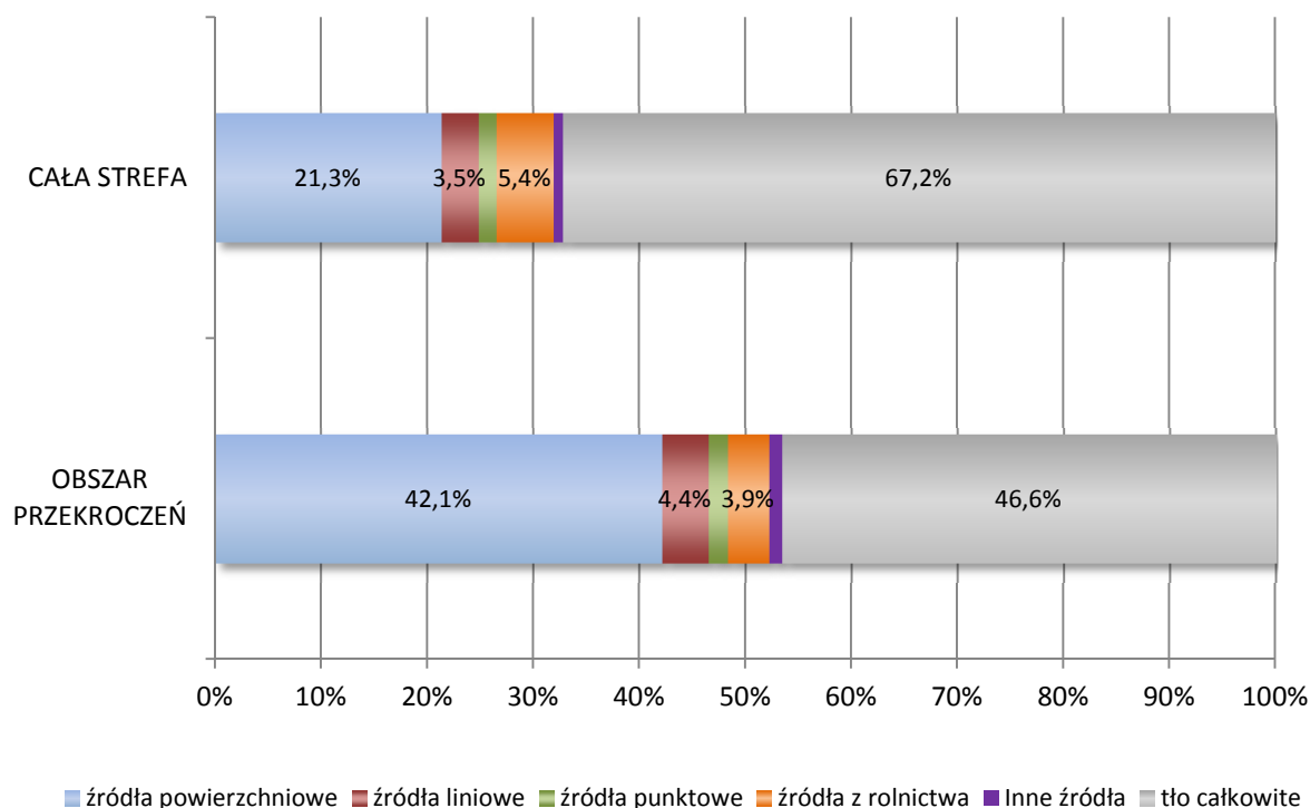
Rysunek 30. Średnie udziały źródeł emisji w stężeniach rocznych obliczone na obszarze całej strefy opolskiej oraz na obszarze przekroczeń stężeń 24-godzinnych pyłu zawieszonego PM10 w roku bazowym 2016 (źródło: na podstawie wyników modelowania matematycznego modelem CALPUFF).
