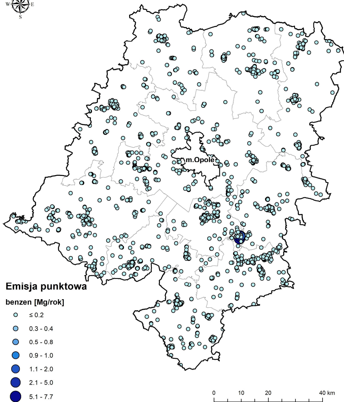
Rysunek 56. Rozkład emisji punktowej benzenu w roku 2016 na terenie strefy opolskiej (źródło: opracowanie własne).
