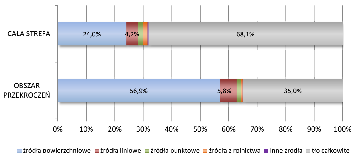
Rysunek 31. Średnie udziały źródeł emisji w stężeniach rocznych obliczone na obszarze całej strefy opolskiej oraz na obszarze przekroczeń stężeń średniorocznych pyłu zawieszonego PM 2,5 w roku bazowym 2016 (źródło: obliczenia własne na podstawie wyników modelowania modelem CALPUFF dla roku 2016.)
