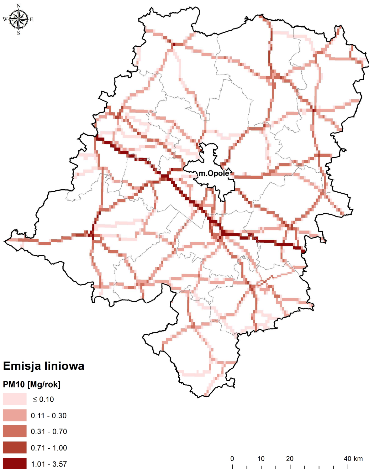
Rysunek 69. Rozkład emisji liniowej pyłu zawieszonego PM10 z dróg krajowych i wojewódzkich w roku 2016 na terenie strefy opolskiej (źródło: opracowanie własne).
