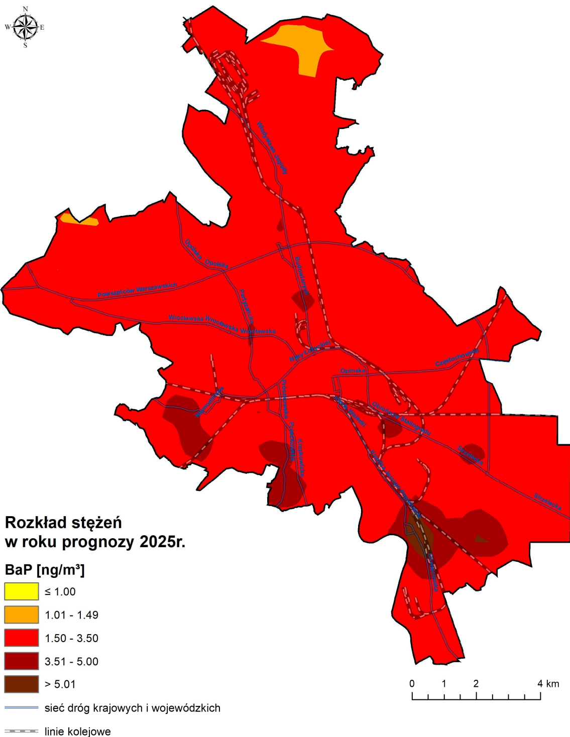
Rysunek 39. Rozkład stężeń średniorocznych benzo(a)pirenu w strefie miasto Opole w roku prognozy 2025 (źródło: opracowanie własne na podstawie wyników modelowania modelem CALPUFF dla 2016 r.).
