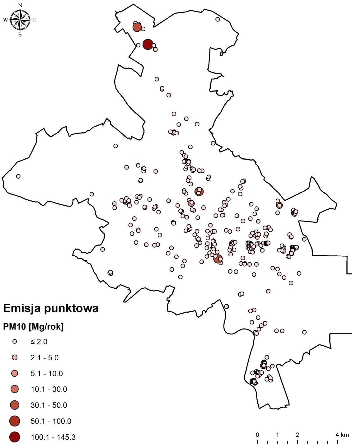
Rysunek 51. Rozkład emisji punktowej pyłu zawieszonego PM10 w roku 2016 na terenie strefy miasto Opole (źródło: opracowanie własne).
