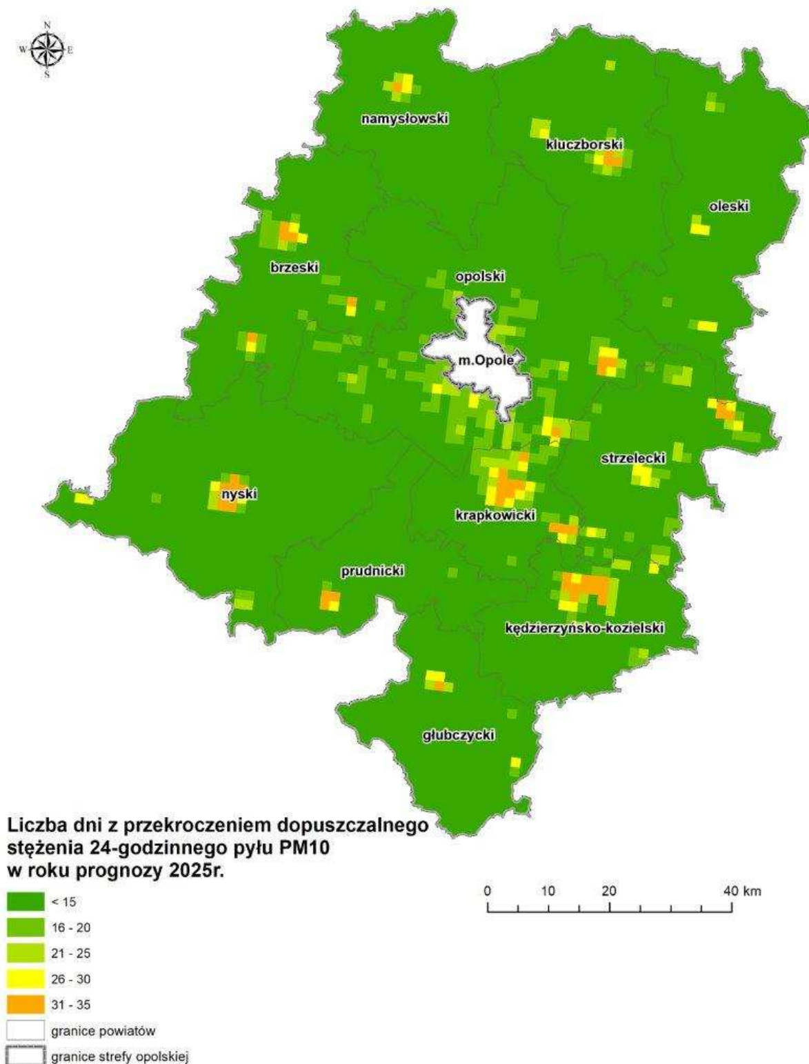
Rysunek 42. Liczba dni z przekroczeniem dopuszczalnego stężenia 24-godzinnego pyłu zawieszzonego PM10 w strefie opolskiej w roku prognozy 2025 (źródło: opracowanie własne na podstawie wyników modelowania modelem CALPUFF dla 2016 r.).
