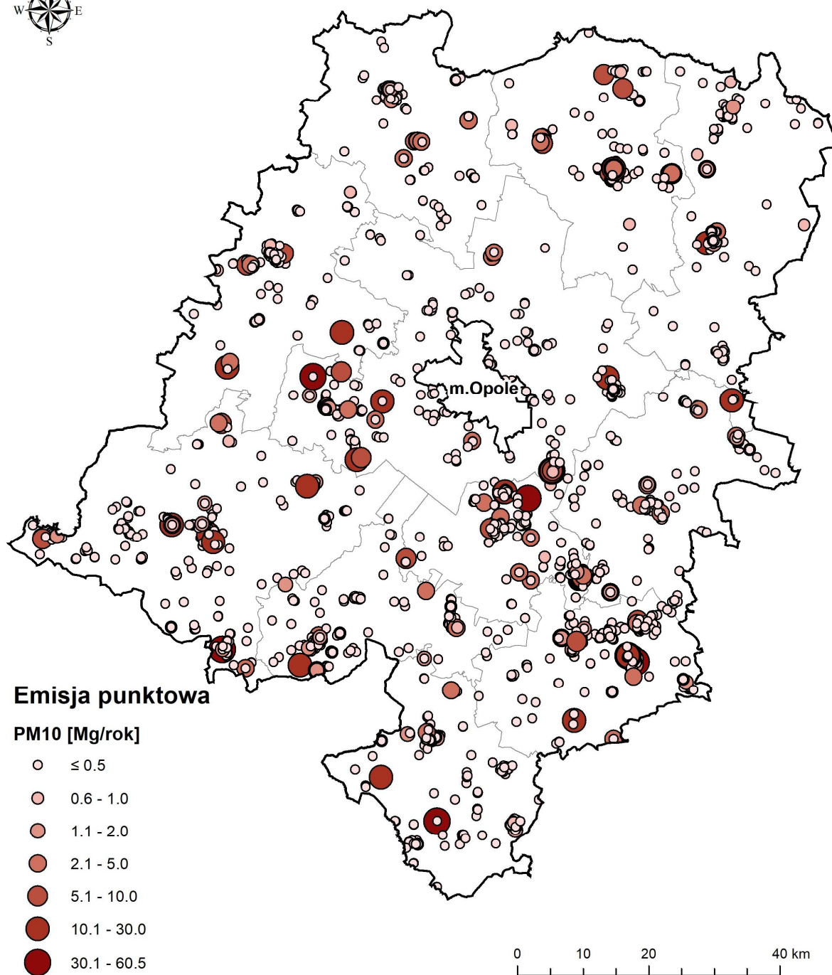
Rysunek 53. Rozkład emisji punktowej pyłu zawieszono PM10 w roku 2016 na terenie strefy opolskiej (źródło: opracowanie własne).
