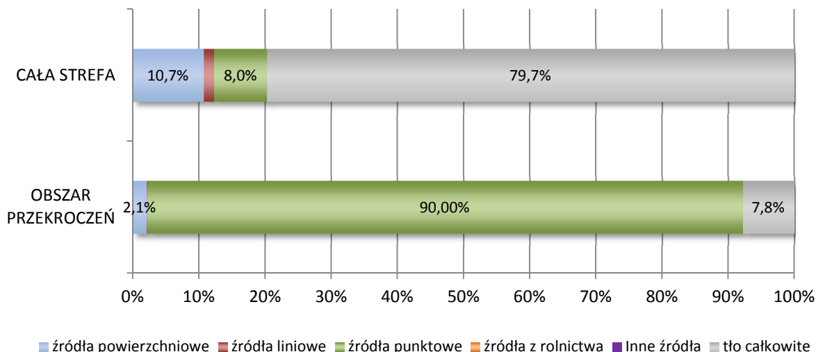
Rysunek 33. Średnie stężenia roczne w podziale na rodzaje źródeł emisji obliczone w na obszarze całej strefy opolskiej oraz na obszarze przekroczeń stężeń średniorocznych benzenu w roku bazowym 2016 (źródło: obliczenia własne na podstawie wyników modelowania modelem CALPUFF dla roku 2016).
