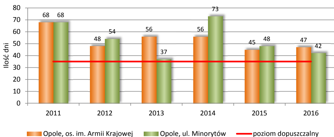
Rysunek 19. Ilość dni z przekroczeniem dopuszczalnego poziomu 24-godzinnego pyłu zawieszonego PM10 w strefie miasto Opole (źródło: opracowanie własne na podstawie danych WIOŚ).
