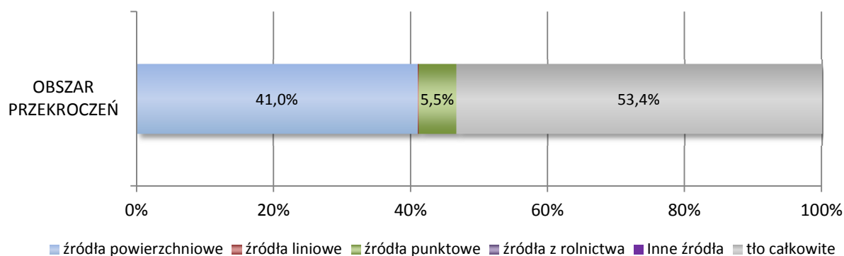
Rysunek 29. Średnie stężenia roczne w podziale na rodzaje źródeł emisji obliczone w na obszarze całej strefy miasto Opole oraz na obszarze przekroczeń stężeń średniorocznych benzo(a)pirenu w roku bazowym 2016 (źródło: na podstawie wyników modelowania matematycznego modelem CALPUFF).
