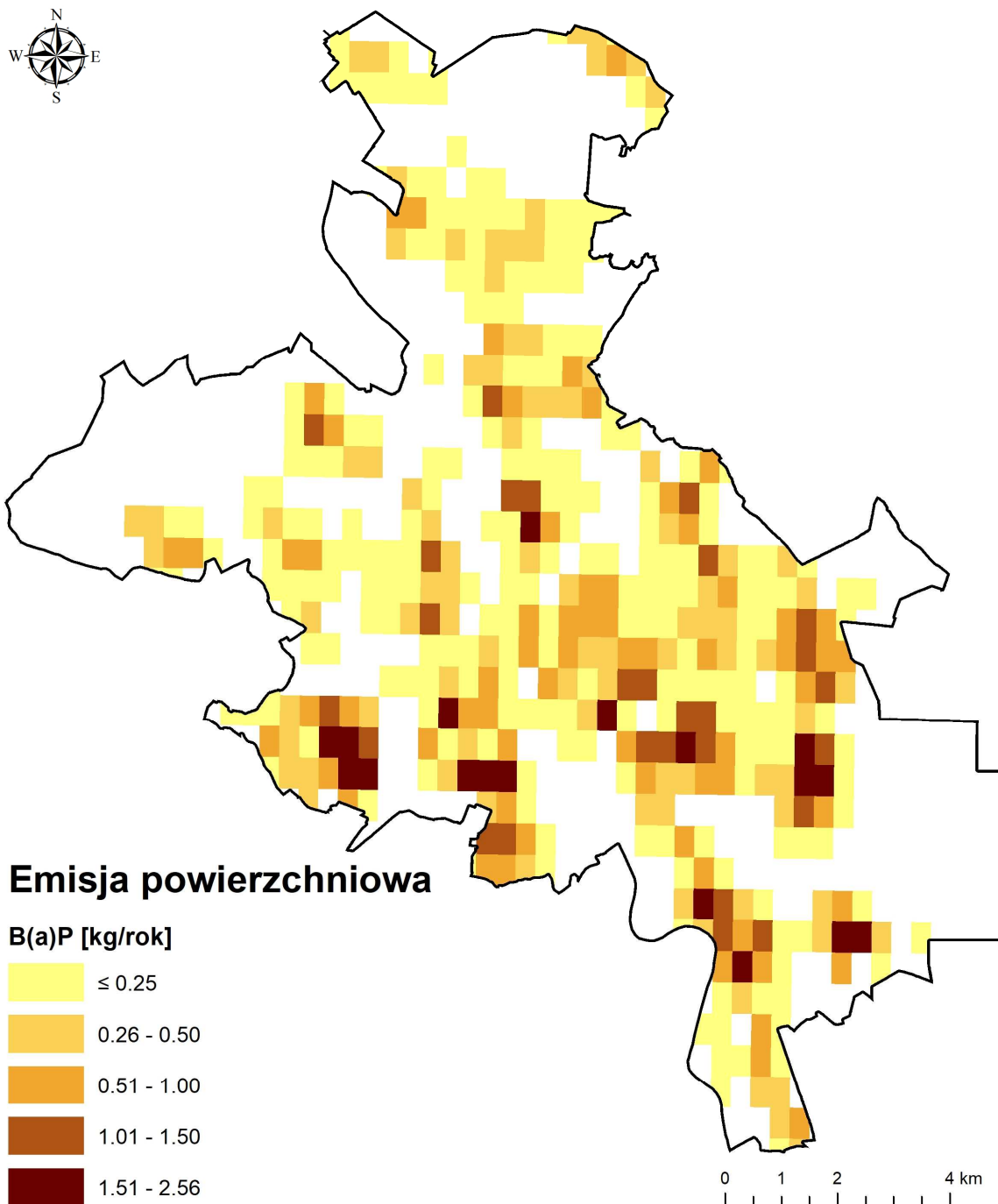
Rysunek 60. Rozkład emisji powierzchniowej benzo(a)pirenu w roku 2016 na terenie strefy miasto Opole (źródło: opracowanie własne).
