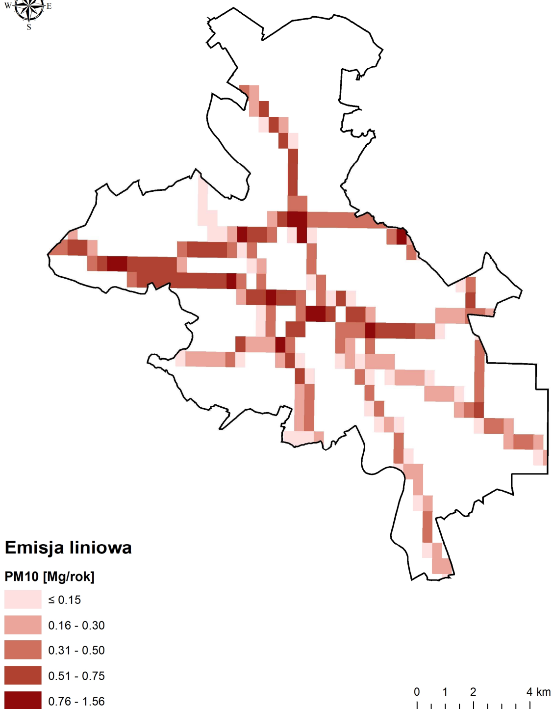
Rysunek 65. Rozkład emisji liniowej pyłu zawieszanego PM10 z dróg krajowych i wojewódzkich w roku 2016 na terenie miasta Opola (źródło: opracowanie własne).
