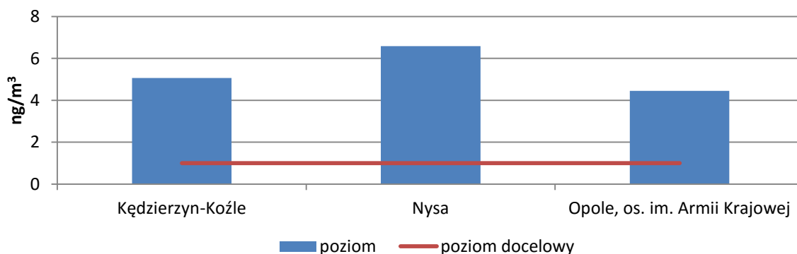
Rysunek 4 Wyniki pomiarów dla średniego rocznego stężenia benzo(a)pirenu, w 2014 r. 48
