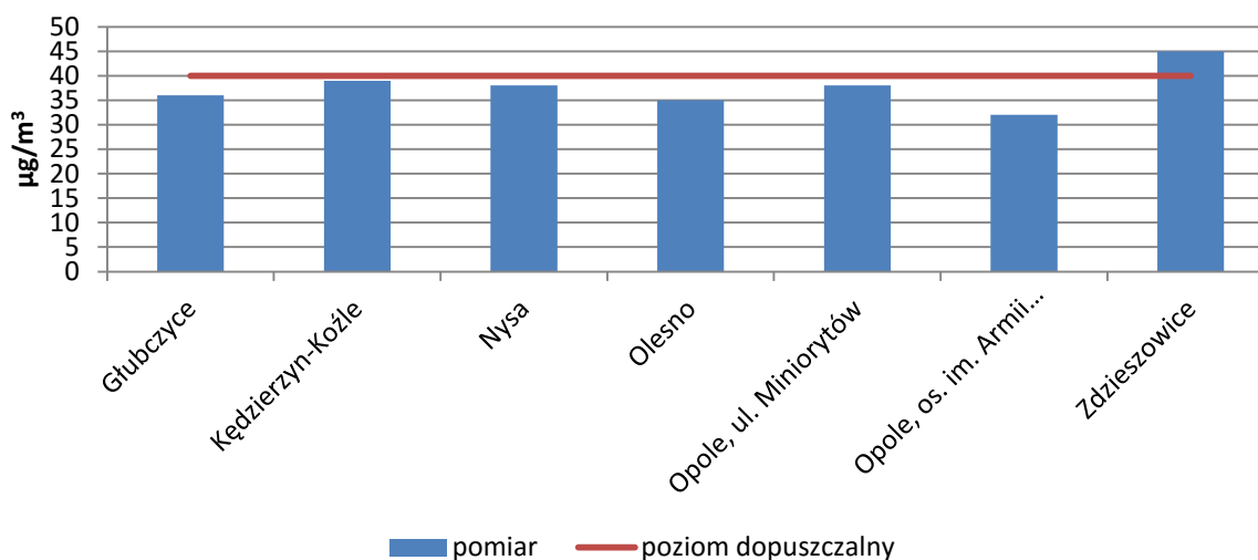
Rysunek 2 Wyniki pomiarów dla średniego rocznego stężenia pyłu zawieszonego PM 10 w 2014 r. 46
