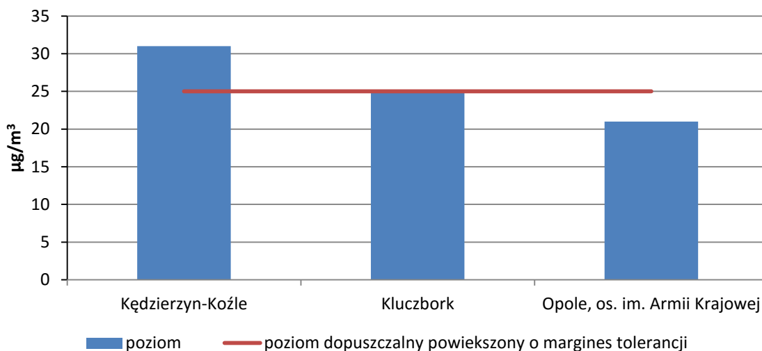
Rysunek 3 Wyniki pomiarów dla średniego rocznego stężenia pyłu zawieszonego PM 2,5 w 2014 r. 47
