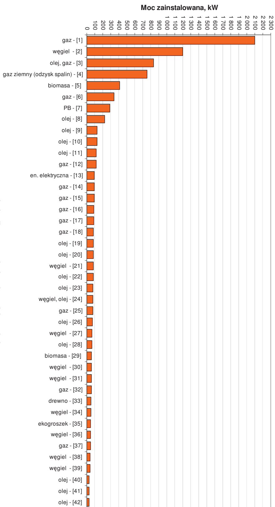
Rys. 12. Kotłownie indywidualne i lokalne na terenie gminy Ozimek.
