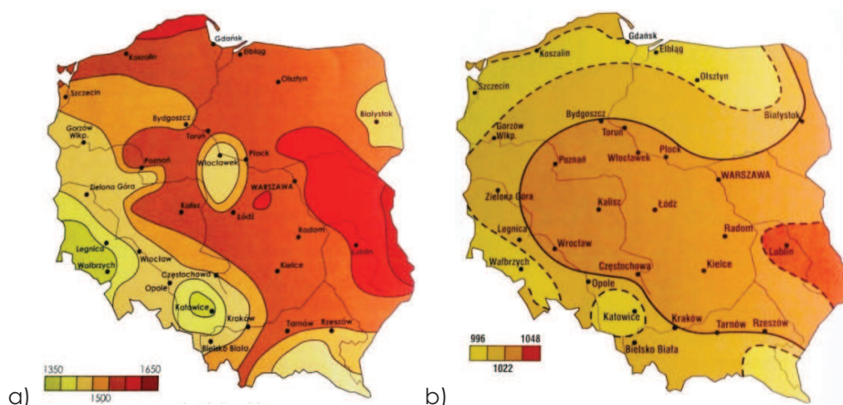
Rysunek 6. Mapy rozkładów a) średniorocznych sum promieniowania całkowitego na powierzchnię poziomą, w kWh/m 2 , b) średniorocznych sum usłonecznienia w h/rok 12
