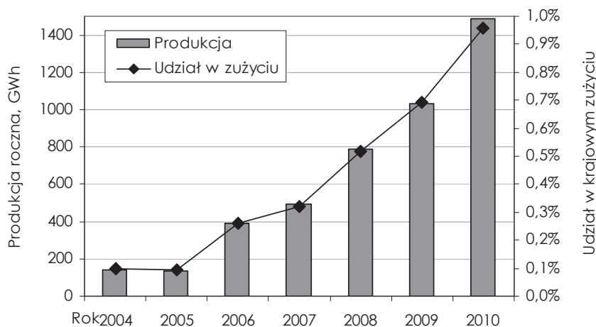
Rys. 5. Produkcja energii elektrycznej przez elektrownie wiatrowe w Polsce
