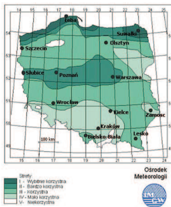
Rys. 3. Mapa stref wietrzności Polski 9
