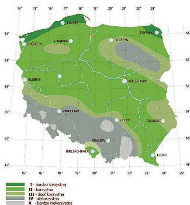
Rys. 2. Mapa stref wietrzności Polski – opracowanie własne w oparciu o mapę sporządzoną przez DELGREEN Sp. z o.o. 8
