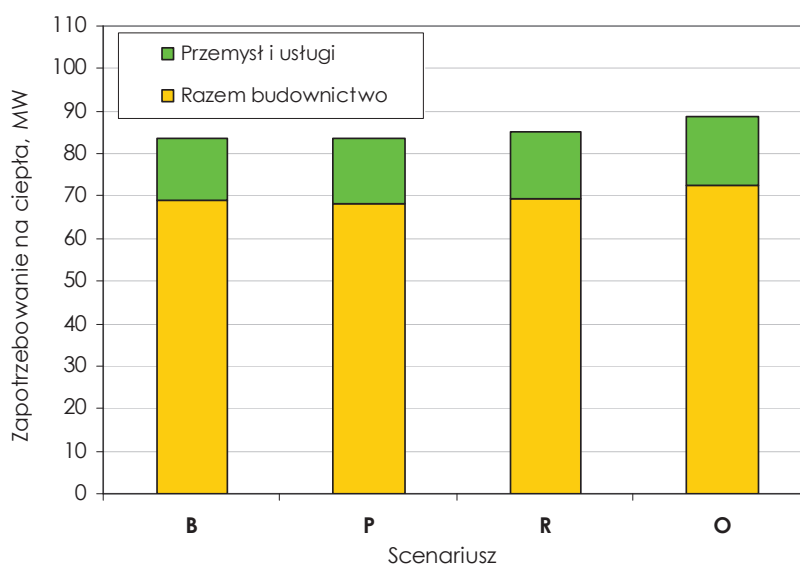
Rys. 13. Obecny i przyszły bilans potrzeb cieplnych gminy. „B” – stan bazowy (obecny), „P” – scenariusz pesymistyczny, „R” – realistyczny, „O” – optymistyczny.
